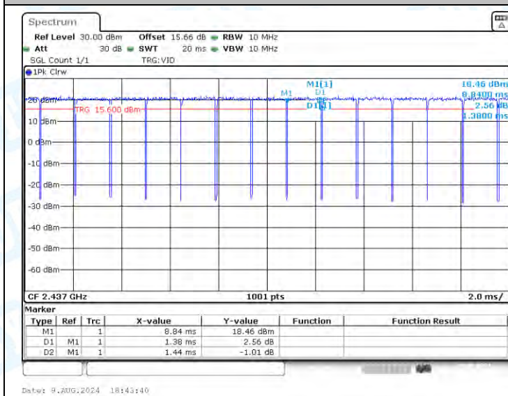
NTNV-11G-Ant1-2437
