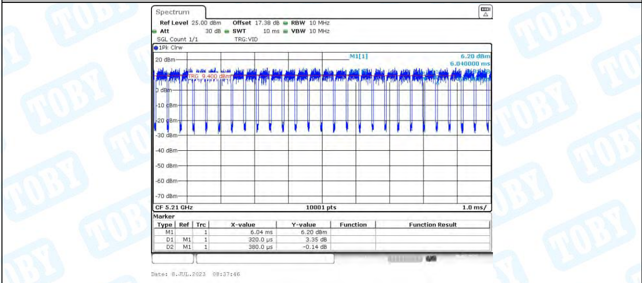
11AC80-CDD_Ant2_5210
