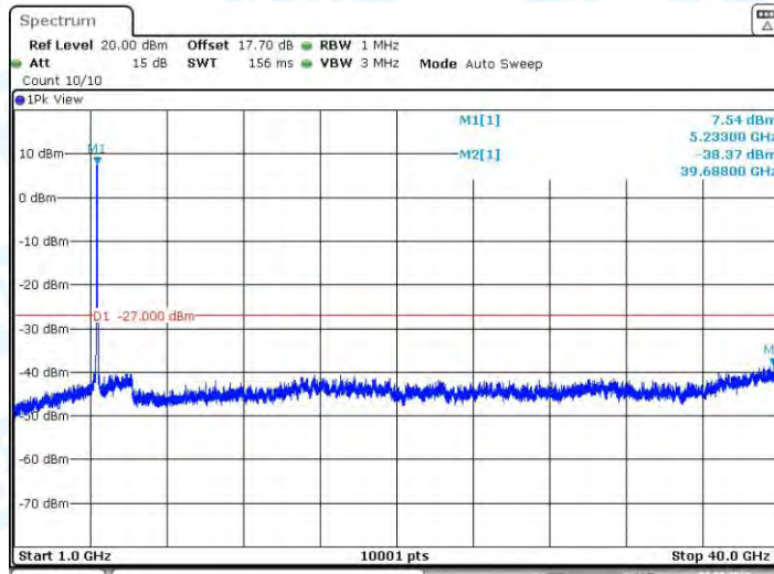
11N40-CDD_Ant1_5230_1000~40000
