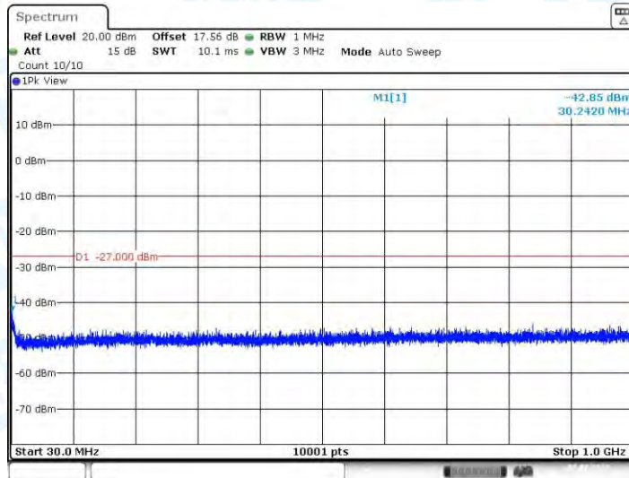
11N40-CDD_Ant2_5550_30~1000
