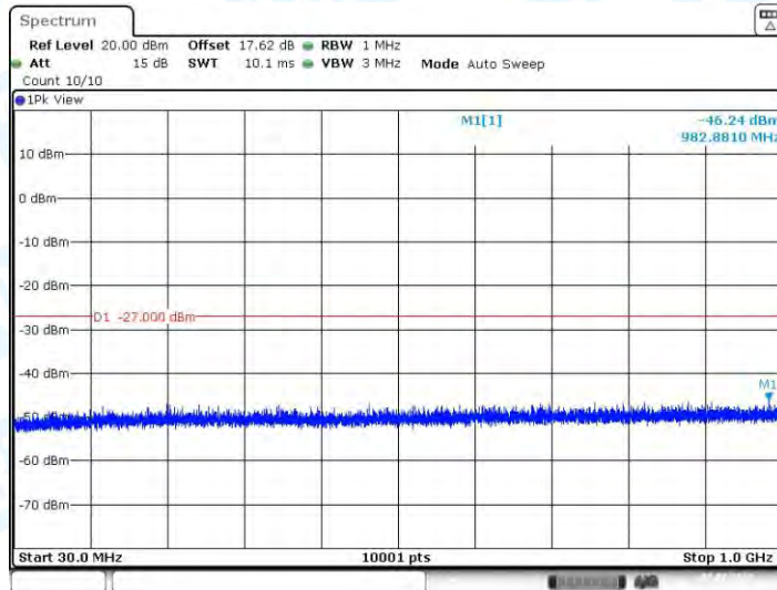
11N20-CDD_Ant1_5580_30~1000
