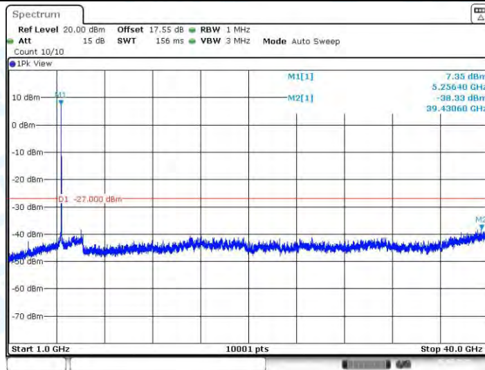
11N20-CDD_Ant1_5260_1000~40000
