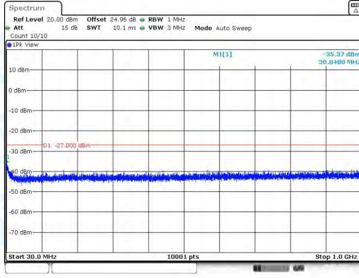
11N40-CDD_Ant2_5755_30~1000
