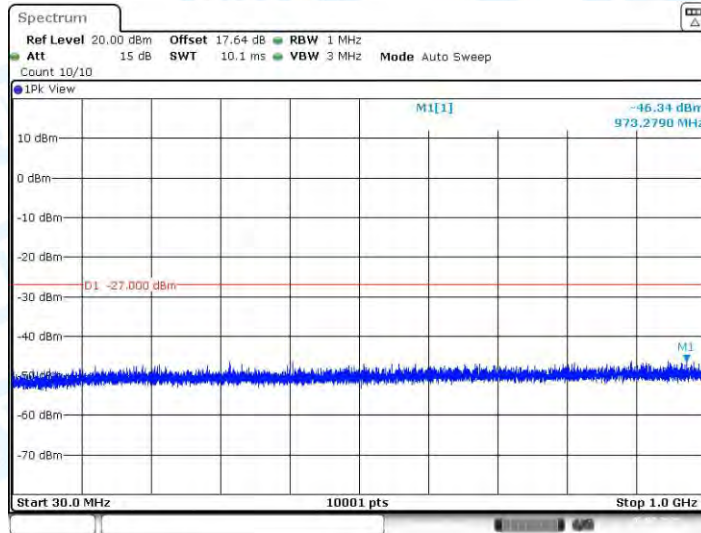
11N20-CDD_Ant2_5580_30~1000
