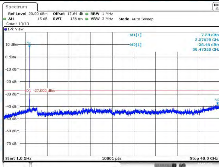
11N20-CDD_Ant2_5580_1000~40000
