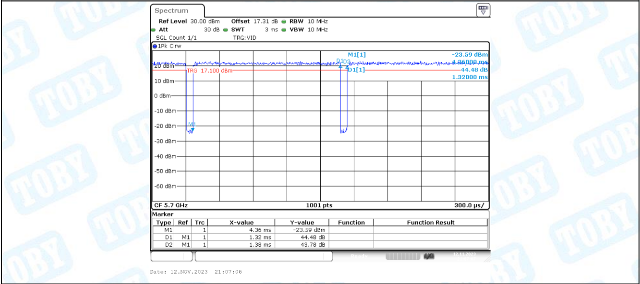
11AC20MIMO_Ant2_5700
