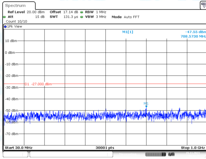
11AC20MIMO_Ant2_5500_30~1000
