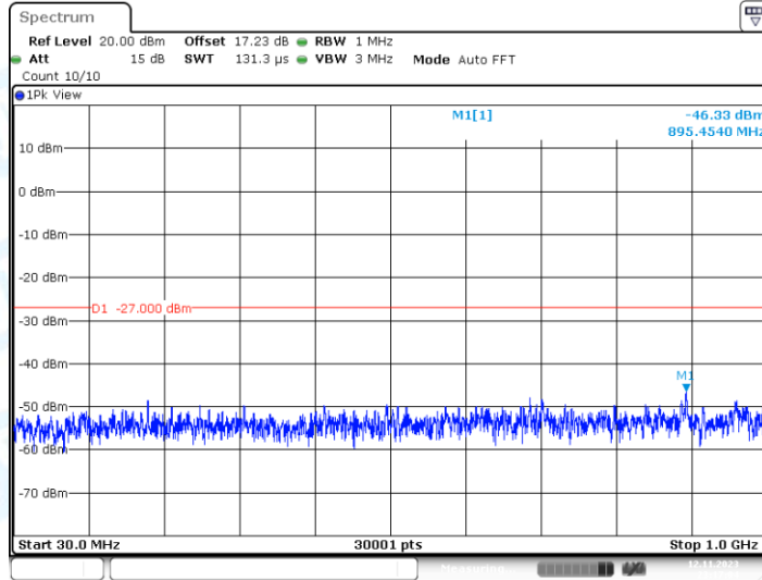
11AC40MIMO_Ant2_5710_30~1000
