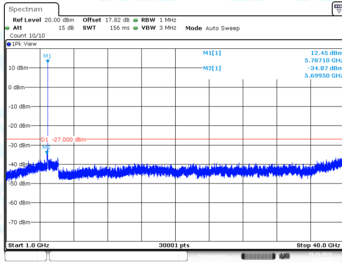
11AC20MIMO_Ant2_5785_1000~40000
