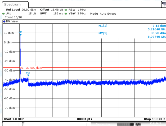
11AC80MIMO_Ant2_5210_1000~40000
