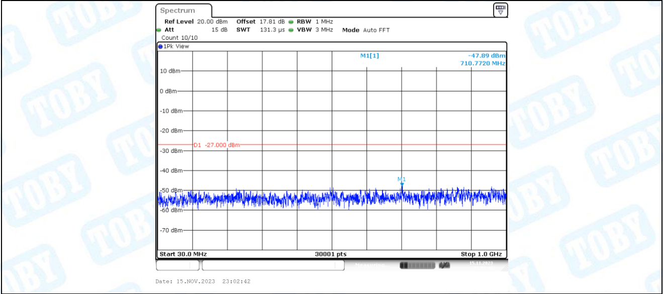
11AC40MIMO_Ant1_5795_1000~40000
