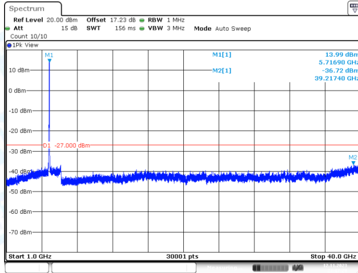
11AC40MIMO_Ant2_5710_1000~40000
