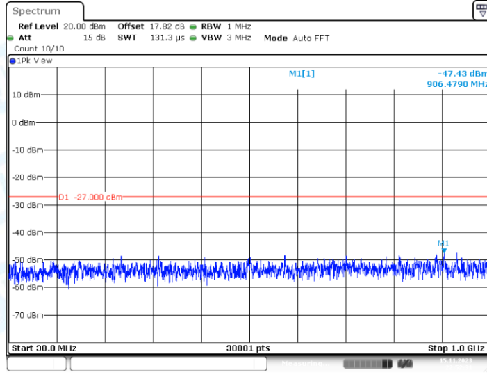
11AC20MIMO_Ant2_5785_30~1000
