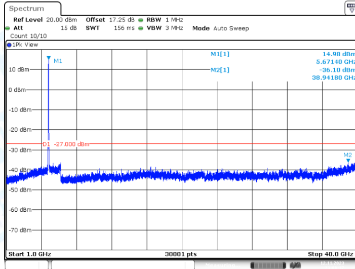
11AC40MIMO_Ant1_5670_1000~40000
