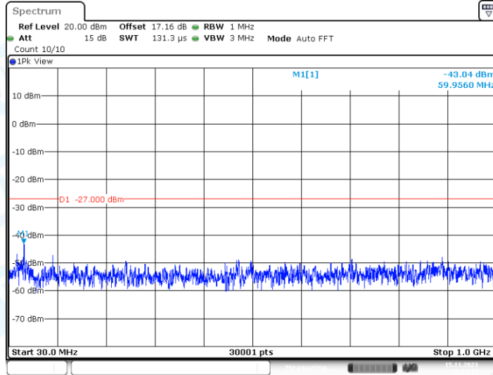
11AC40MIMO_Ant2_5510_30~1000
