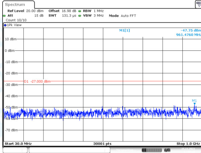
11AC80MIMO_Ant2_5210_30~1000
