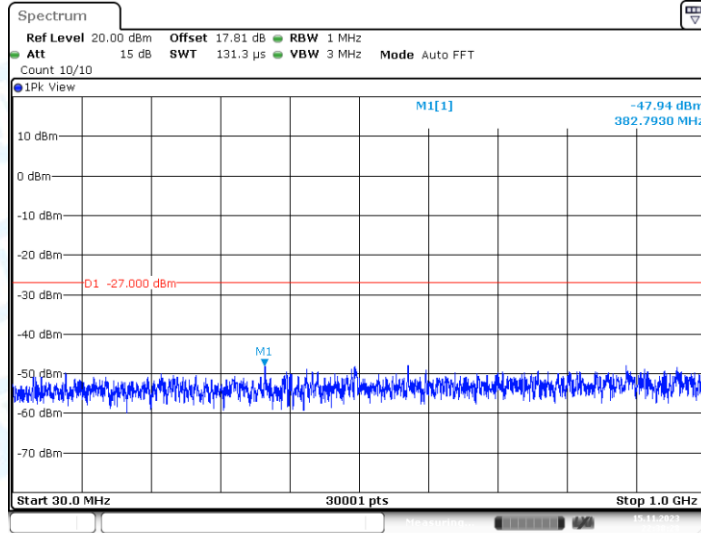
11N40MIMO_Ant1_5755_30~1000
