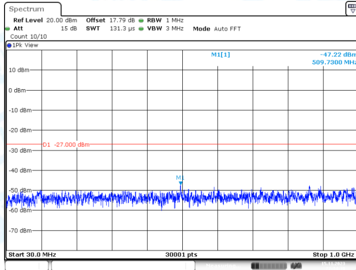
11N20MIMO_Ant1_5825_30~1000
