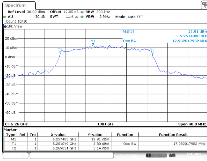
11AC20MIMO_Ant2_5260
