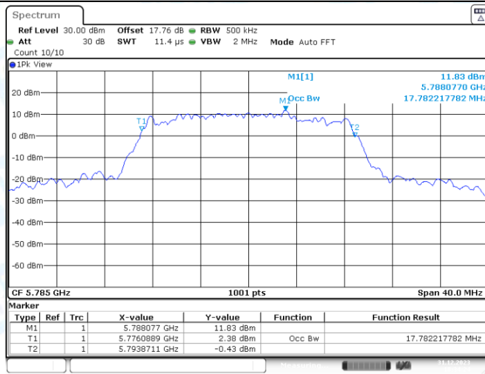
11AC20MIMO_Ant2_5785
