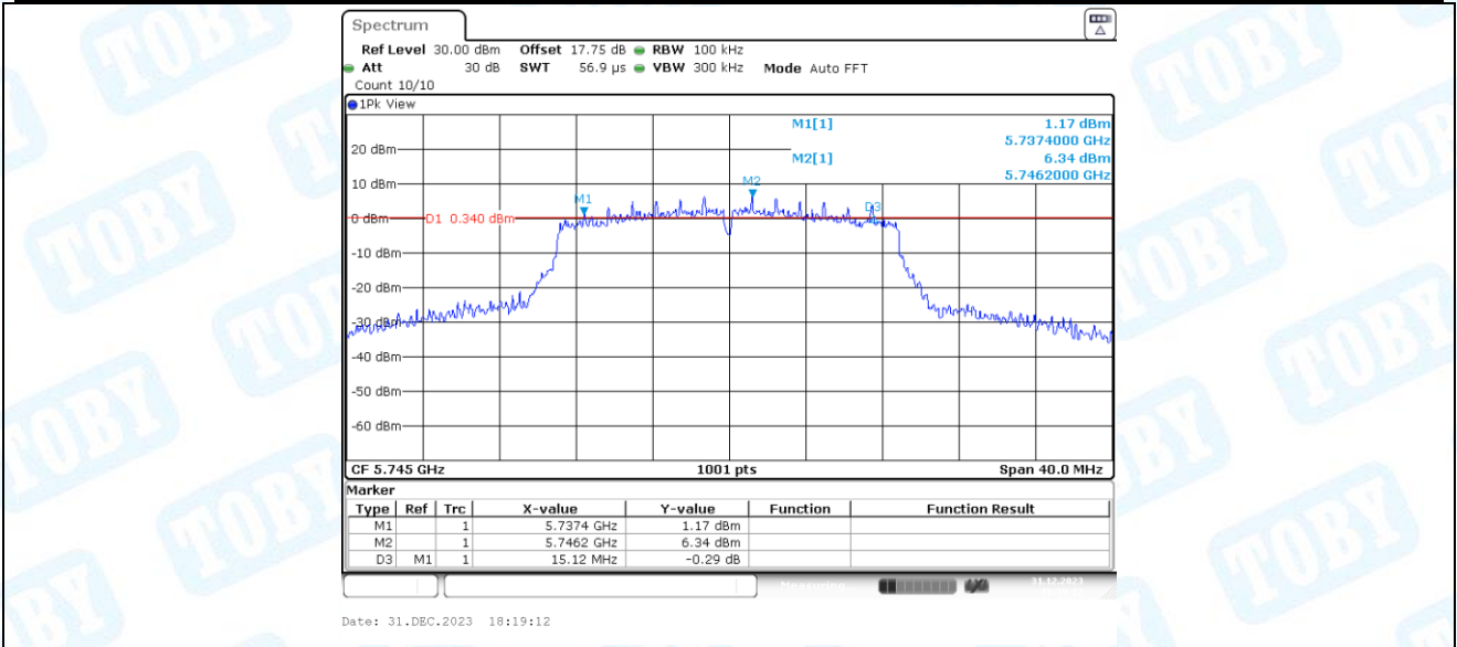
11N20MIMO_Ant2_5745
