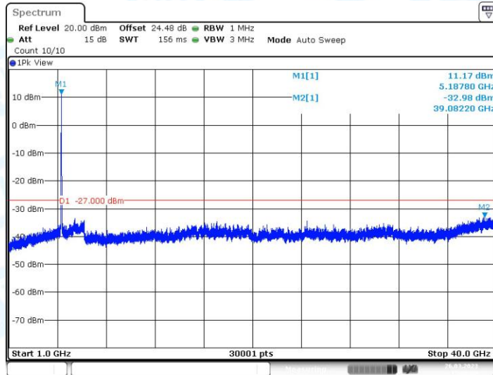
11AC40MIMO_Ant1_5190_1000~40000
