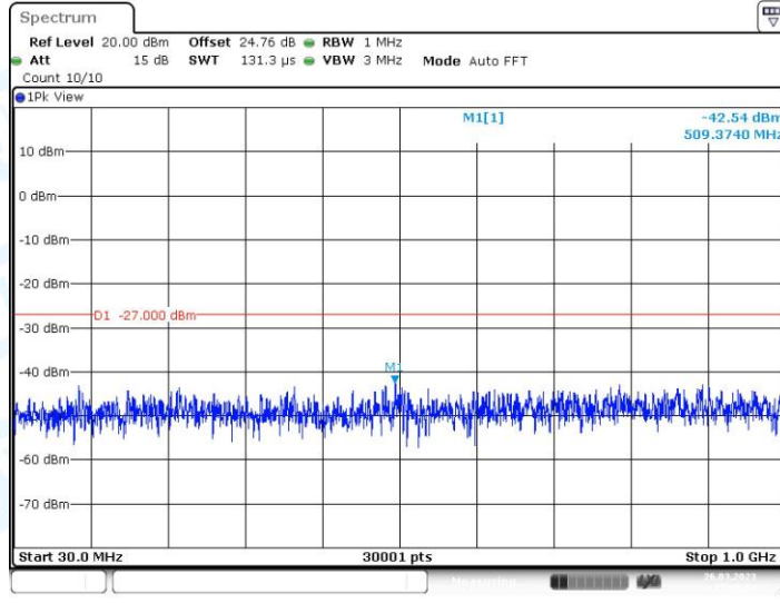
11AC40MIMO_Ant2_5270_30~1000
