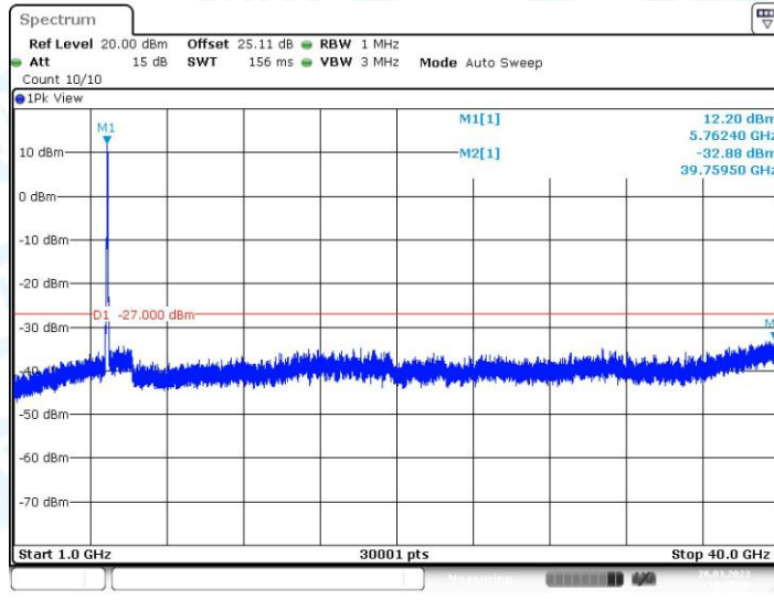
11N40MIMO_Ant2_5755_1000~40000
