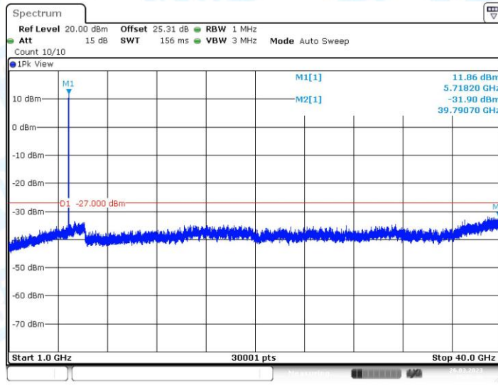
11AC20MIMO_Ant2_5720_1000~40000
