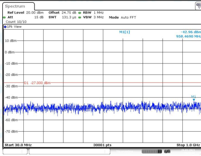
11AC40MIMO_Ant2_5310_30~1000
