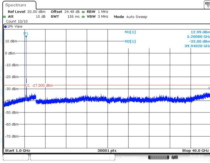
11AC20MIMO_Ant1_5200_1000~40000
