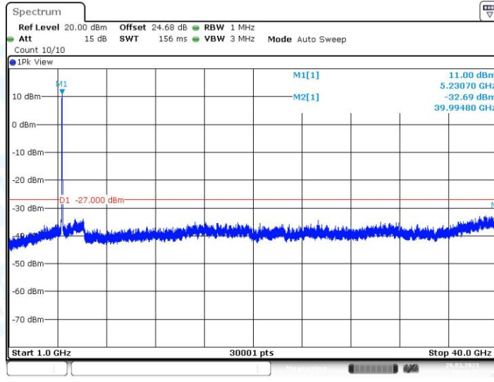
11AC40MIMO_Ant1_5230_1000~40000
