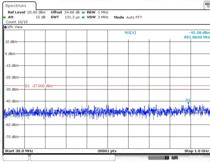
11AC20MIMO_Ant1_5240_30~1000
