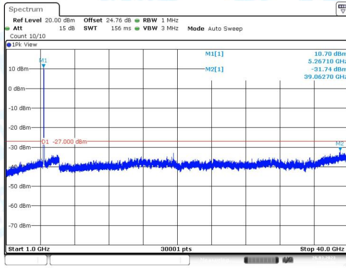
11AC40MIMO_Ant2_5270_1000~40000
