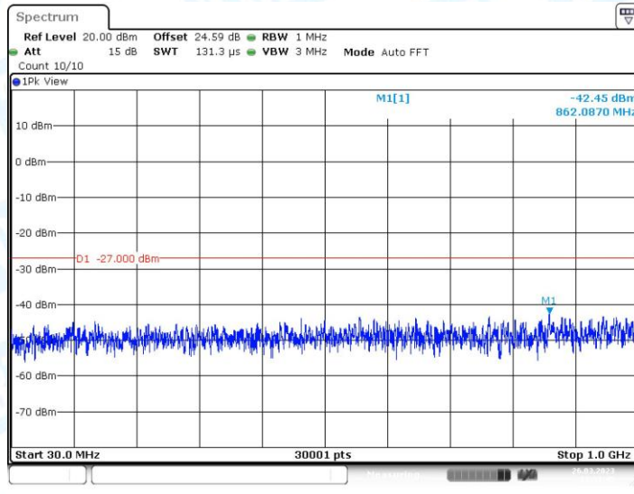
11AC20MIMO_Ant2_5180_30~1000
