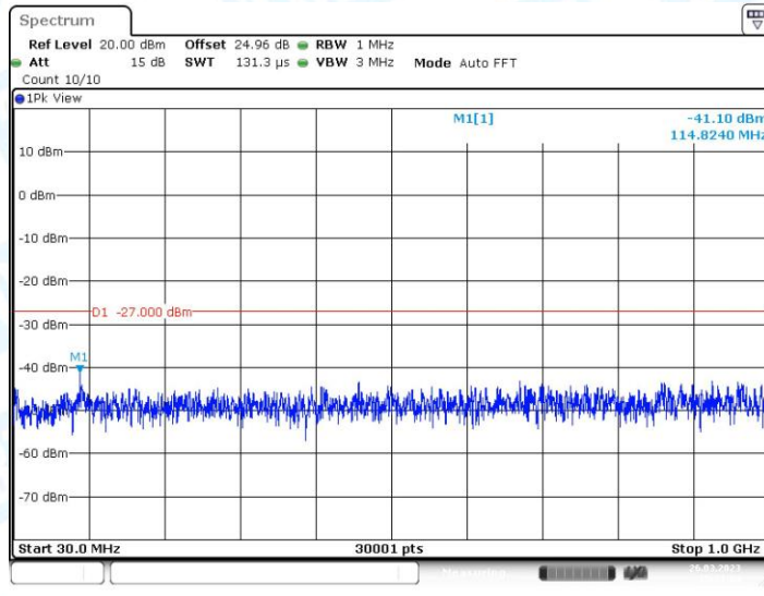
11AC20MIMO_Ant1_5825_30~1000
