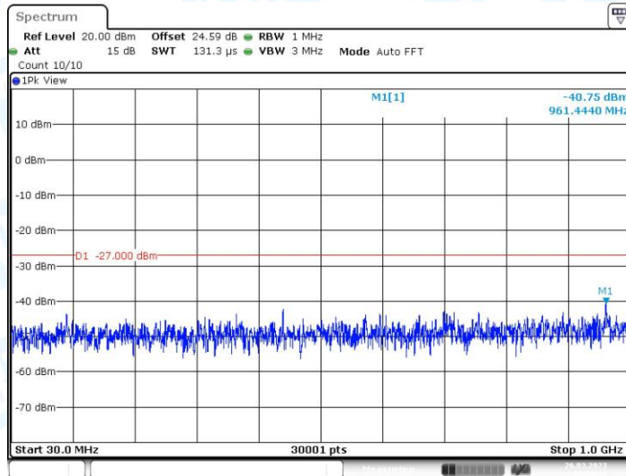
11AC40MIMO_Ant2_5190_30~1000
