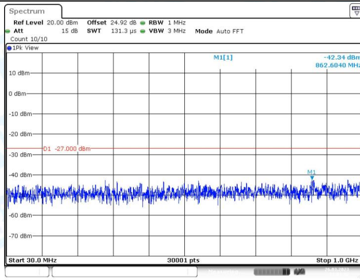
11N40MIMO_Ant1_5795_30~1000
