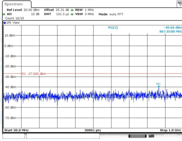
11AC20MIMO_Ant2_5720_30~1000
