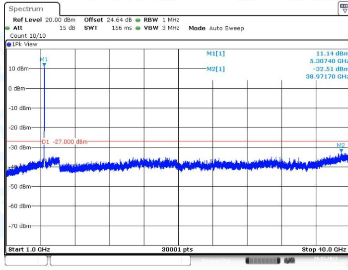
11AC40MIMO_Ant1_5310_1000~40000
