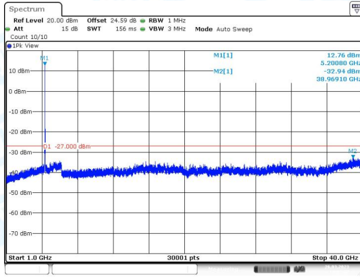
11AC20MIMO_Ant2_5200_1000~40000
