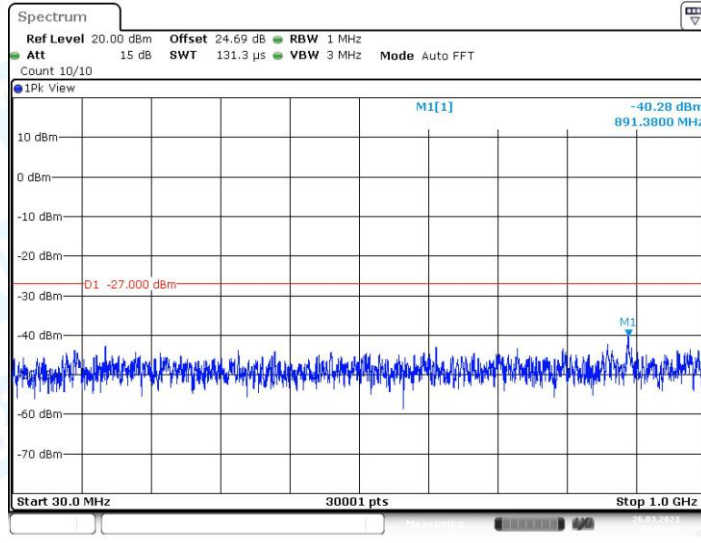
11AC40MIMO_Ant1_5270_30~1000
