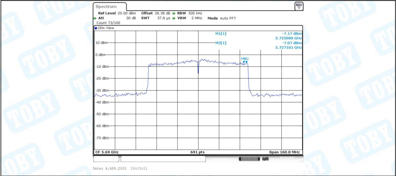
11AC80MIMO_Ant2_5690_UNII-3
