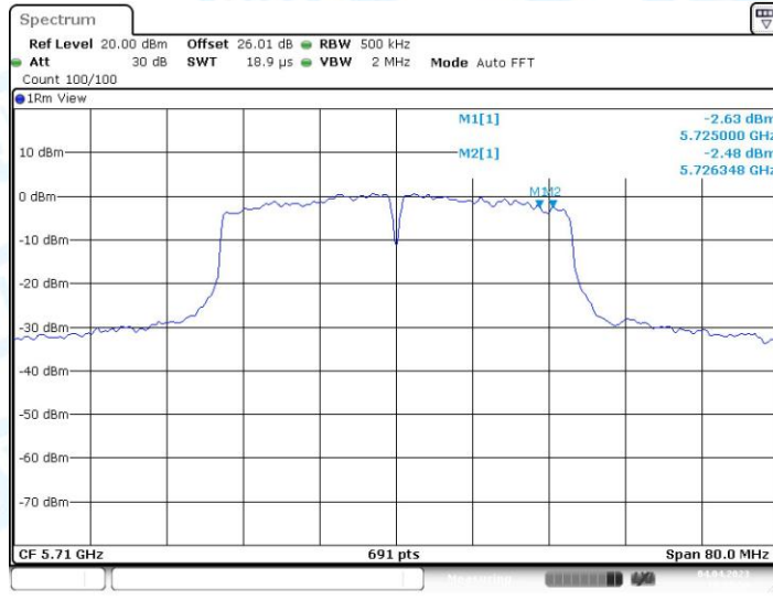
11AC40MIMO_Ant1_5710_UNII-3
