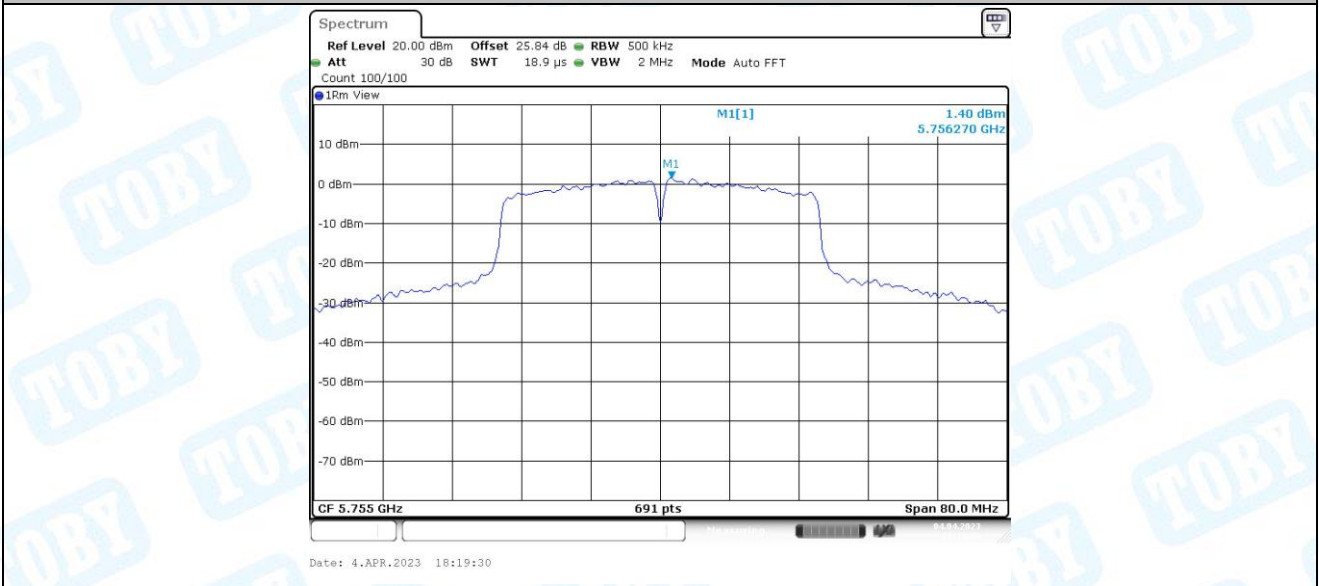
11N40MIMO_Ant2_5755
