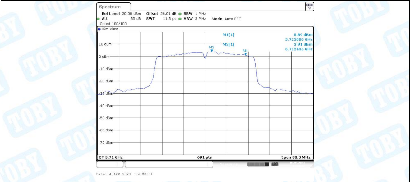
11AC40MIMO_Ant2_5710_UNII-2C
