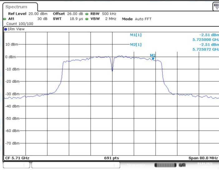
11AC40MIMO_Ant2_5710_UNII-3
