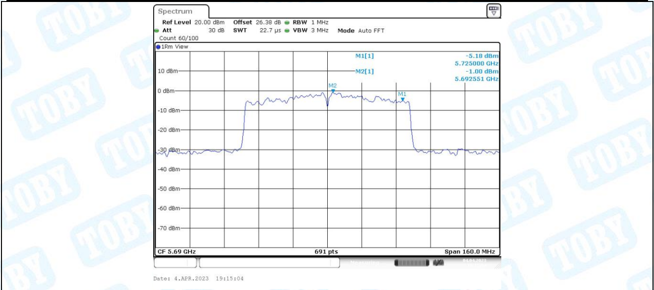
11AC80MIMO_Ant2_5690_UNII-2C
