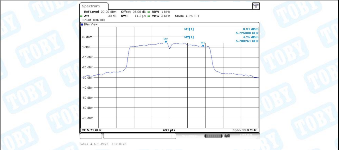
11N40MIMO_Ant1_5710_UNII-3
