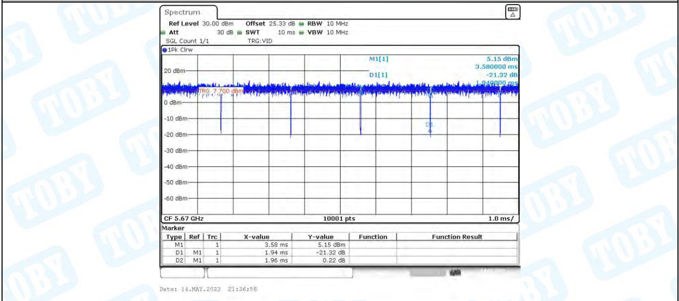
11AX40MIMO_Ant4_5670
