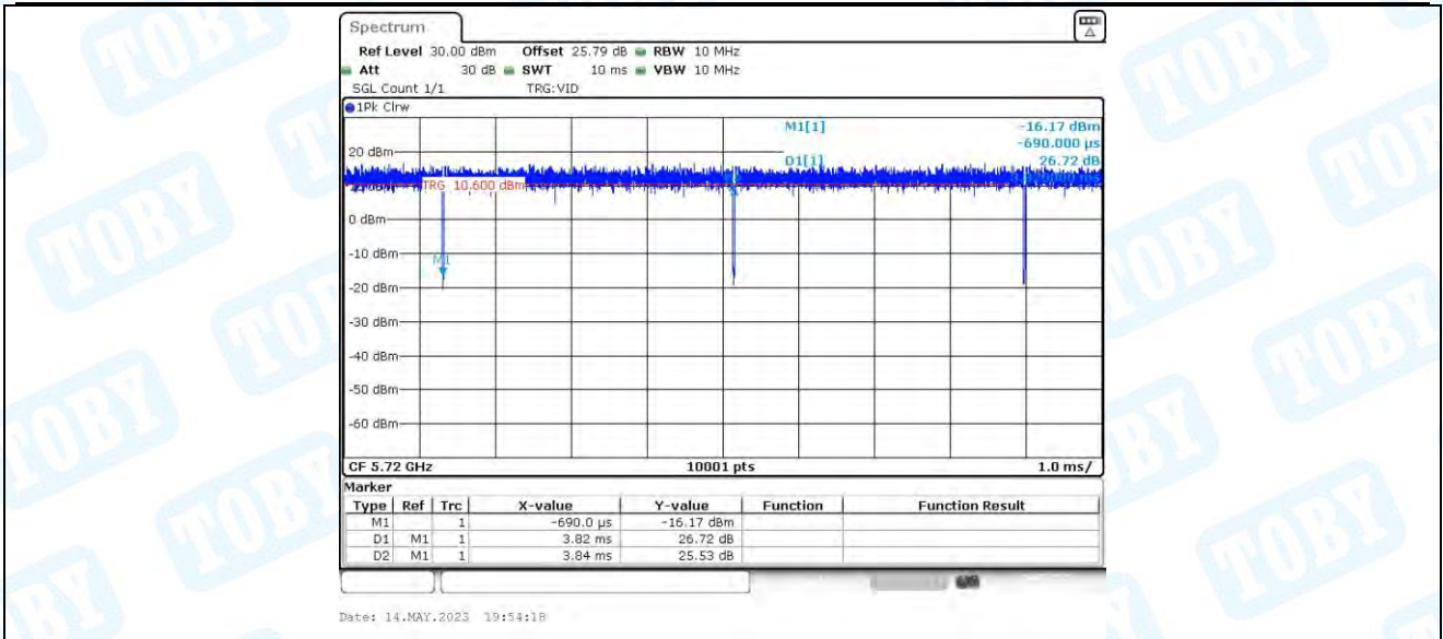
11AX20MIMO_Ant3_5720
