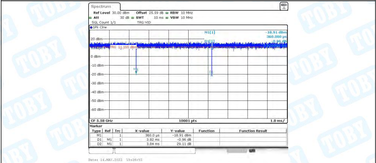
11AX20MIMO_Ant3_5580
