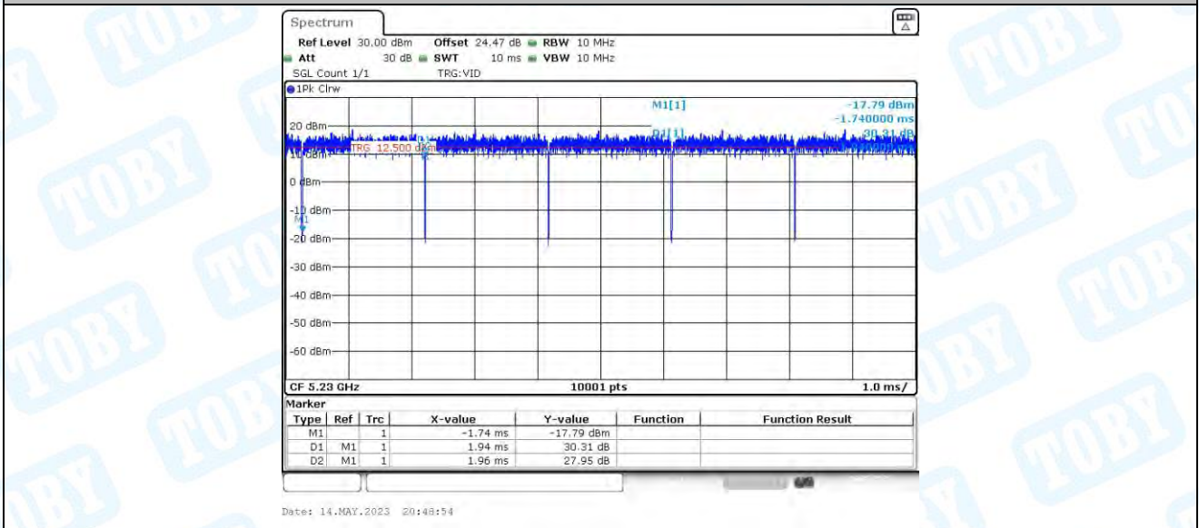
11AX40MIMO_Ant2_5230
