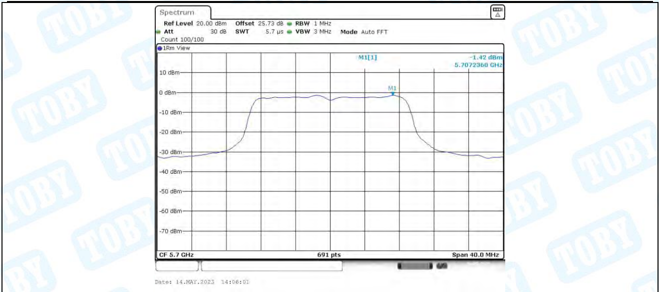
11AC20MIMO_Ant3_5700
