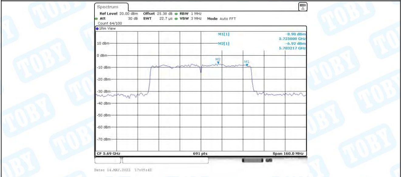
11AC80MIMO_Ant4_5690_UNII-2C
