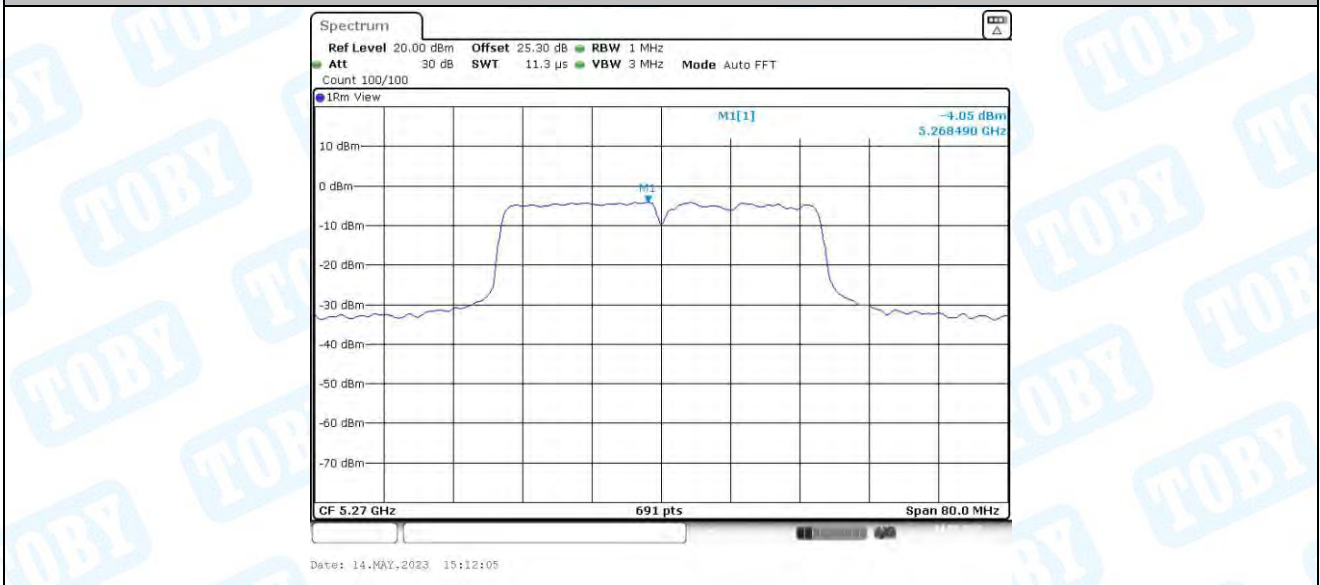
11AC40MIMO_Ant3_5270
