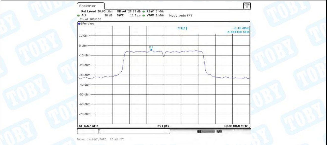
11AC40MIMO_Ant2_5670
