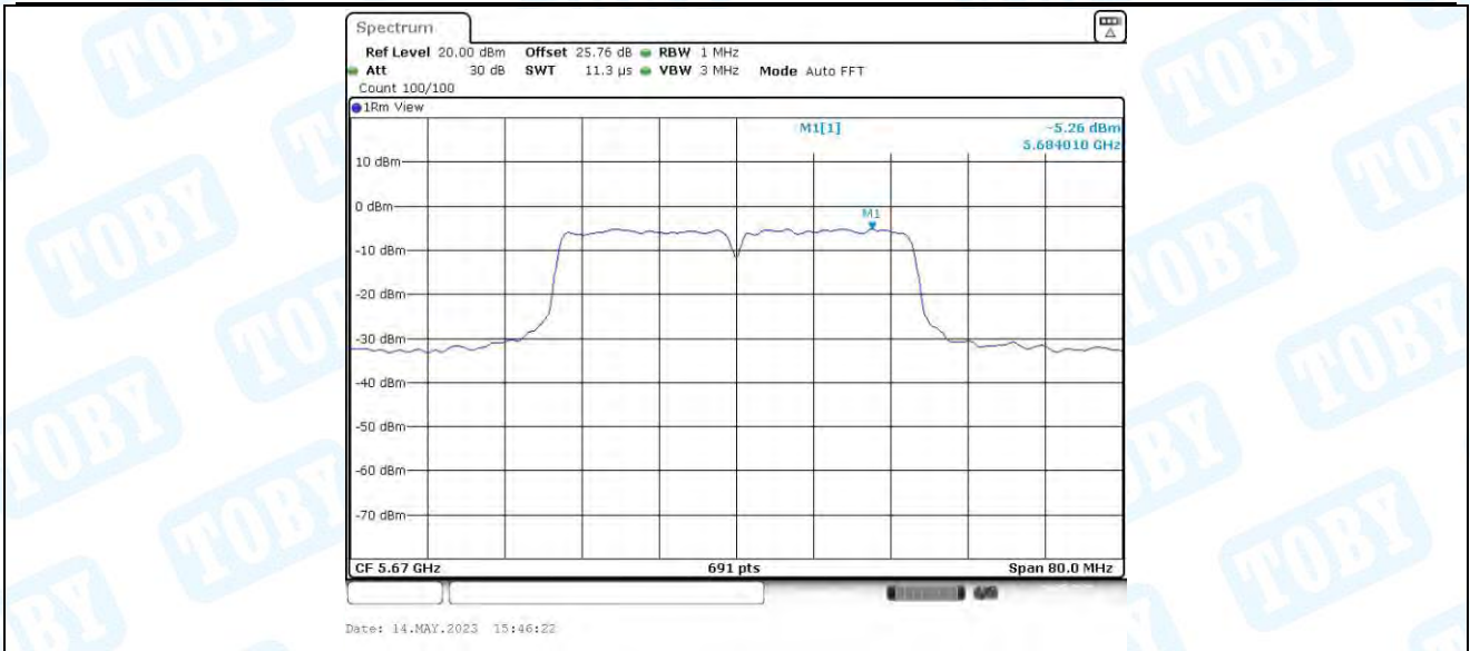
11AC40MIMO_Ant3_5670
