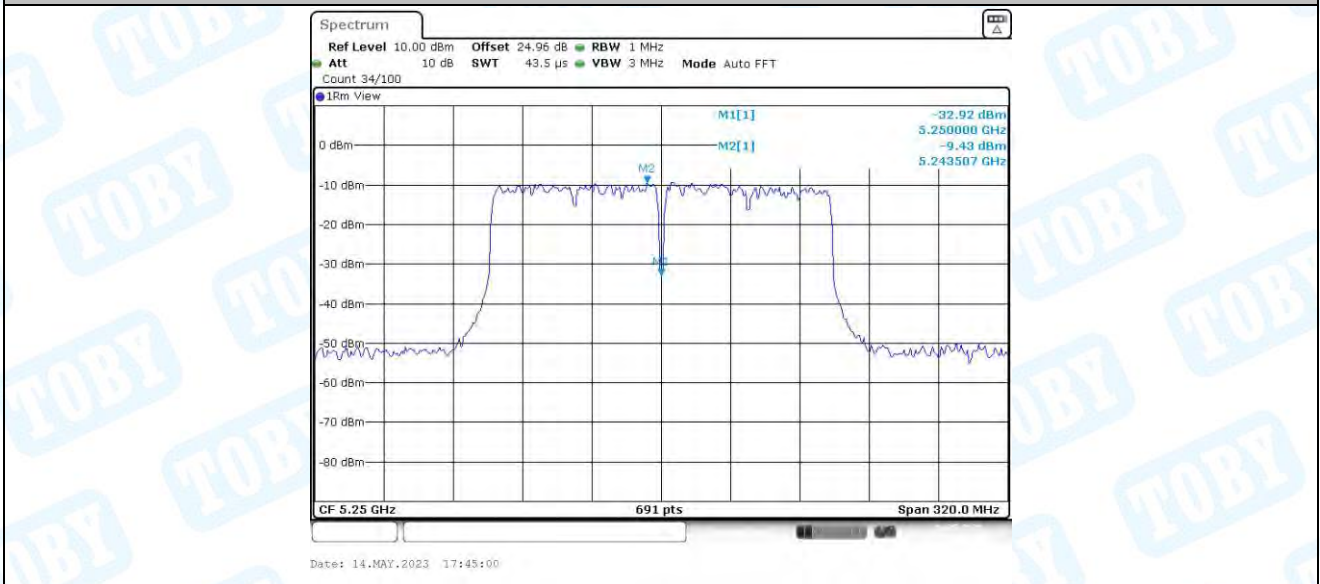
11AC160MIMO_Ant4_5250_UNII-1
