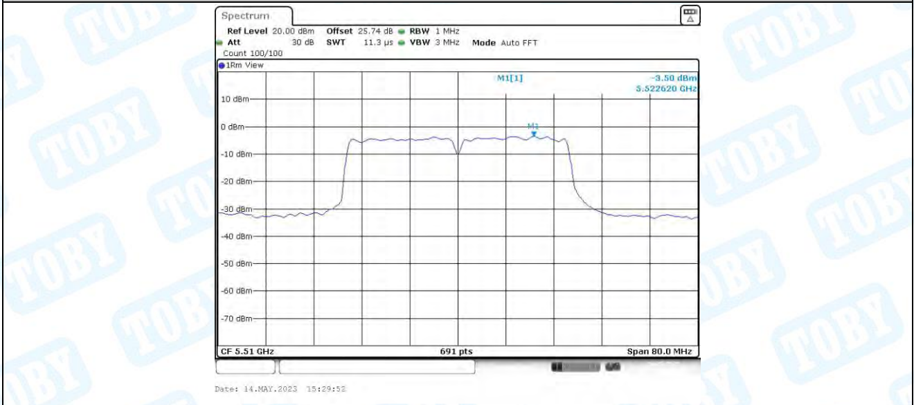
11AC40MIMO_Ant3_5510
