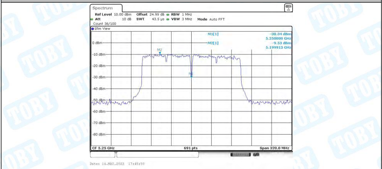
11AC160MIMO_Ant1_5250_UNII-2A
