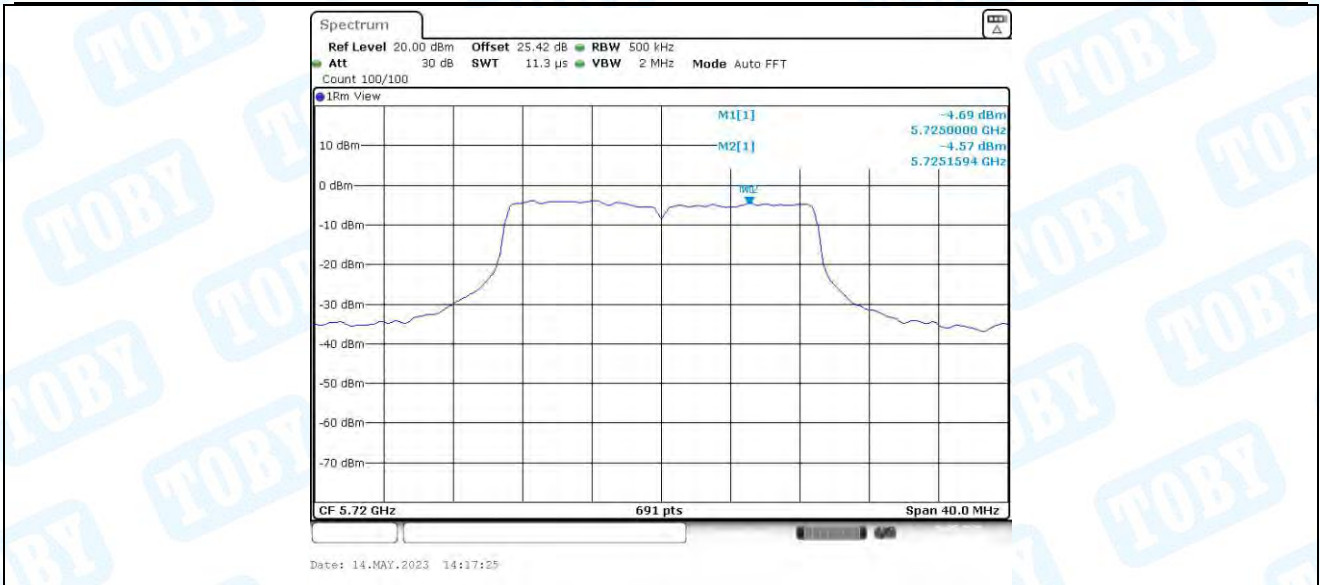
11AC20MIMO_Ant4_5720_UNII-3
