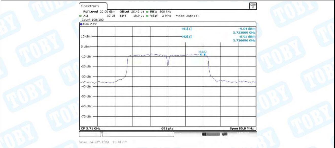
11N40MIMO_Ant4_5710_UNII-3
