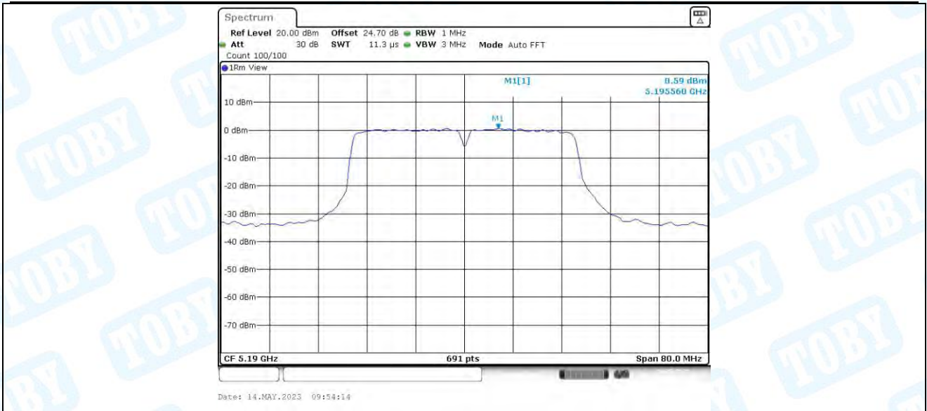
11N40MIMO_Ant4_5190
