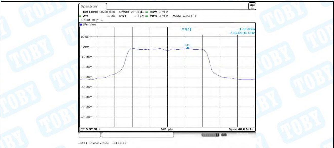
11AC20MIMO_Ant3_5320
