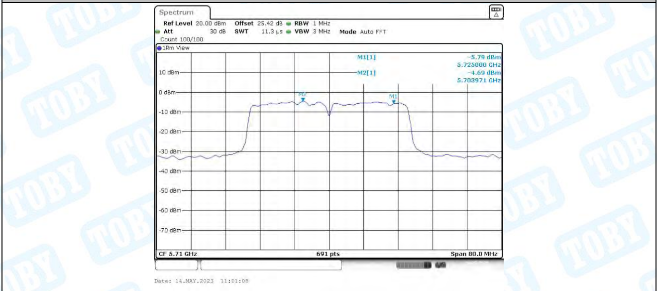
11N40MIMO_Ant4_5710_UNII-2C
