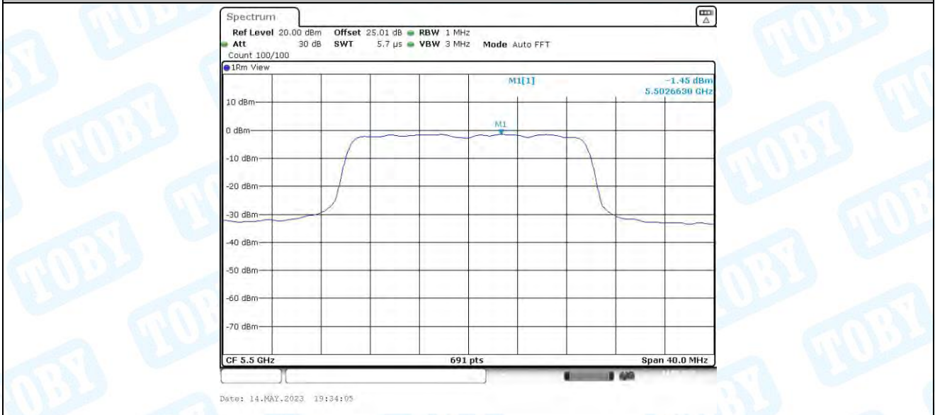
11AX20MIMO_Ant2_5500
