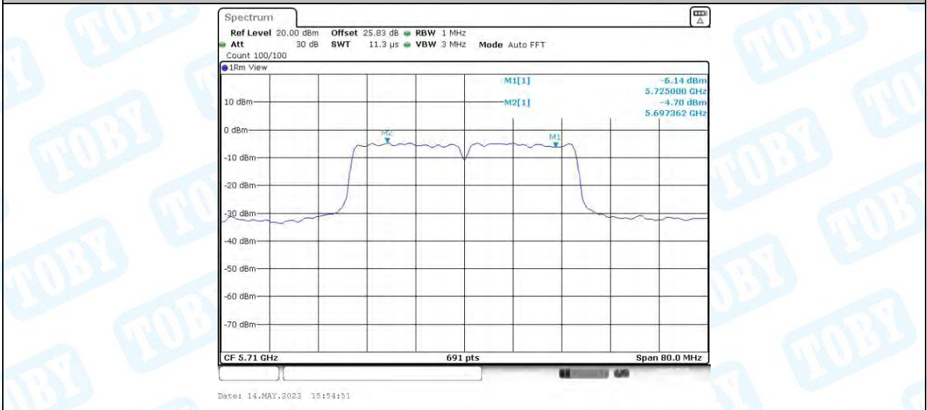
11AC40MIMO_Ant3_5710_UNII-2C
