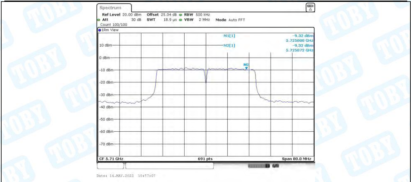
11N40MIMO_Ant2_5710_UNII-3
