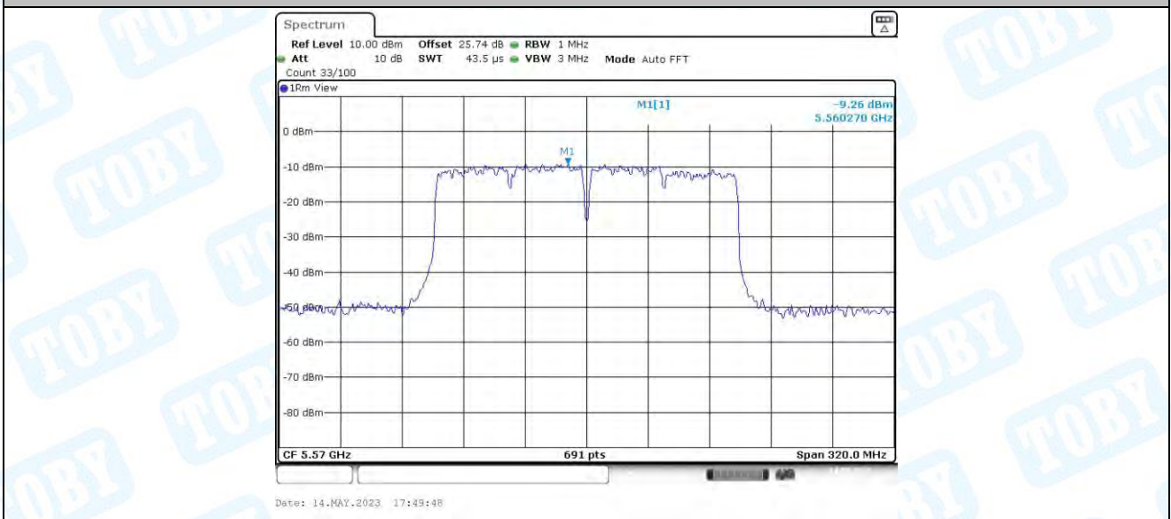
11AC160MIMO_Ant3_5570
