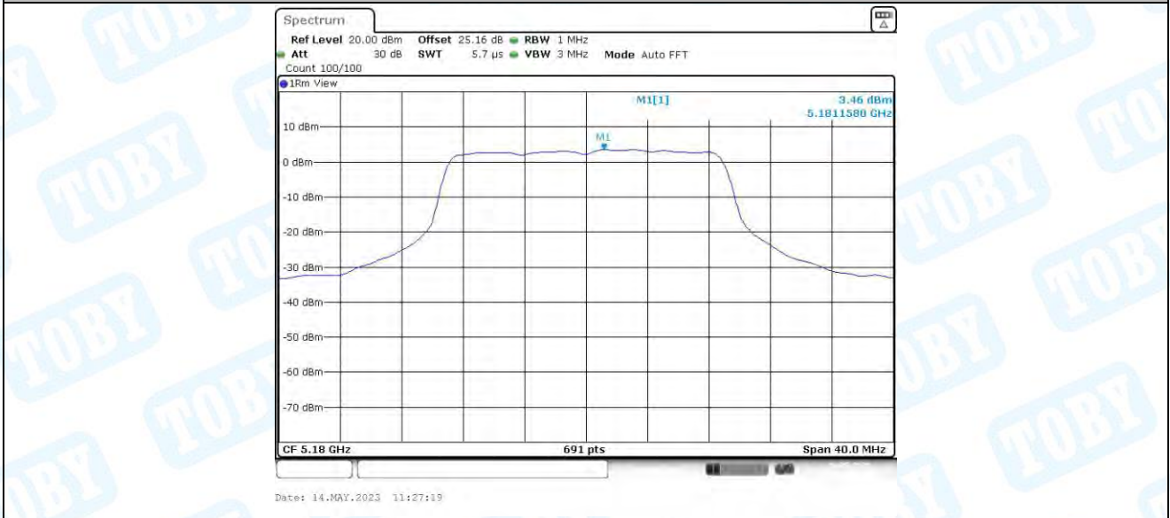
11AC20MIMO_Ant3_5180
