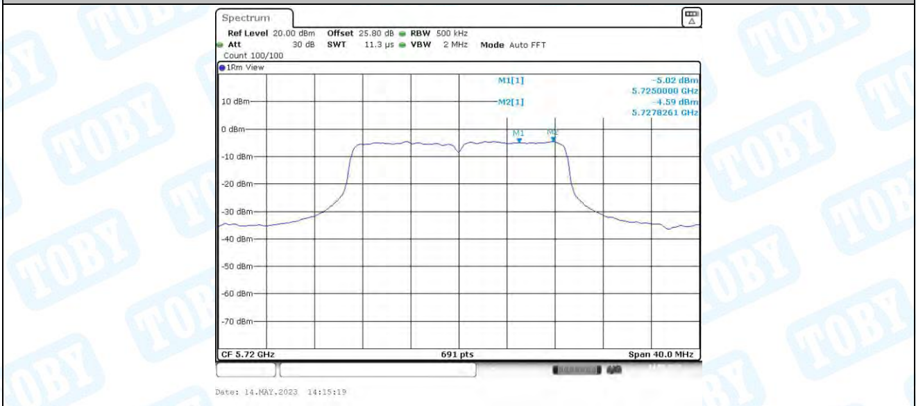
11AC20MIMO_Ant3_5720_UNII-3
