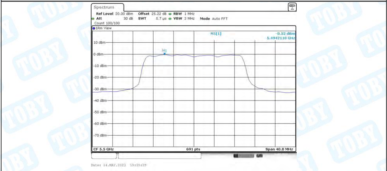
11AX20MIMO_Ant4_5500
