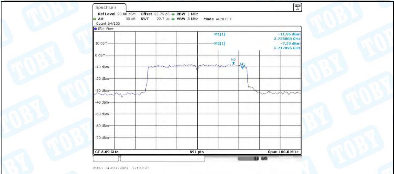
11AC80MIMO_Ant3_5690_UNII-2C
