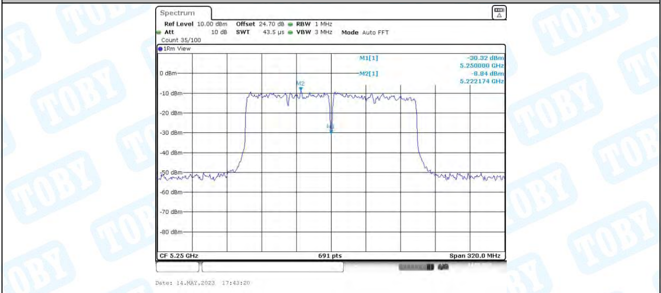
11AC160MIMO_Ant2_5250_UNII-1
