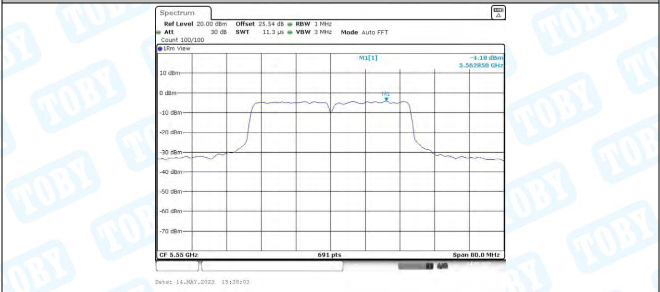
11AC40MIMO_Ant3_5550
