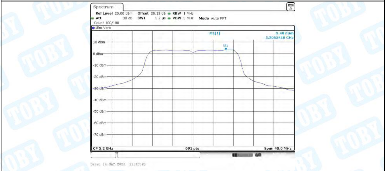
11AC20MIMO_Ant3_5200
