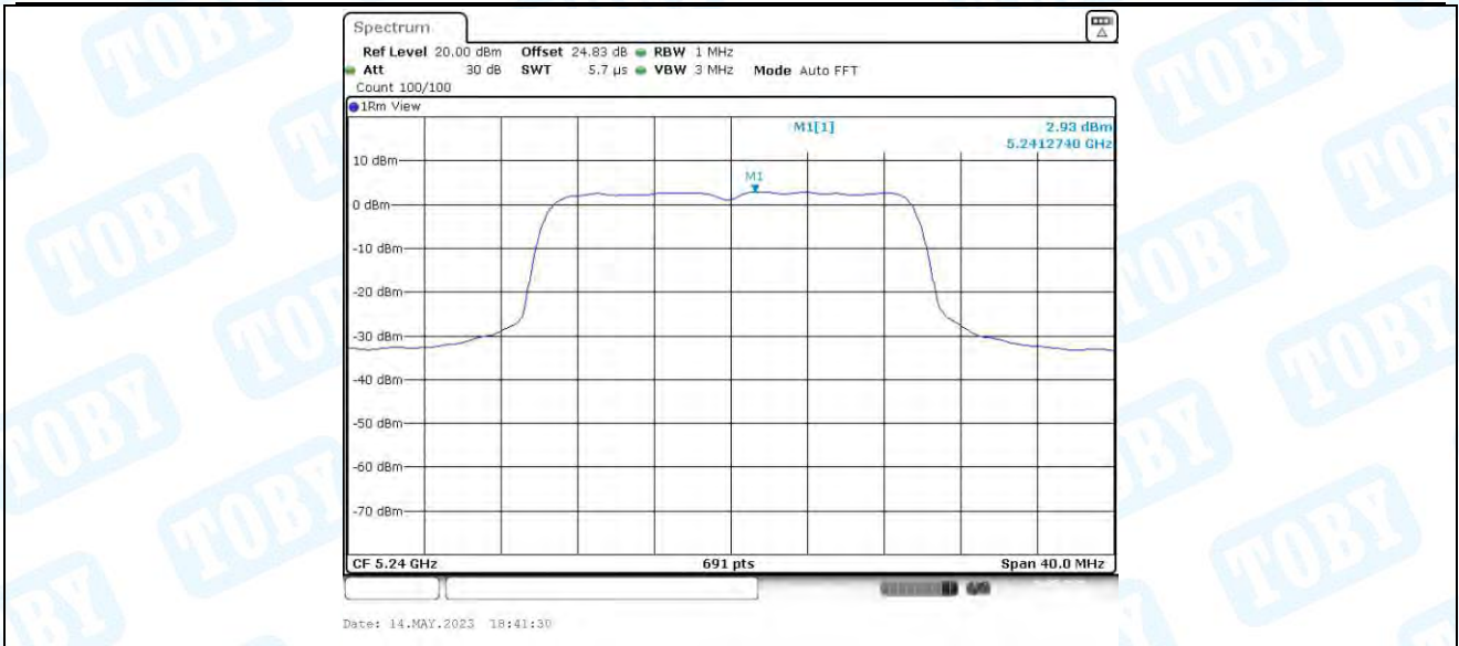
11AX20MIMO_Ant4_5240
