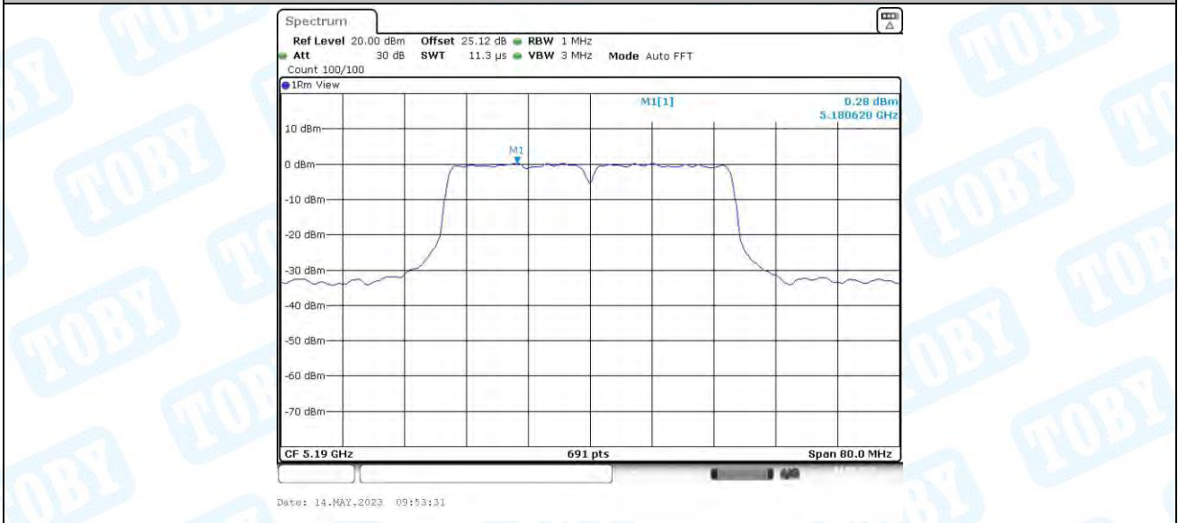
11N40MIMO_Ant3_5190
