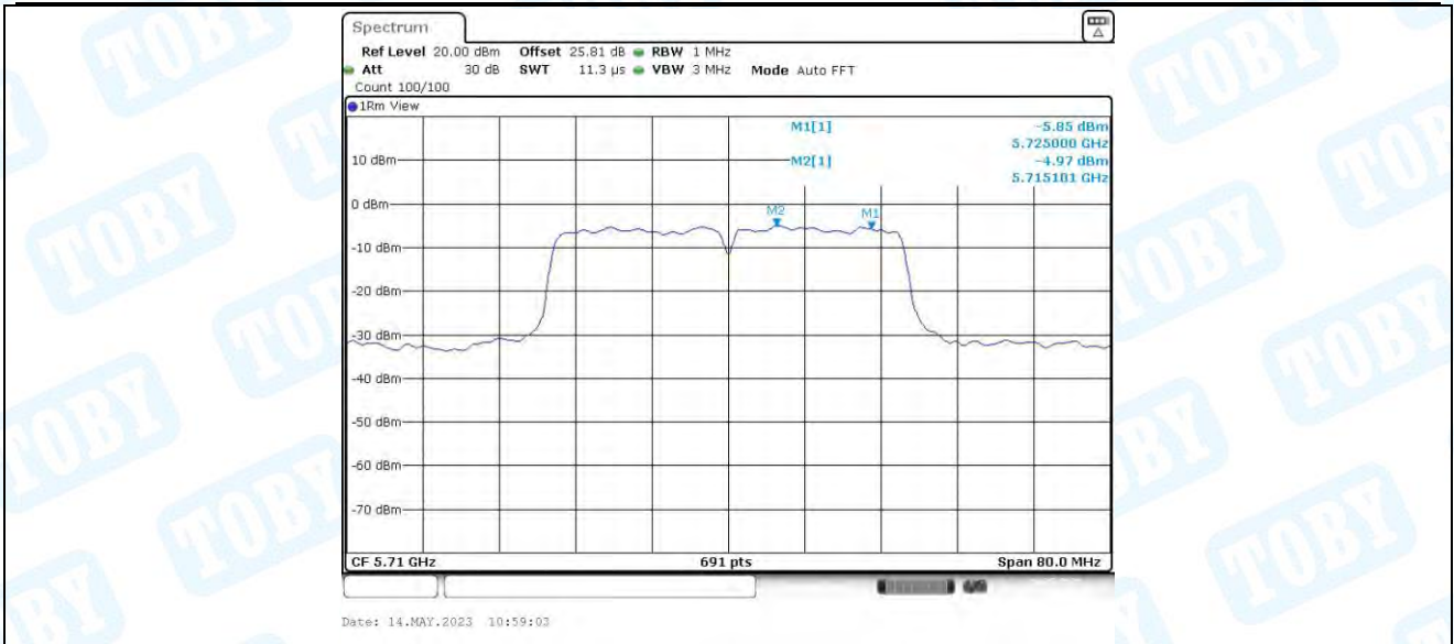
11N40MIMO_Ant3_5710_UNII-2C
