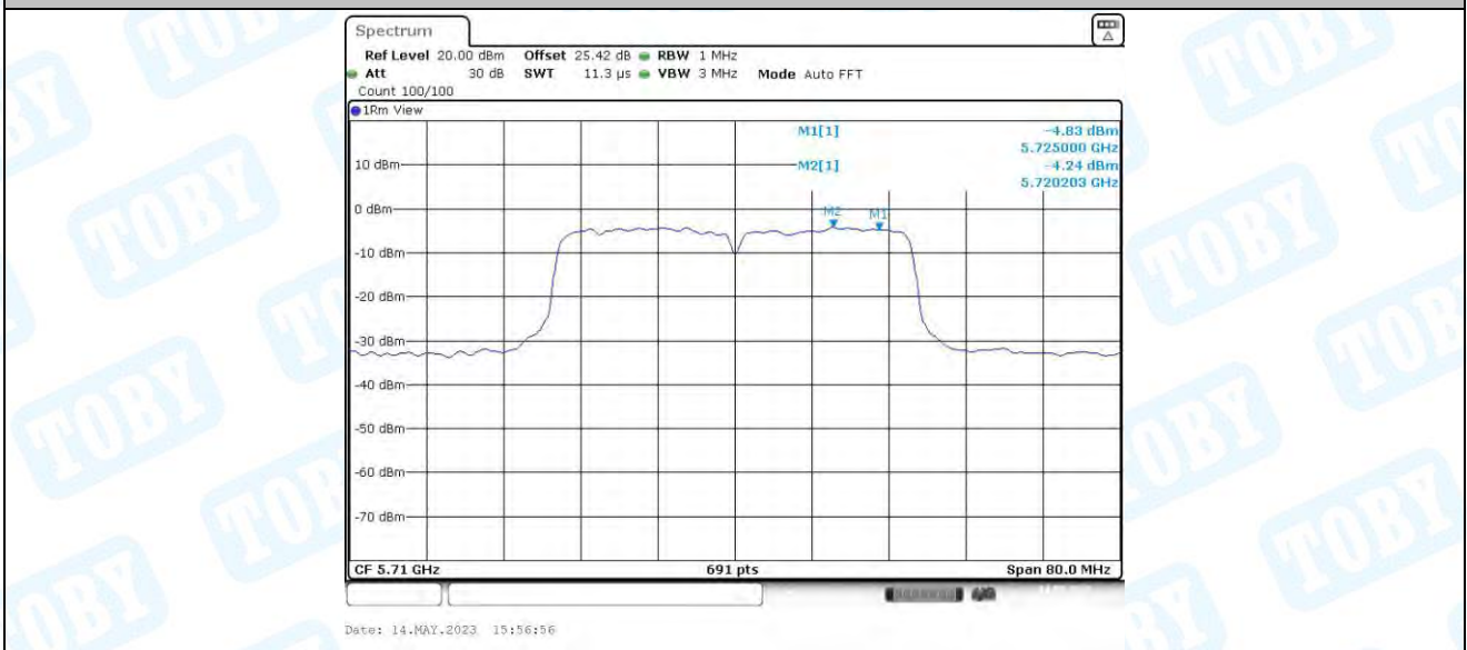
11AC40MIMO_Ant4_5710_UNII-2C
