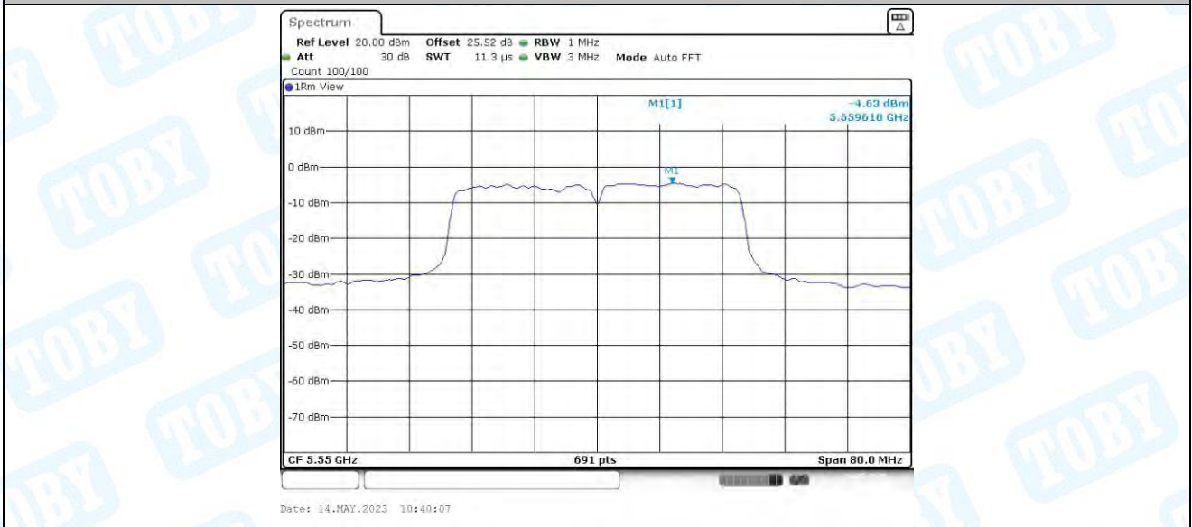
11N40MIMO_Ant3_5550
