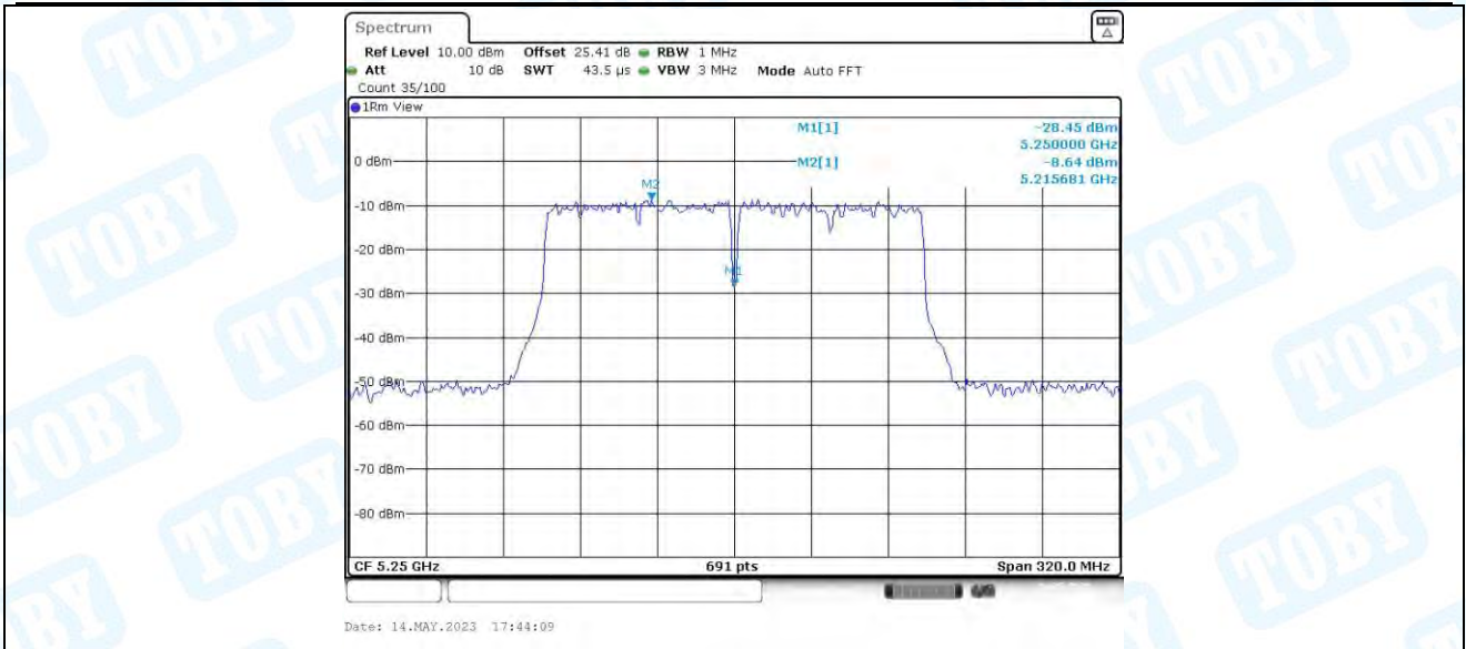
11AC160MIMO_Ant3_5250_UNII-1
