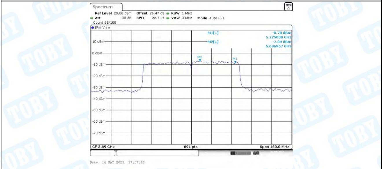
11AC80MIMO_Ant1_5690_UNII-3
