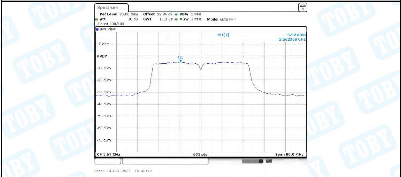
11AC40MIMO_Ant4_5670
