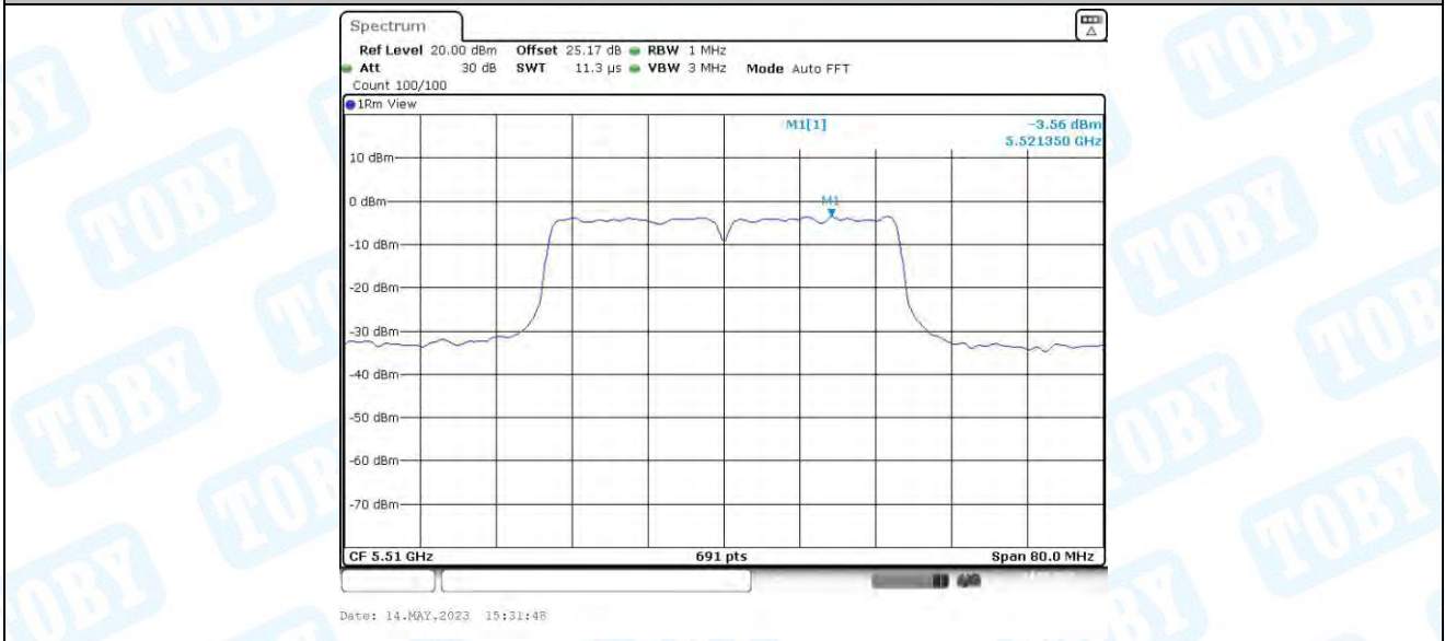
11AC40MIMO_Ant4_5510
