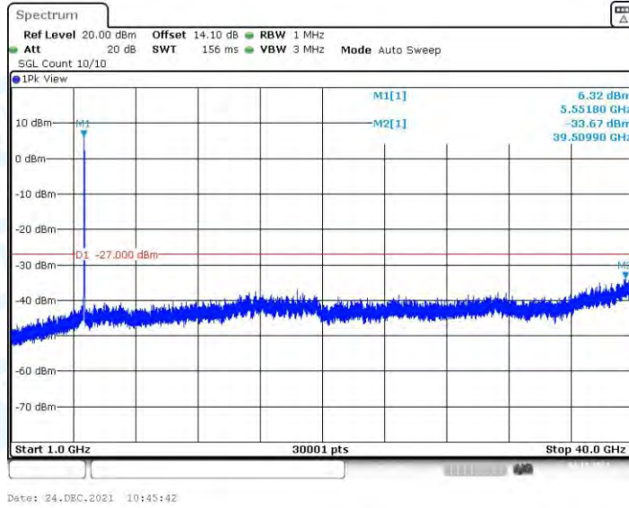
11N40MIMO_Ant3_5550_1000~40000
