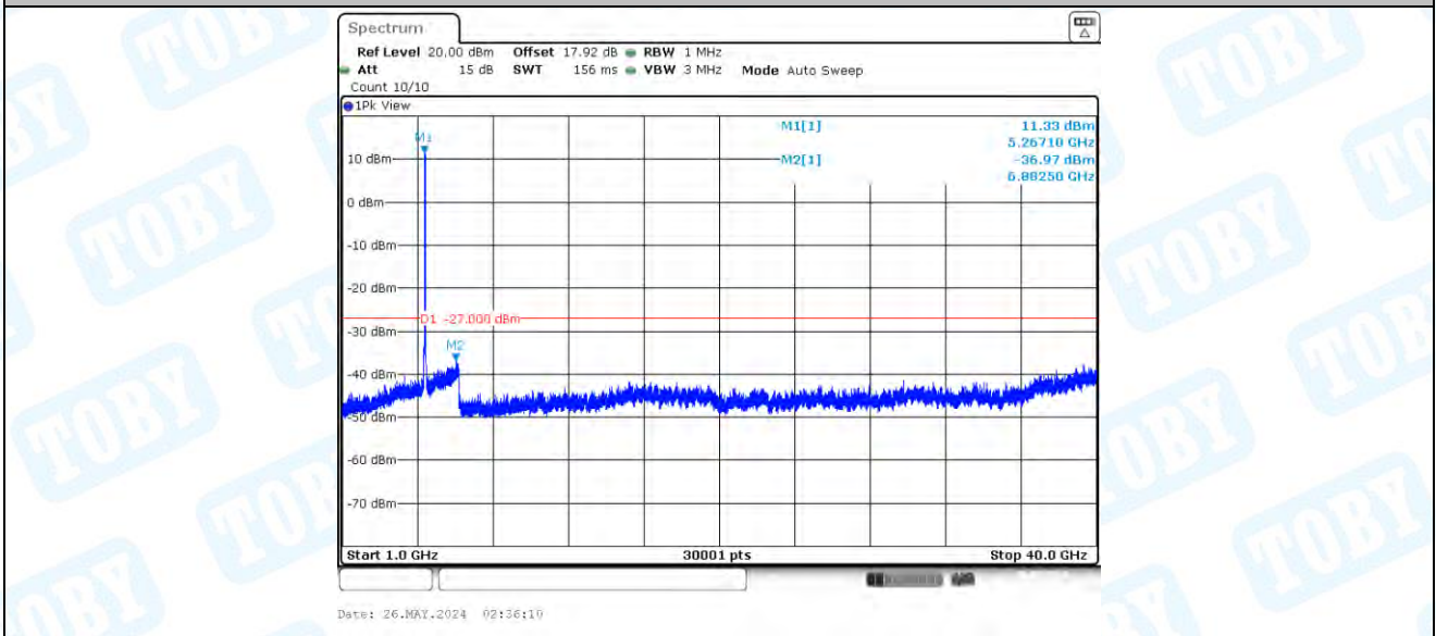
11AC40MIMO_Ant1_5310_30~1000
