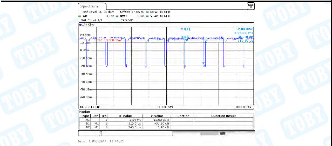
11AX40_Ant3_5510
