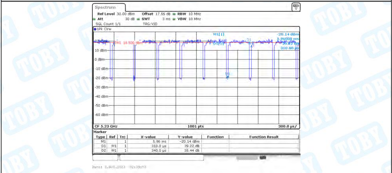
11AX40_Ant3_5230
