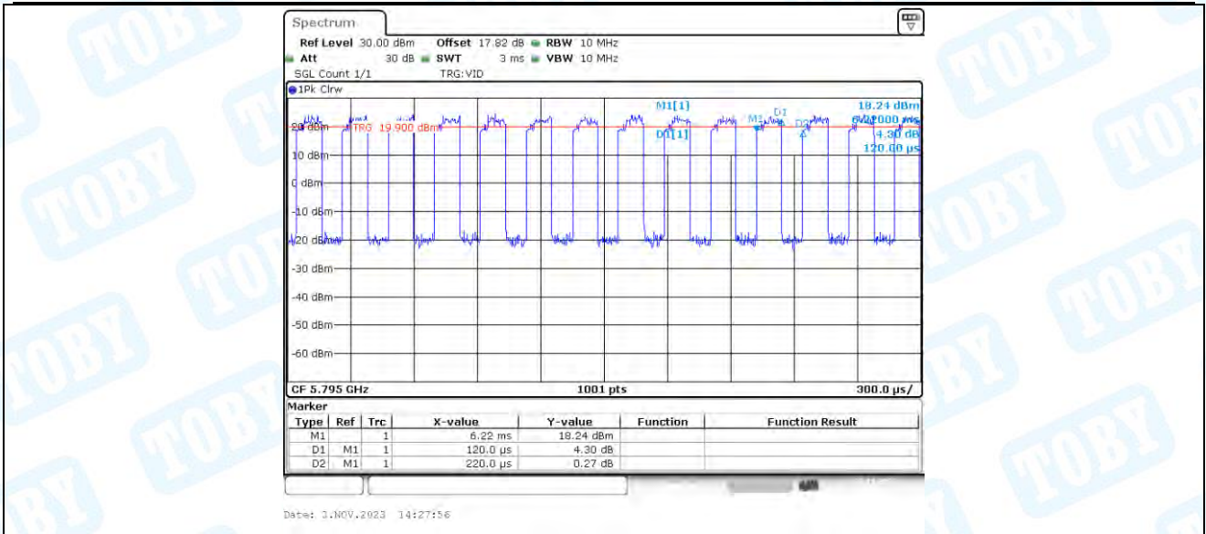
11N40_Ant3_5795
