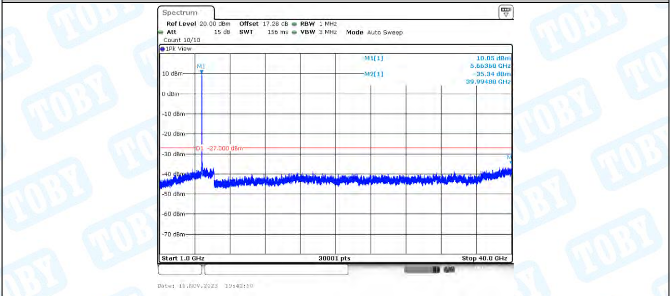
11N40-CDD_Ant1_5710_30~1000
