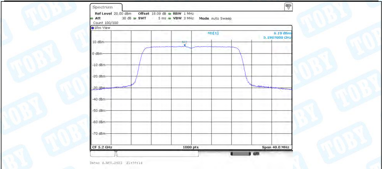
11AX20-BF_Ant2_5200
