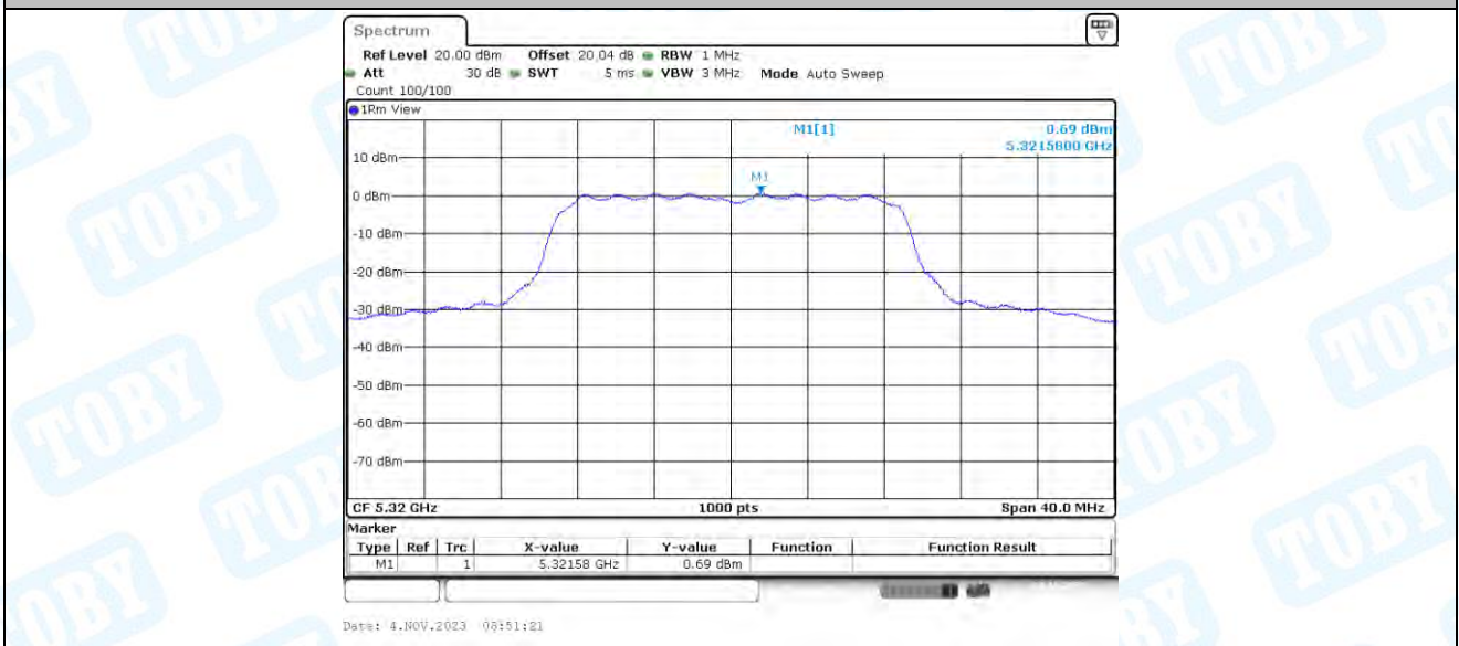
11N20-BF_Ant3_5320
