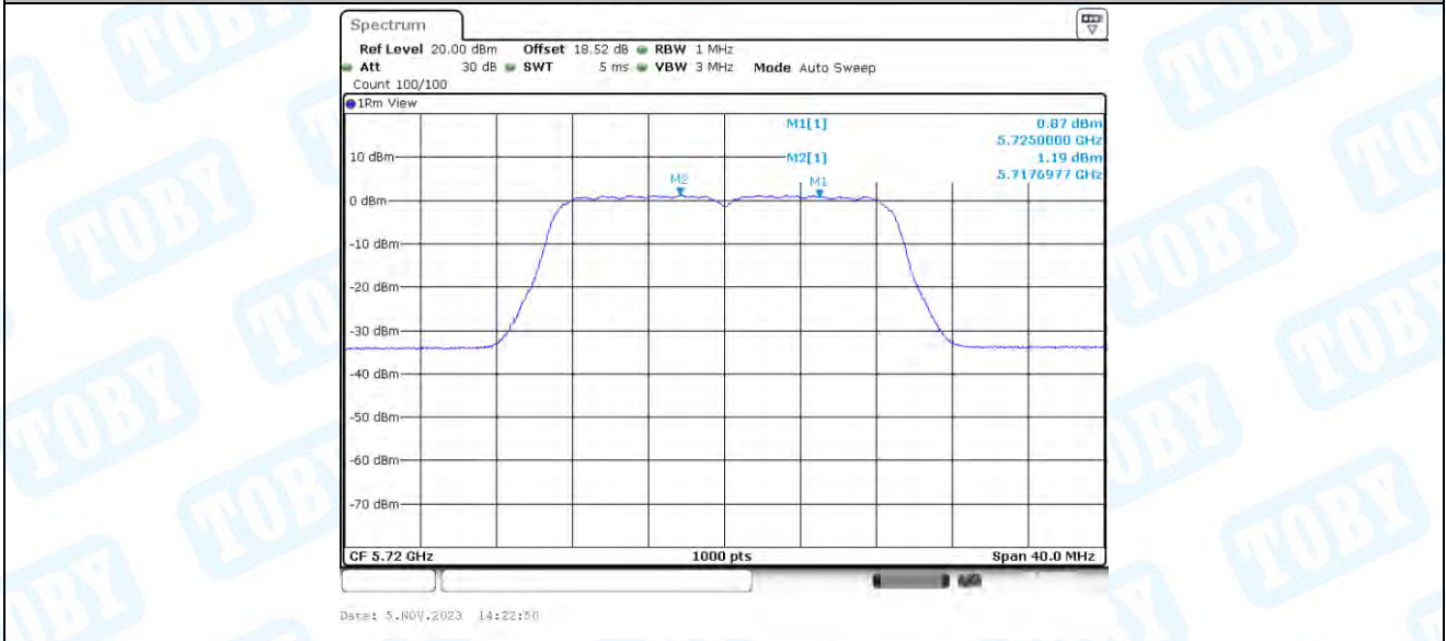
11AC20-BF_Ant3_5720_UNII-2C
