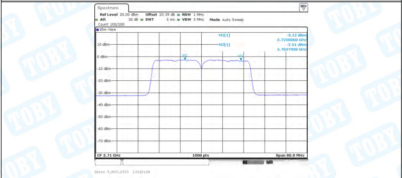
11N40-BF_Ant2_5710_UNII-2C
