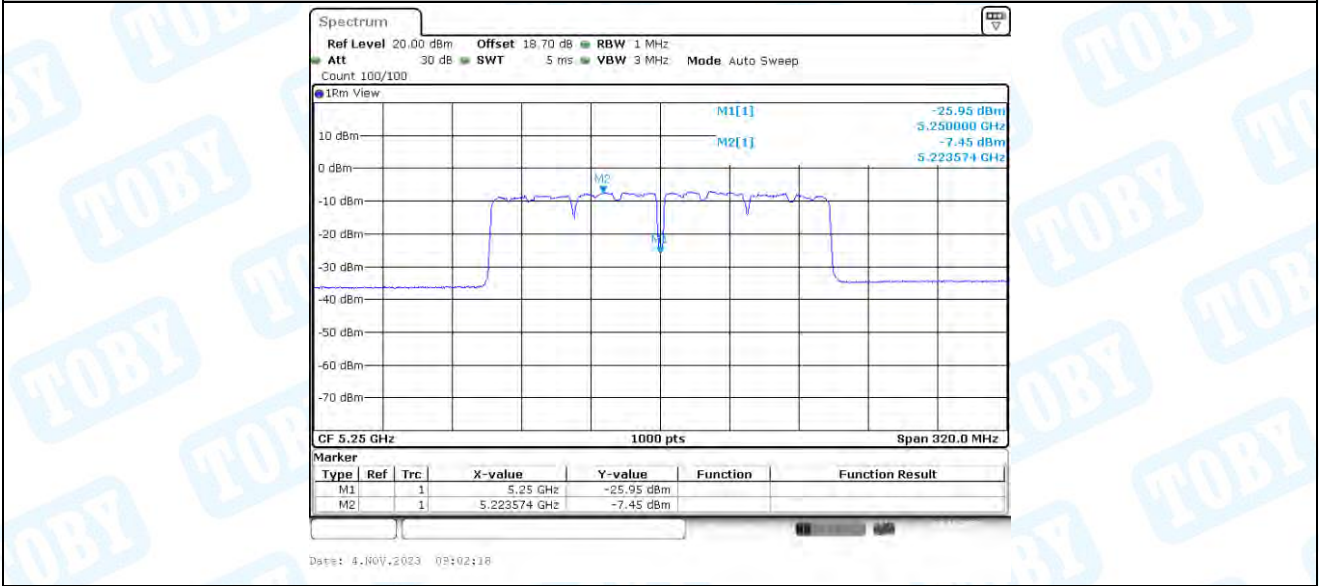
11AC160-BF_Ant1_5250_UNII-2A
