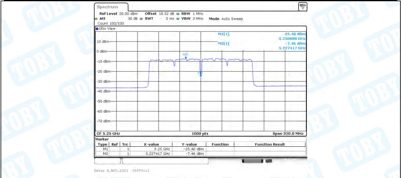
11AC160-BF_Ant3_5250_UNII-1
