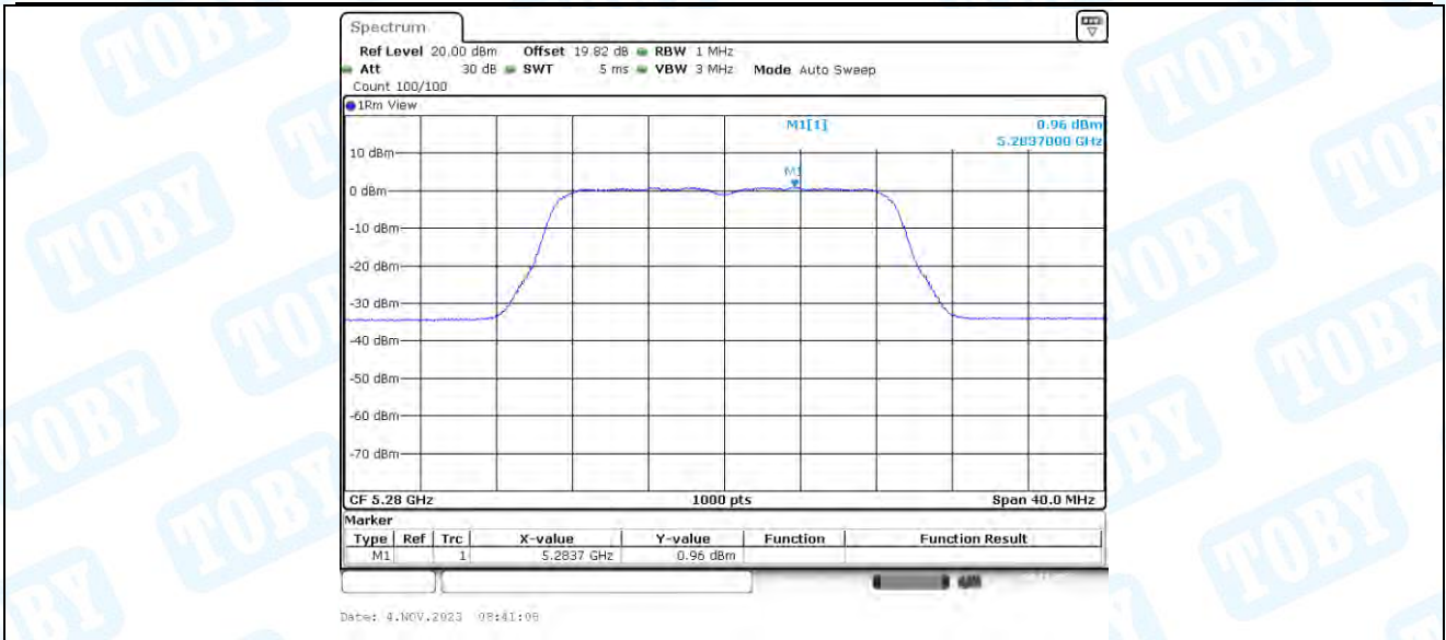
11N20-BF_Ant2_5280
