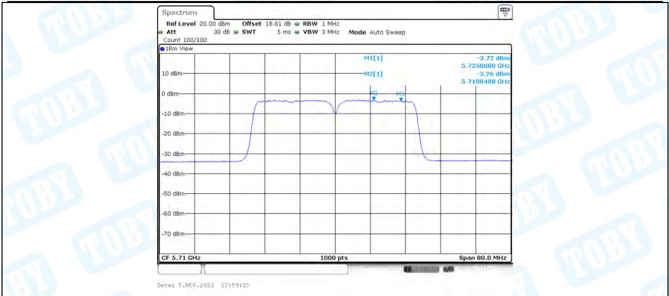
11AC40-BF_Ant1_5710_UNII-3
