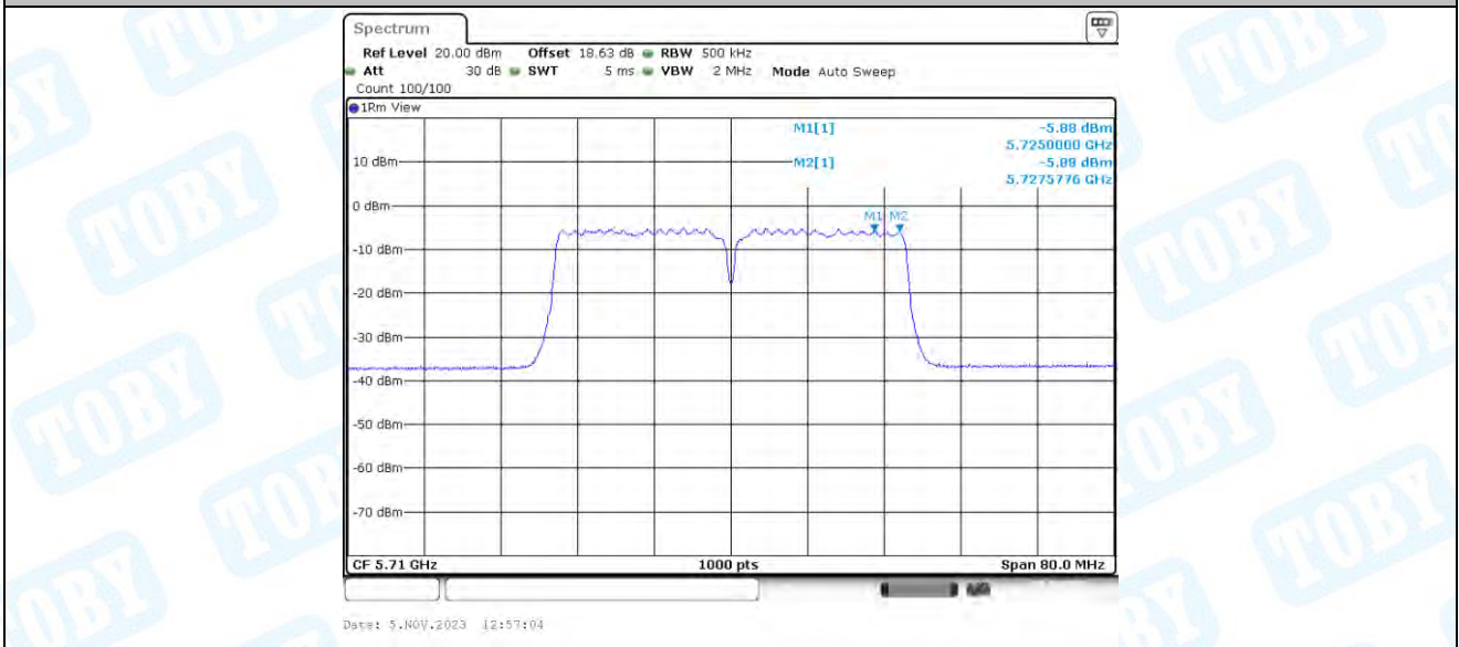
11AC40-BF_Ant3_5710_UNII-3
