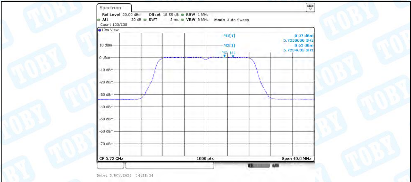
11AC20-BF_Ant2_5720_UNII-2C
