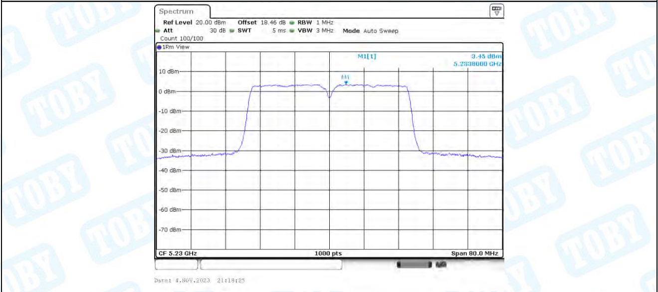
11AC40-BF_Ant3_5230
