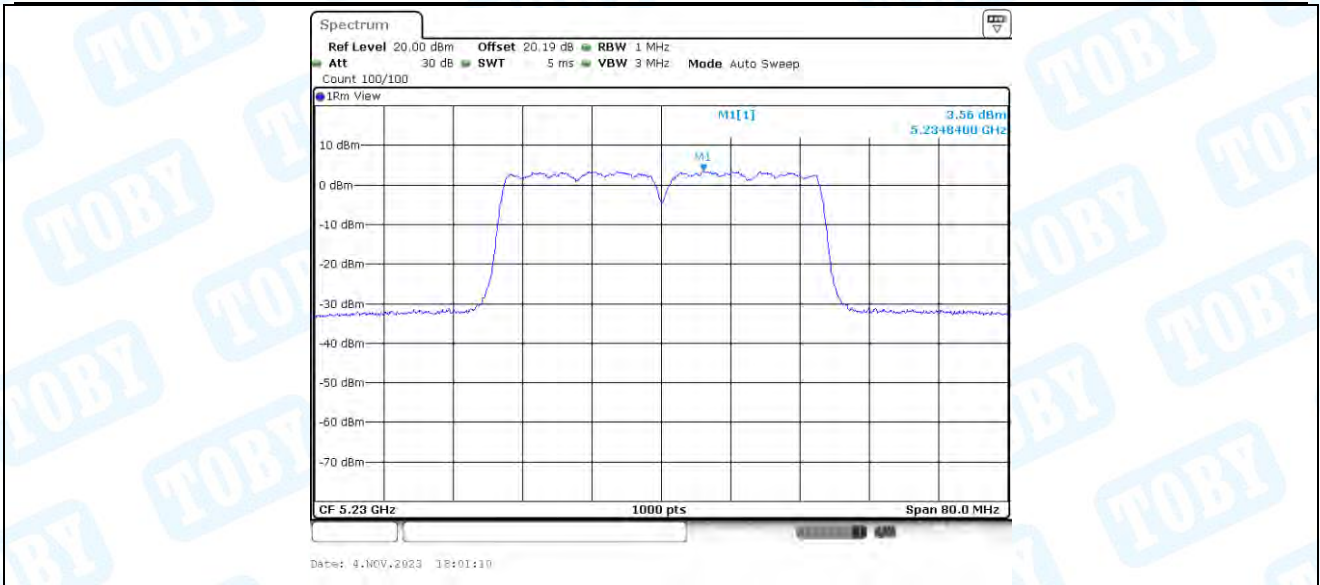
11N40-BF_Ant3_5230
