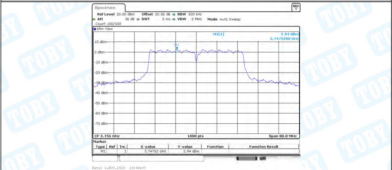
11N40-BF_Ant3_5755
