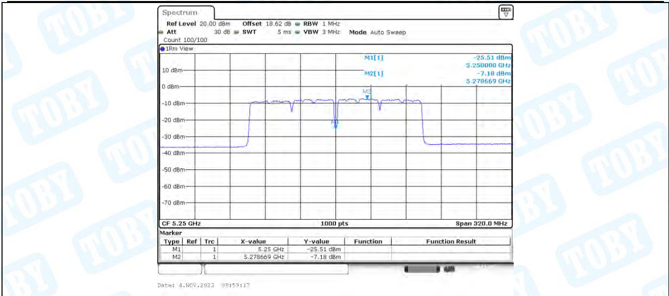
11AC160-BF_Ant2_5250_UNII-2A
