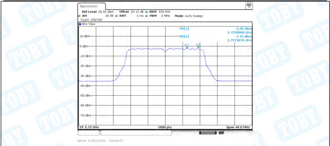
11N20-BF_Ant2_5720_UNII-3
