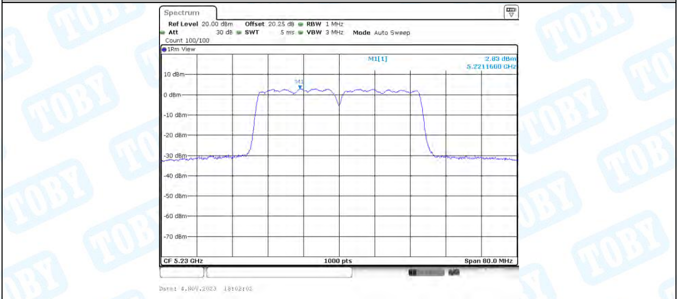
11N40-BF_Ant4_5230
