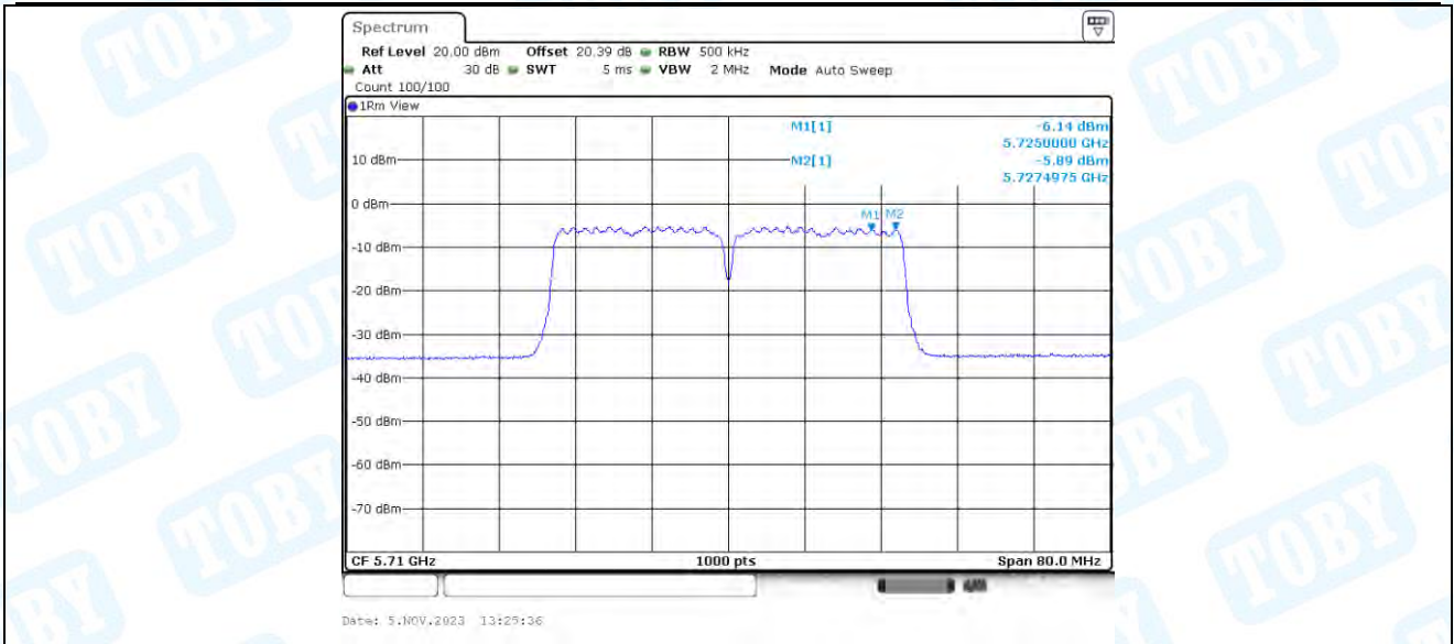
11N40-BF_Ant2_5710_UNII-3
