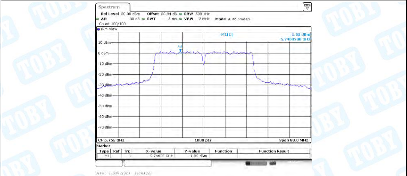
11N40-BF_Ant2_5755
