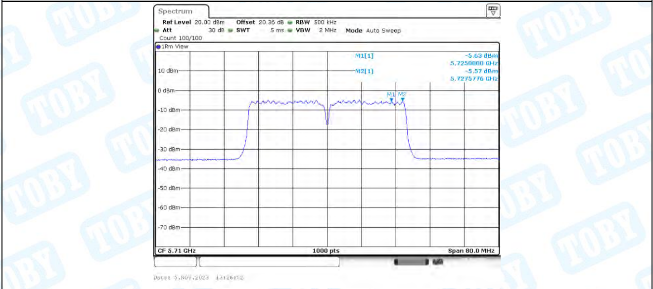
11N40-BF_Ant3_5710_UNII-3
