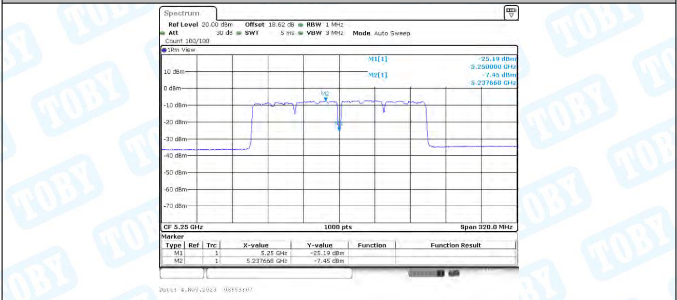
11AC160-BF_Ant2_5250_UNII-1
