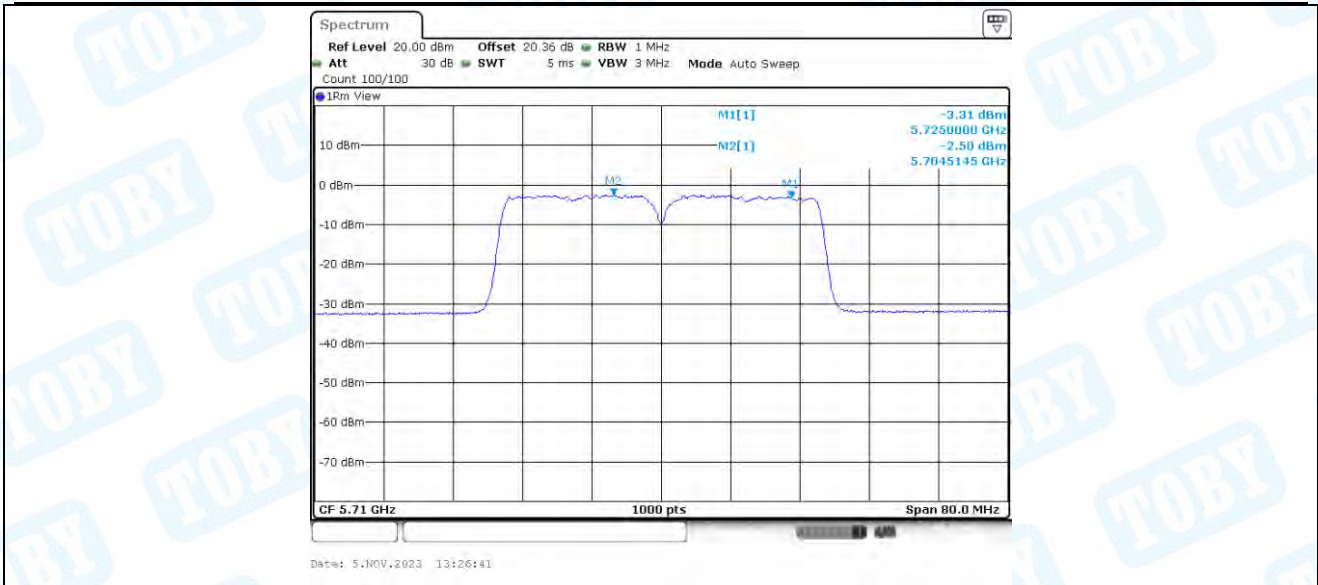
11N40-BF_Ant3_5710_UNII-2C
