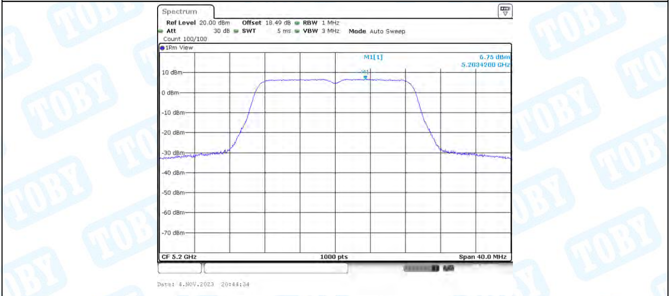
11AC20-BF_Ant2_5200
