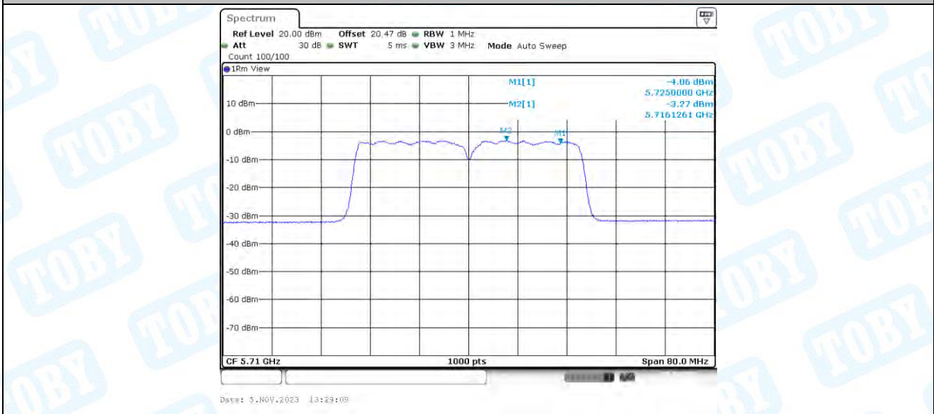
11N40-BF_Ant1_5710_UNII-3
