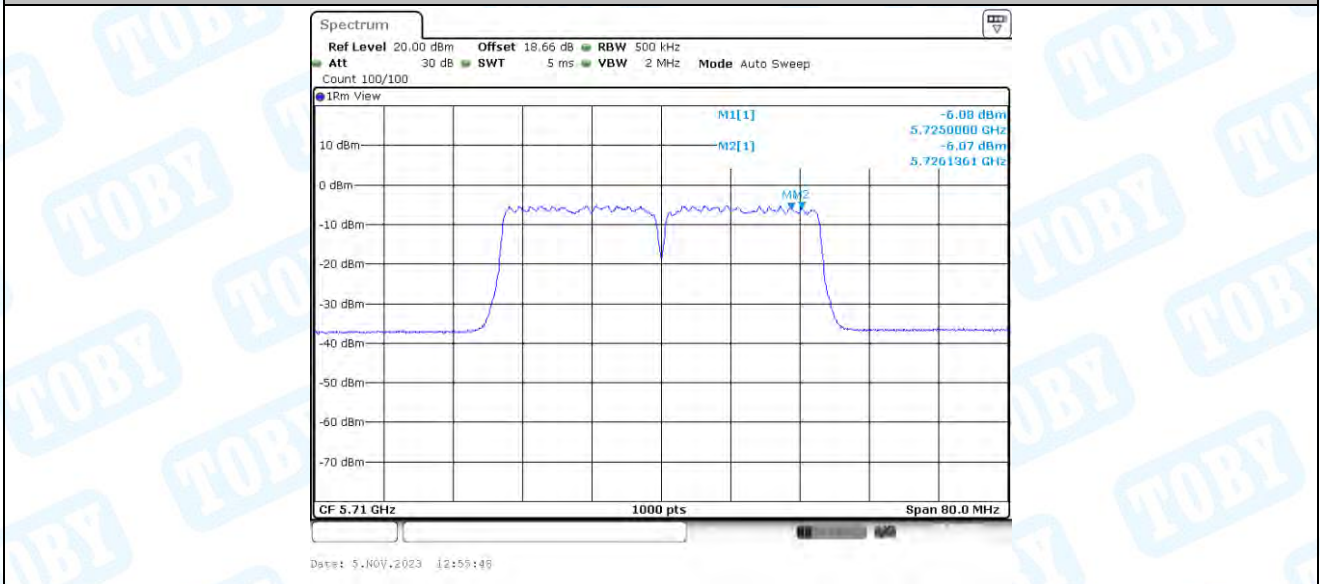
11AC40-BF_Ant2_5710_UNII-3
