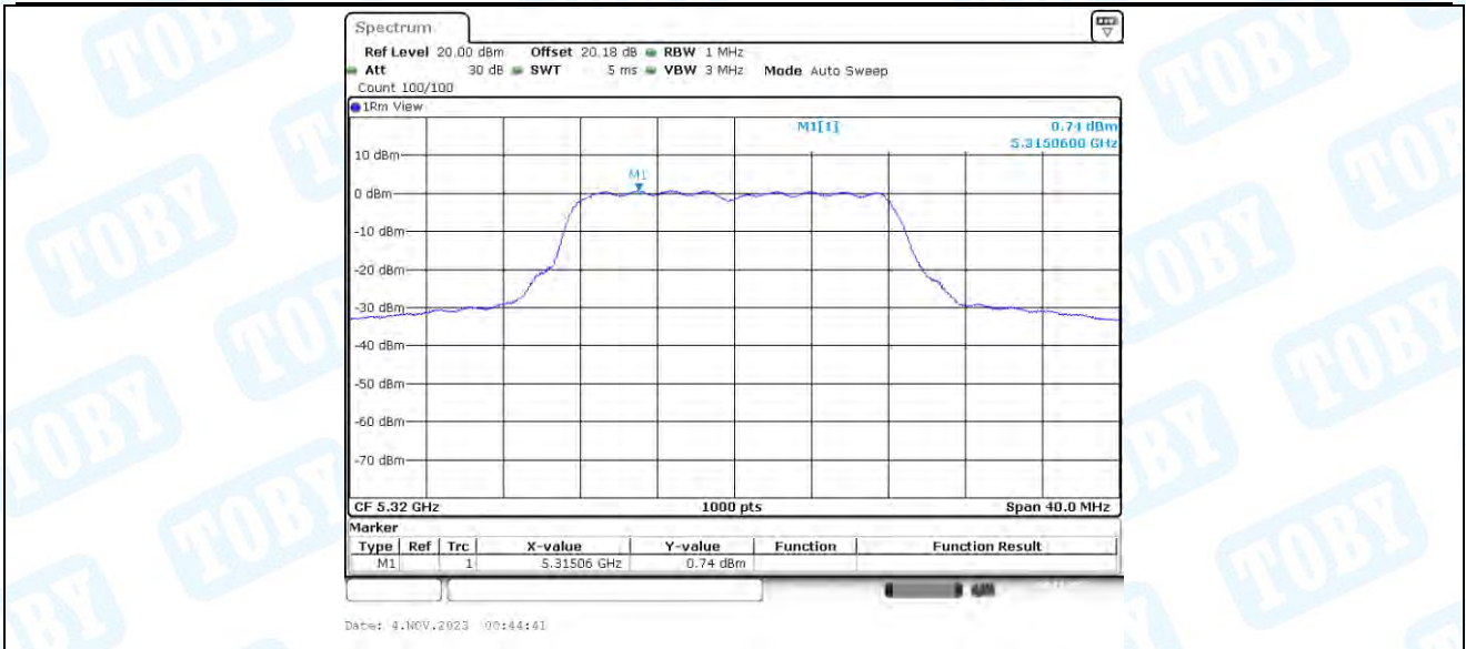
11A-BF_Ant3_5320
