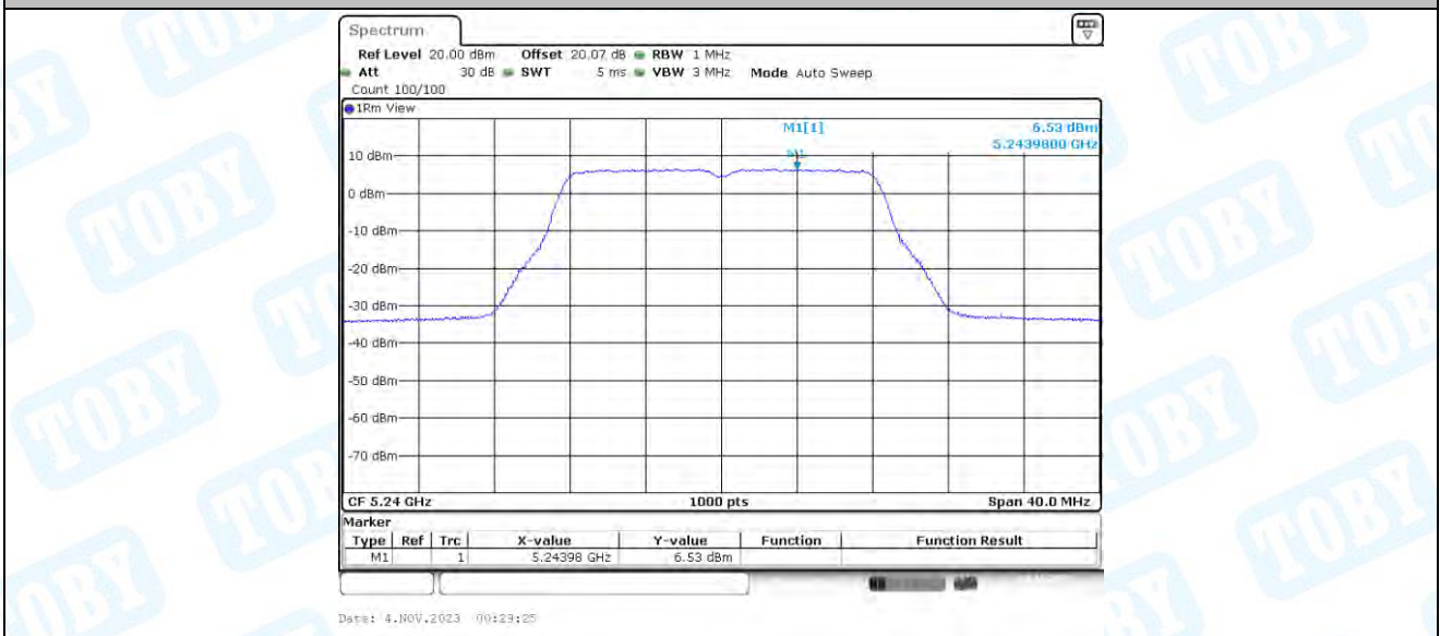
11A-BF_Ant2_5240
