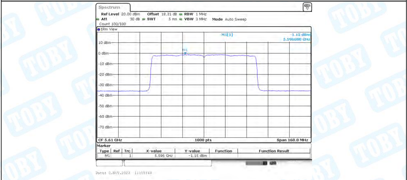
11AX80-CDD_Ant2_5610
