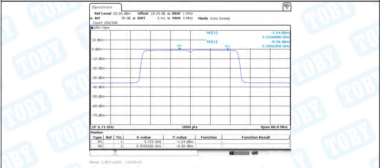
11AX40-CDD_Ant1_5710_UNII-3
