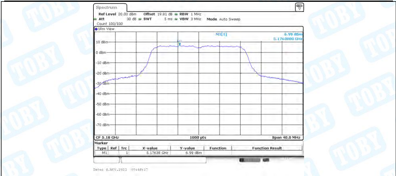
11N20-BF_Ant3_5180
