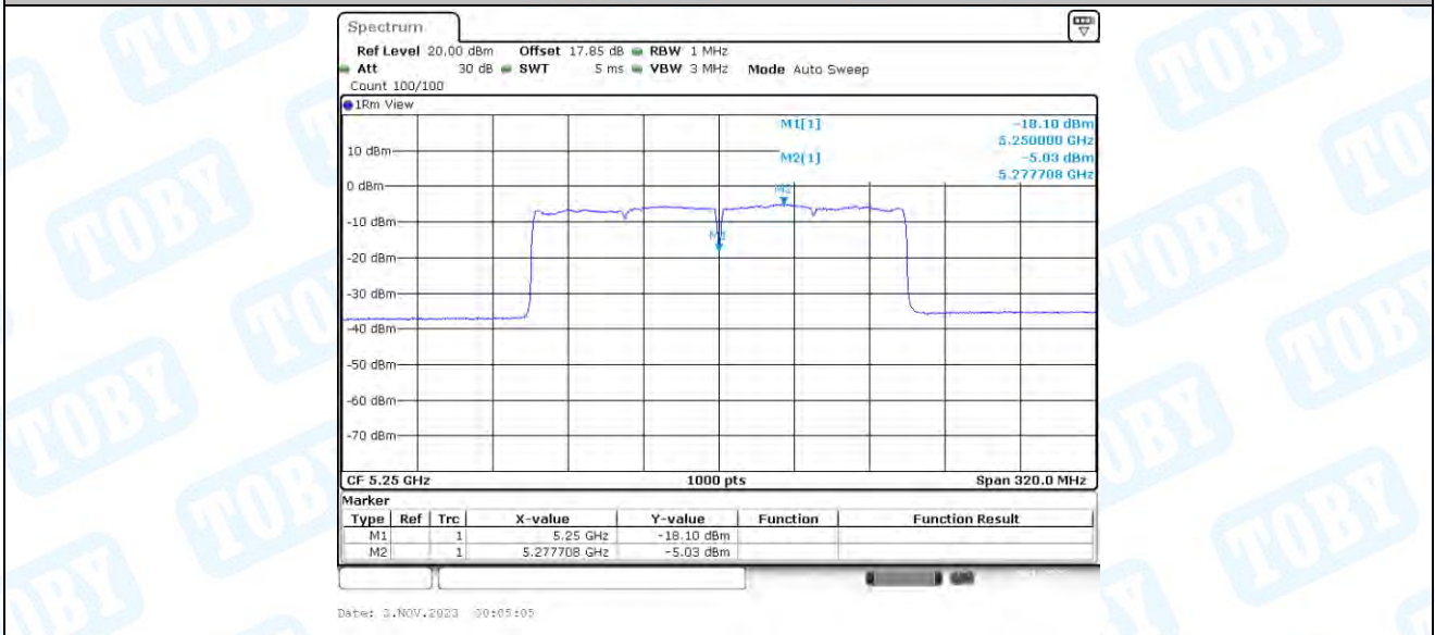
11AX160-CDD_Ant2_5250_UNII-2A
