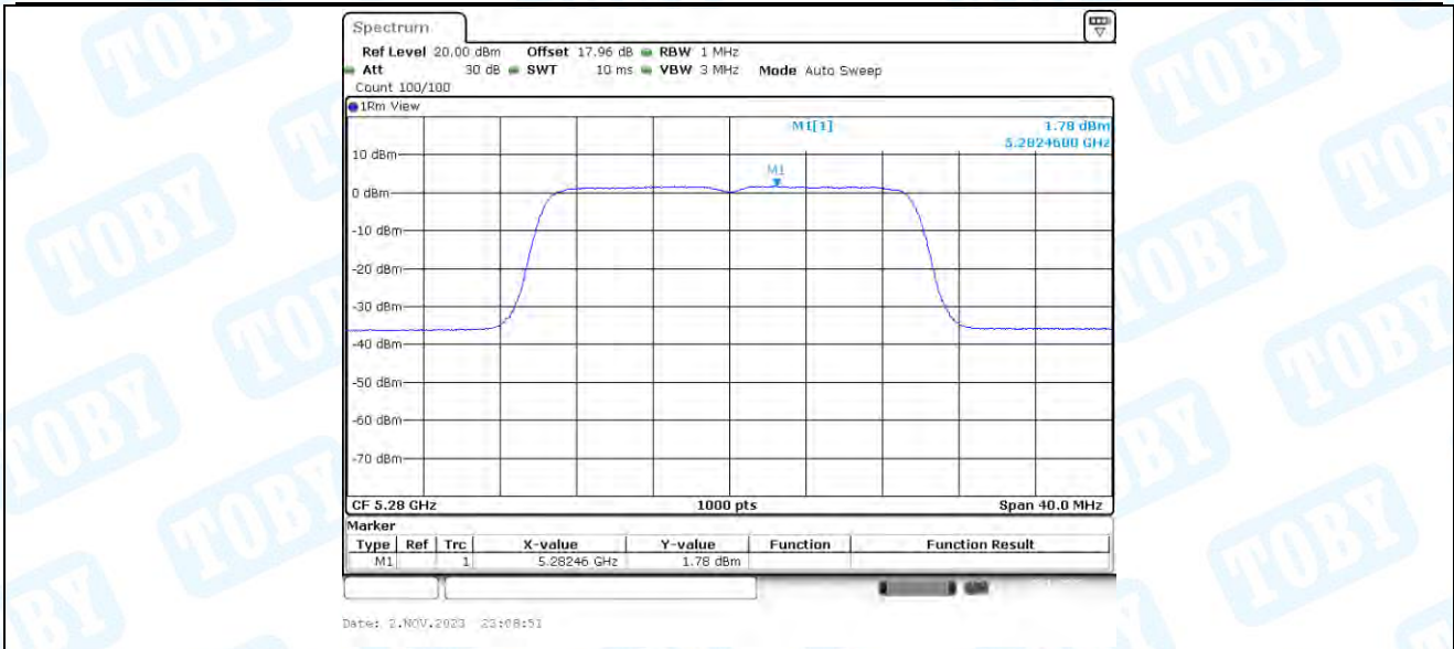
11AX20-CDD_Ant3_5280
