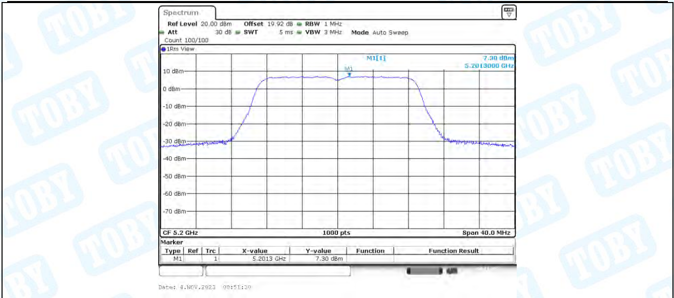
11N20-BF_Ant2_5200
