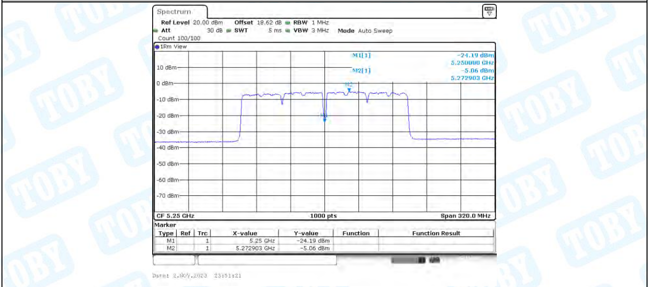
11AC160-CDD_Ant2_5250_UNII-2A
