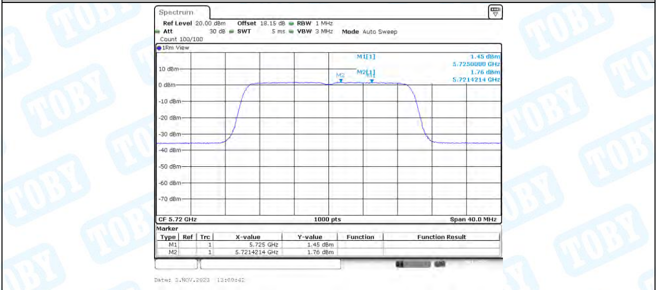
11AX20-CDD_Ant2_5720_UNII-2C
