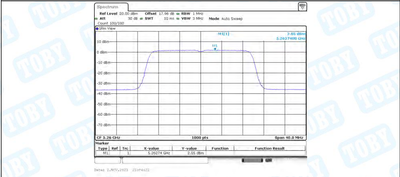
11AX20-CDD_Ant2_5260
