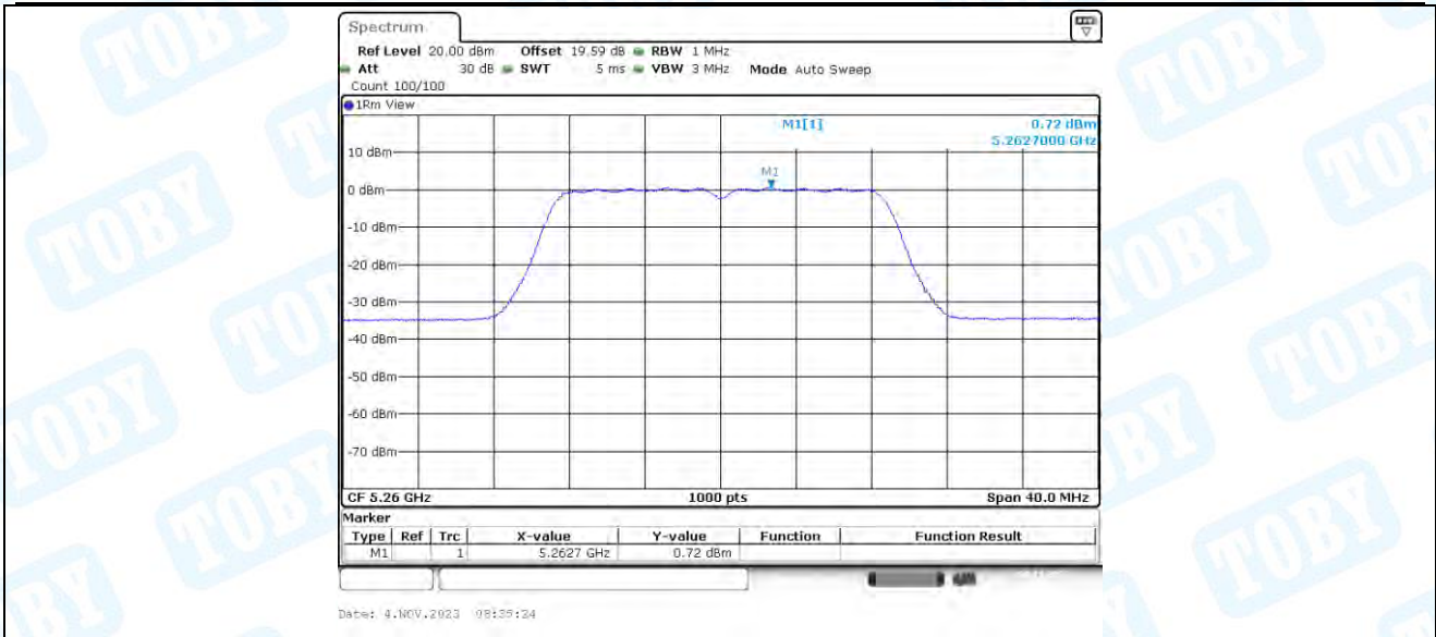
11N20-BF_Ant3_5260
