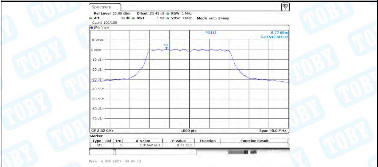
11A-BF_Ant4_5320
