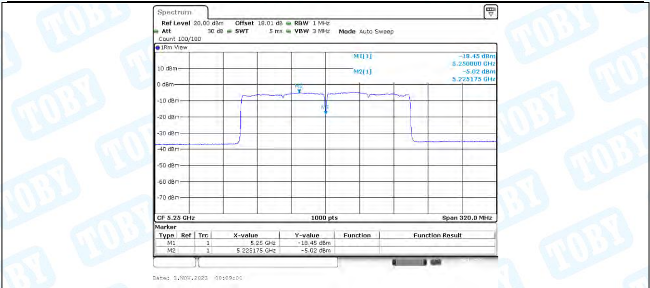
11AX160-CDD_Ant1_5250_UNII-2A
