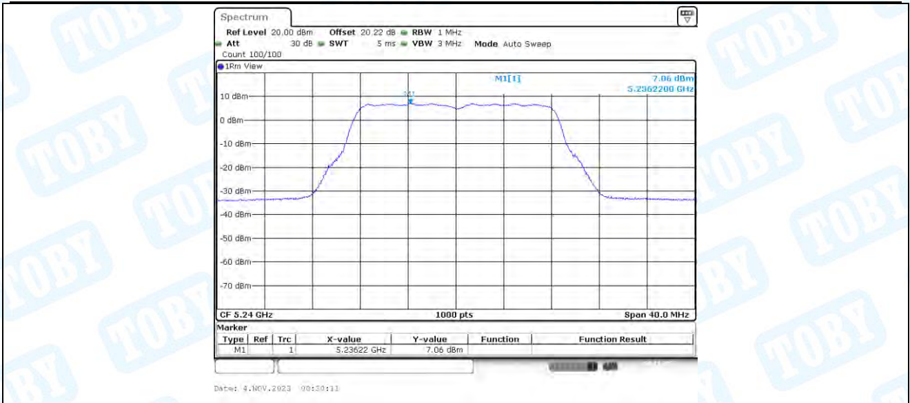
11A-BF_Ant3_5240
