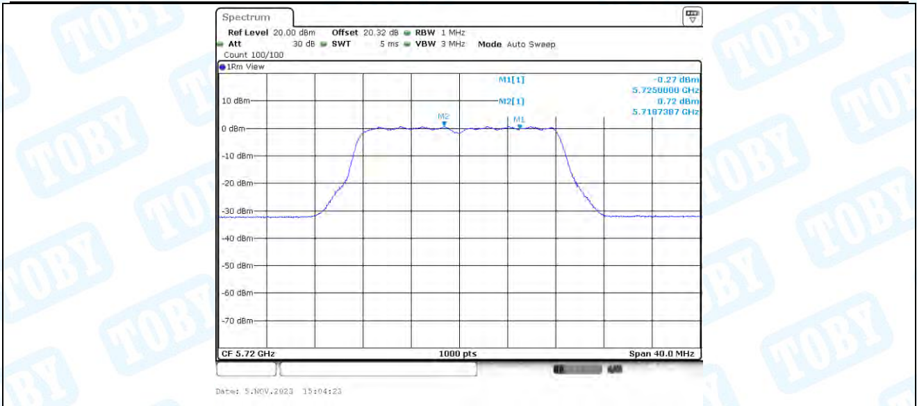
11A-BF_Ant1_5720_UNII-3
