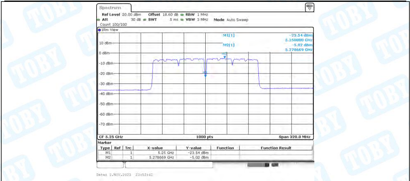
11AC160-CDD_Ant3_5250_UNII-2A
