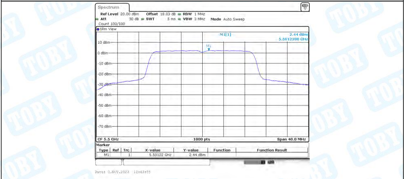
11AX20-CDD_Ant3_5500
