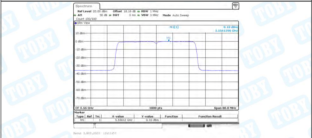
11AX40-CDD_Ant2_5550
