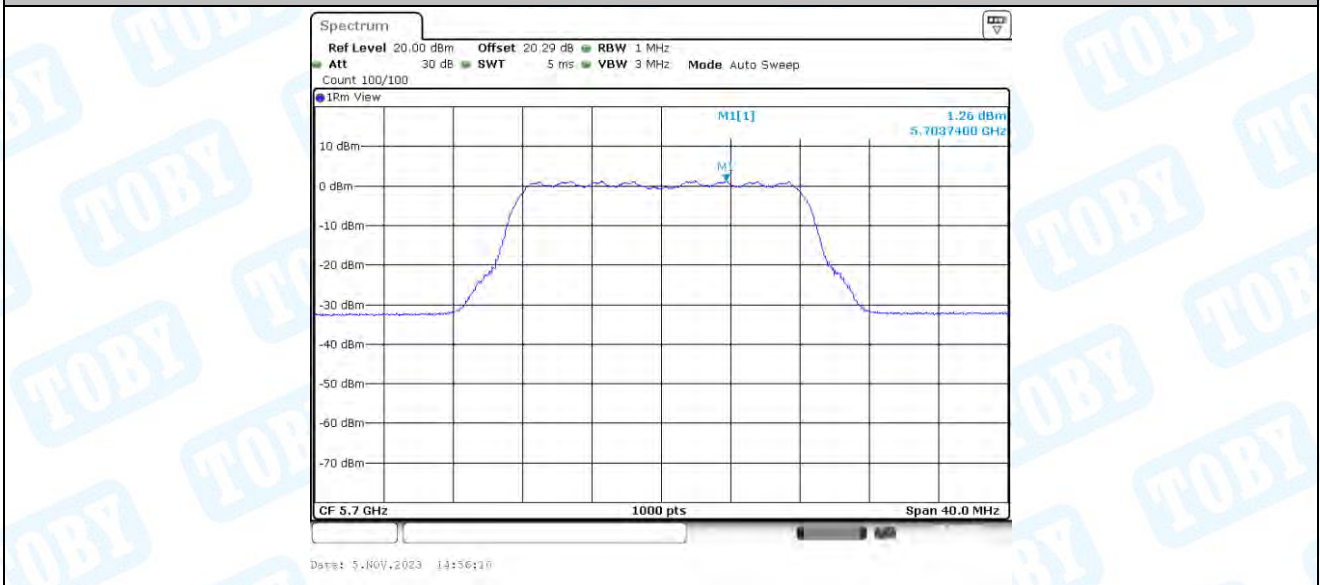
11A-BF_Ant2_5700
