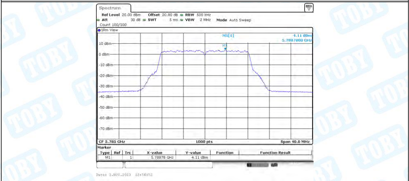
11A-BF_Ant4_5785
