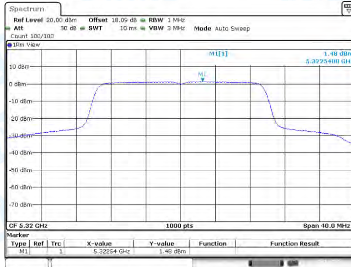
11AX20-CDD_Ant2_5320
