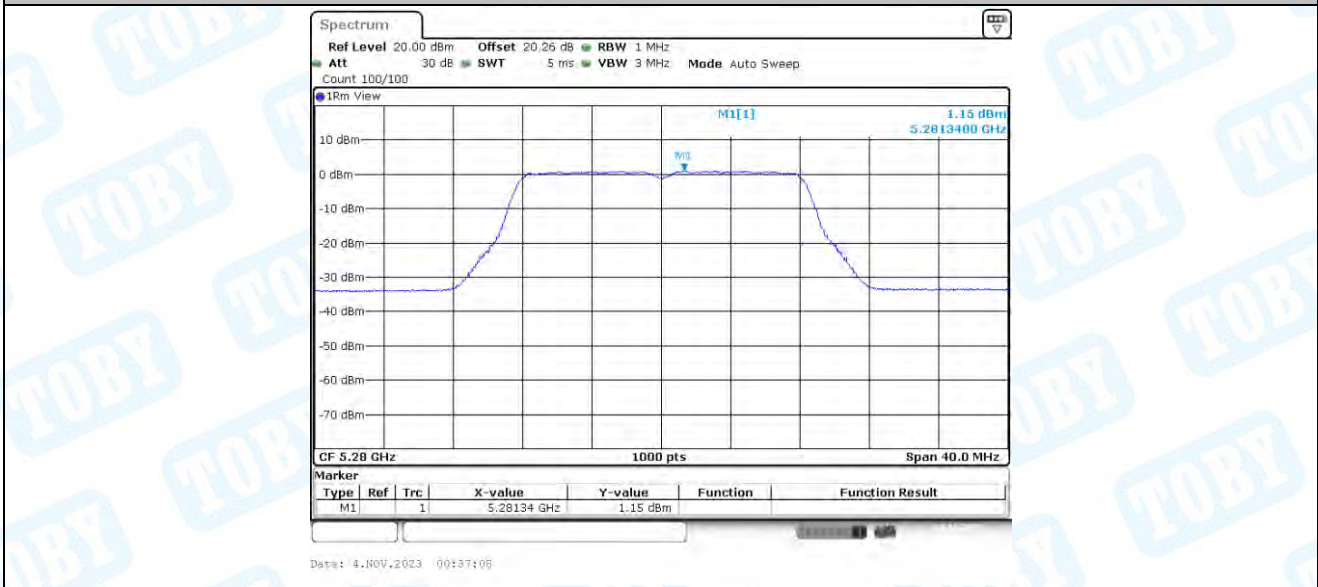
11A-BF_Ant2_5280
