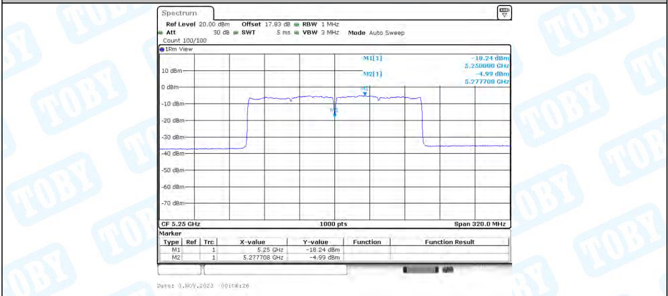
11AX160-CDD_Ant3_5250_UNII-2A
