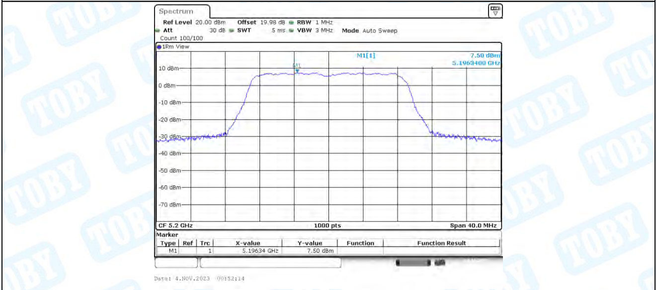
11N20-BF_Ant3_5200
