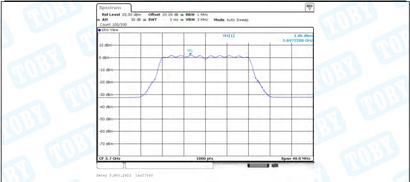
11A-BF_Ant3_5700
