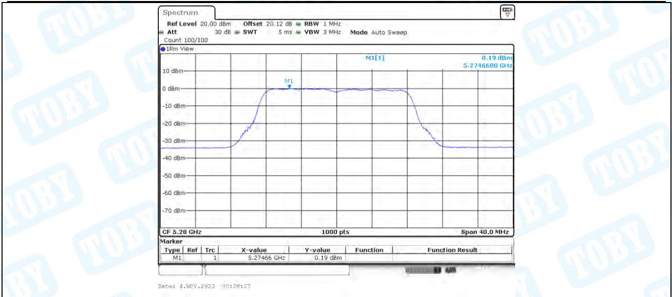
11A-BF_Ant4_5280
