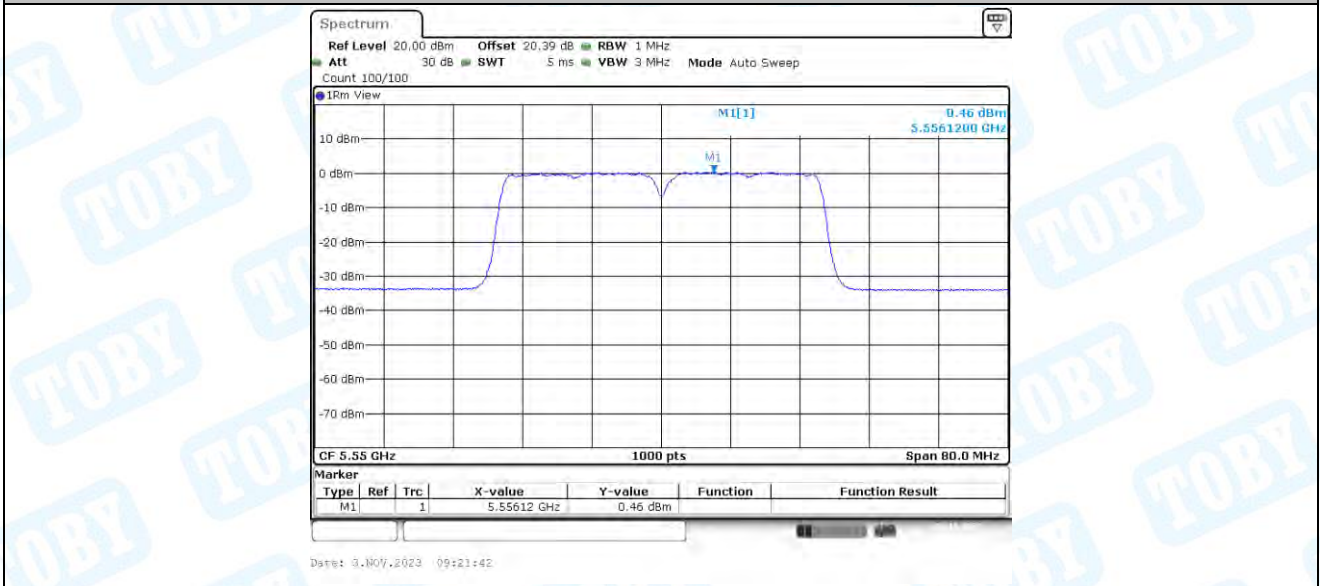
11N40-CDD_Ant2_5550
