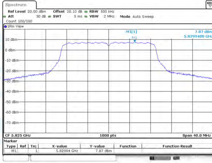
11N20-CDD_Ant3_5825
