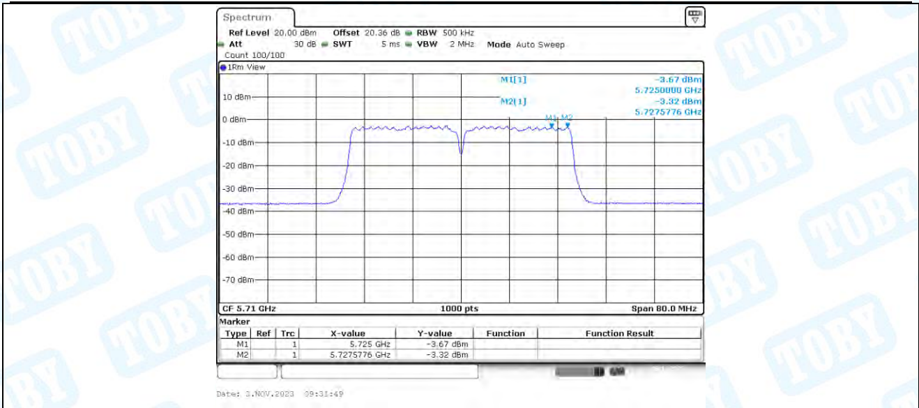
11N40-CDD_Ant3_5710_UNII-3
