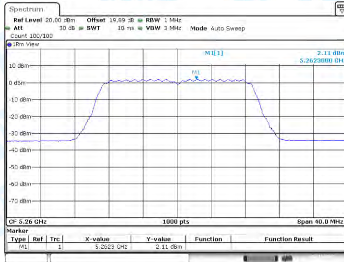
11N20-CDD_Ant2_5260
