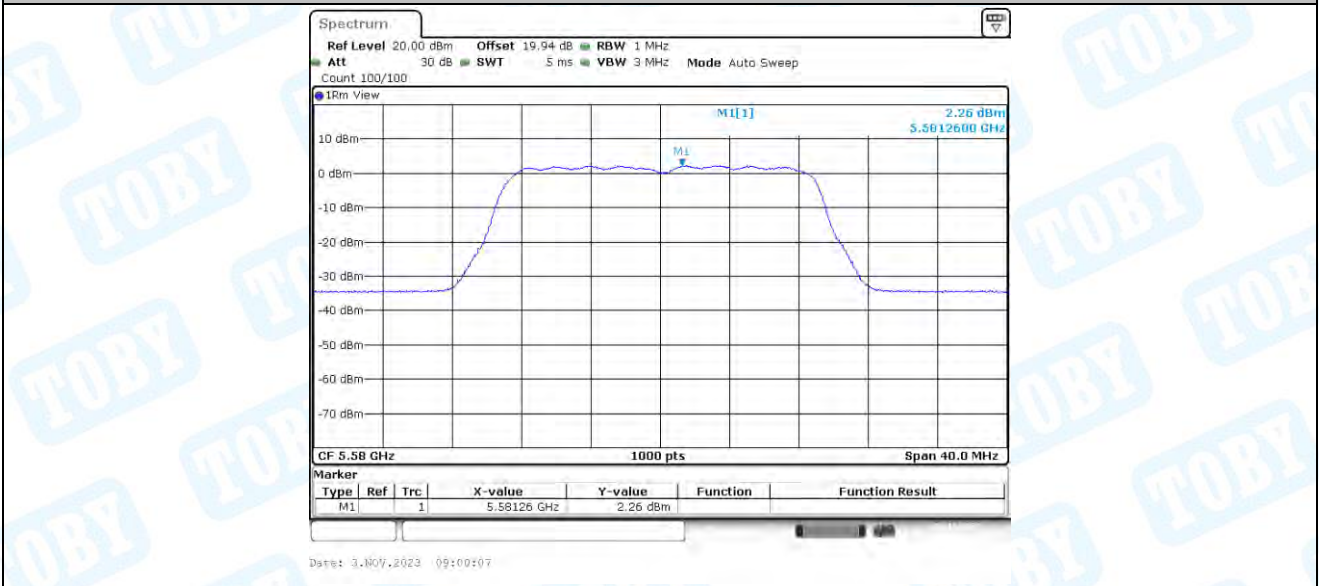
11N20-CDD_Ant2_5580
