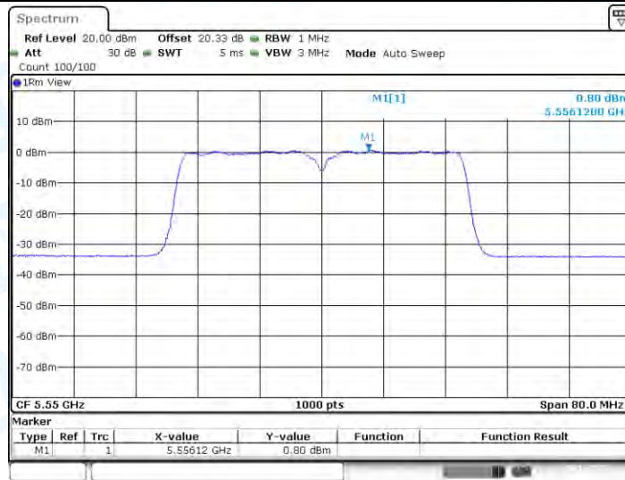
11N40-CDD_Ant3_5550
