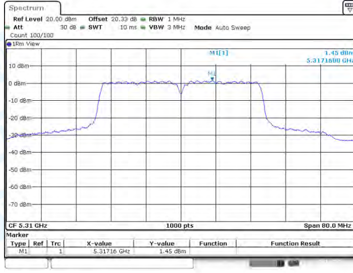
11N40-CDD_Ant2_5310
