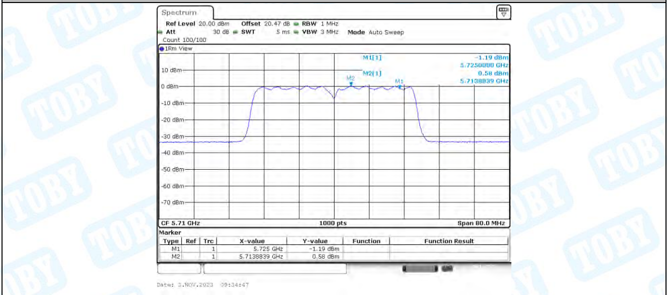
11N40-CDD_Ant1_5710_UNII-3
