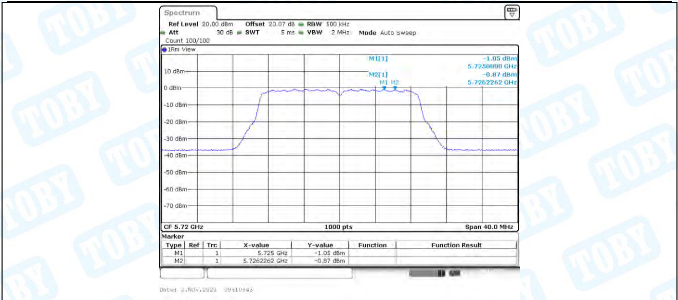
11N20-CDD_Ant3_5720_UNII-3
