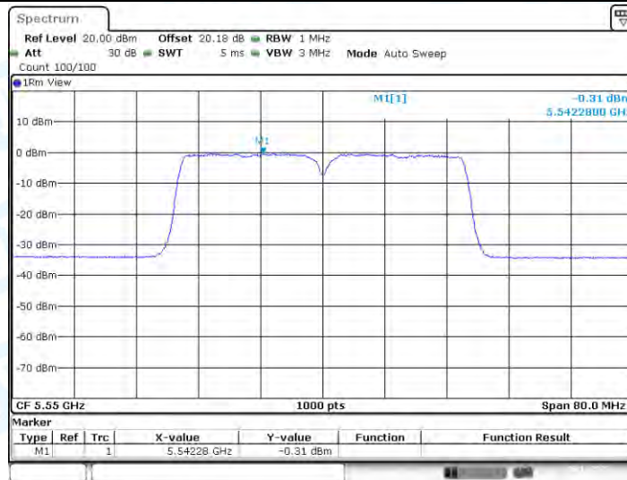
11N40-CDD_Ant3_5550
