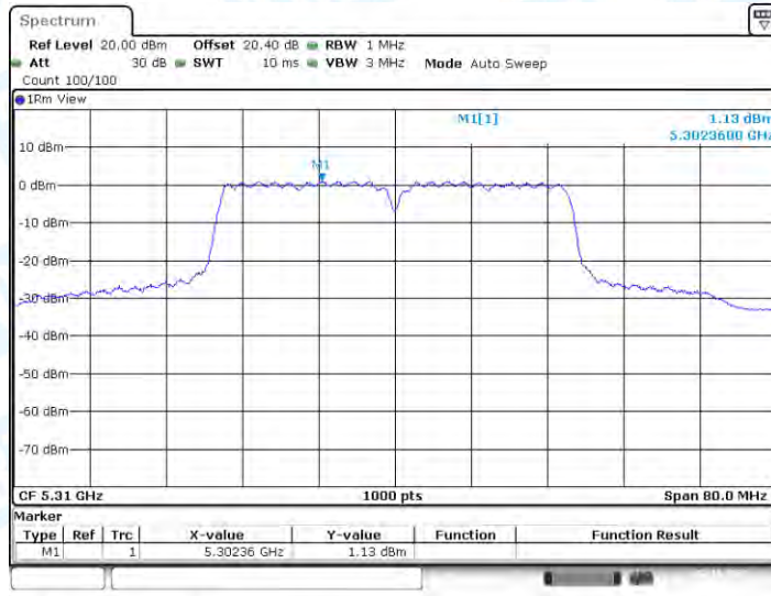
11N40-CDD_Ant3_5310
