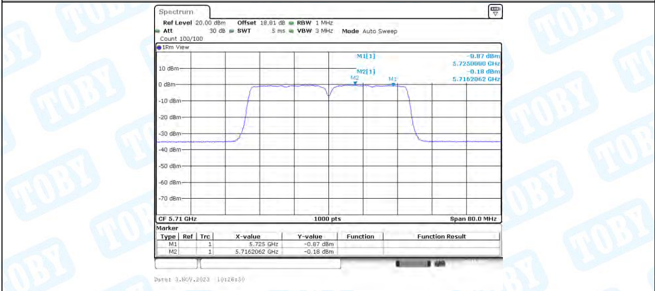
11AC40-CDD_Ant1_5710_UNII-3
