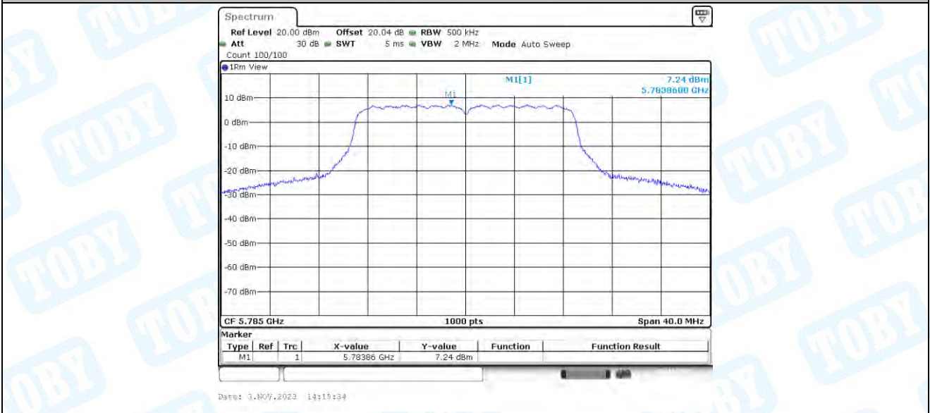
11N20-CDD_Ant3_5785
