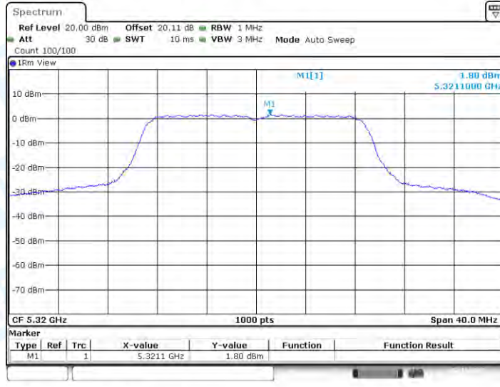
11N20-CDD_Ant3_5320
