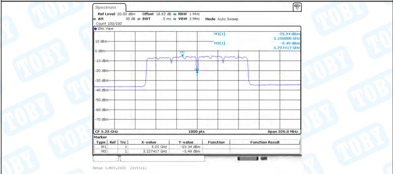
11AC160-CDD_Ant2_5250_UNII-1
