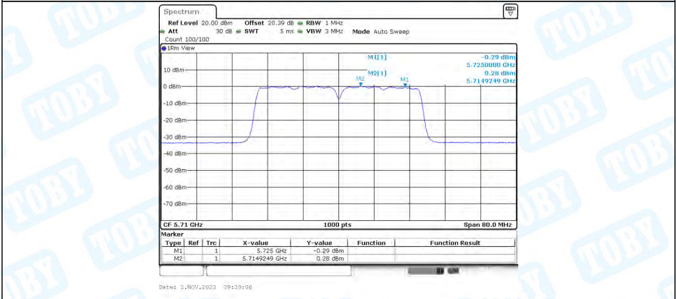
11N40-CDD_Ant2_5710_UNII-2C
