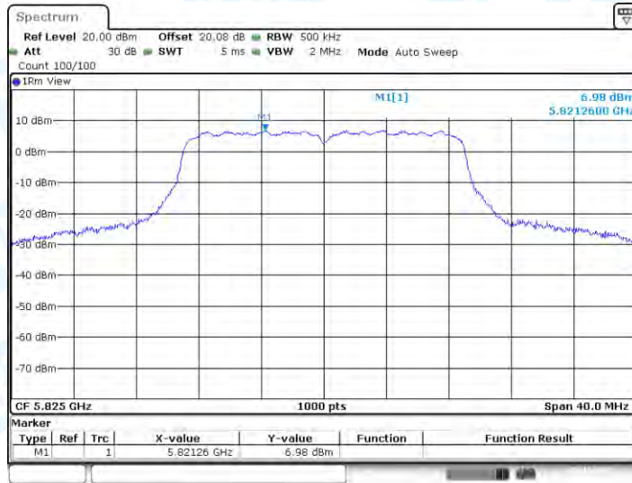
11N20-CDD_Ant4_5825
