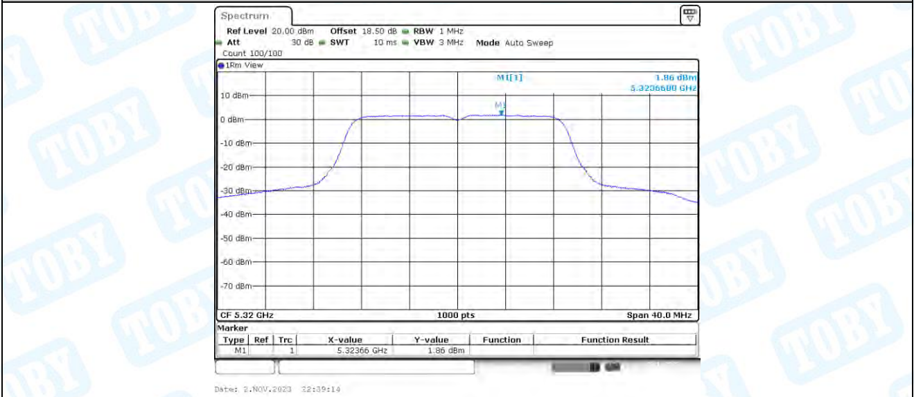
11AC20-CDD_Ant2_5320
