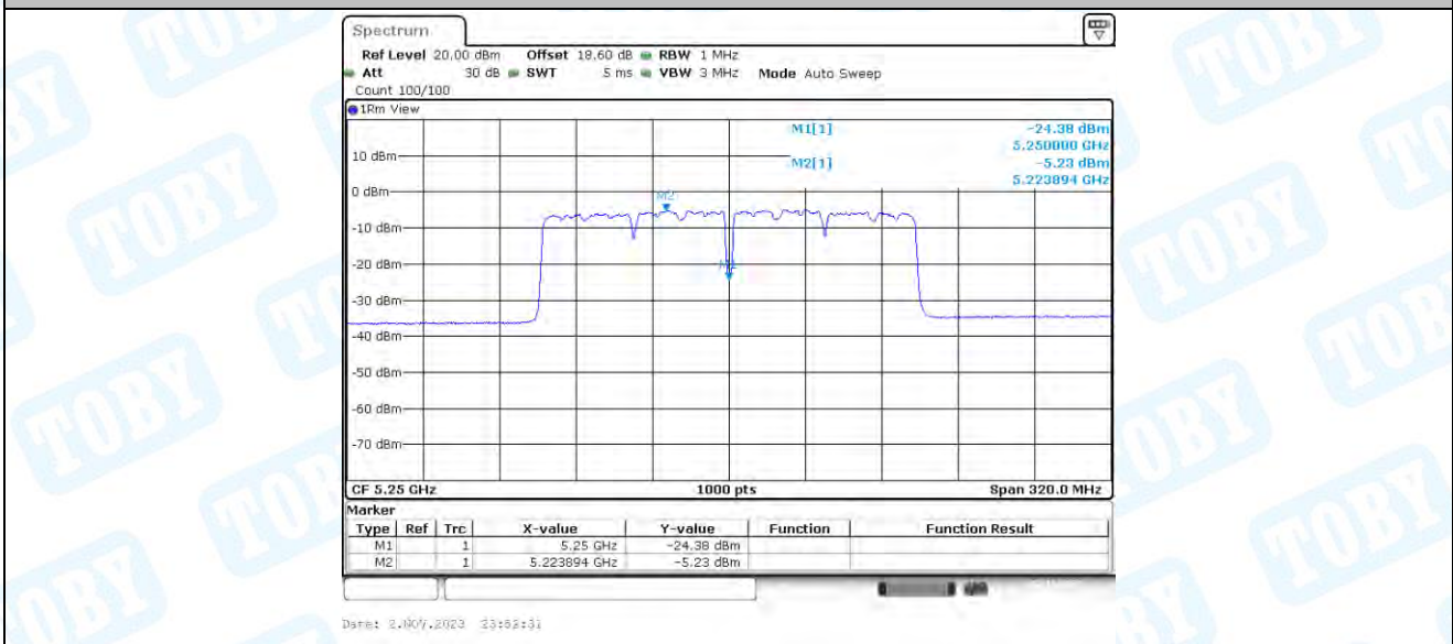
11AC160-CDD_Ant3_5250_UNII-1
