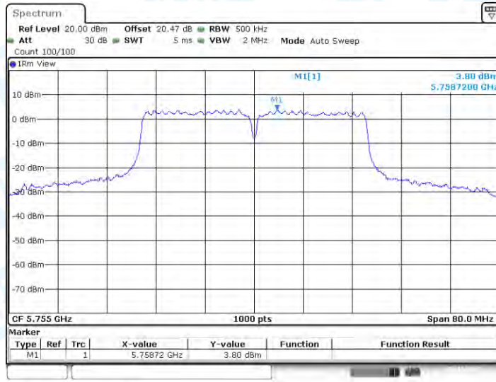
11N40-CDD_Ant3_5755
