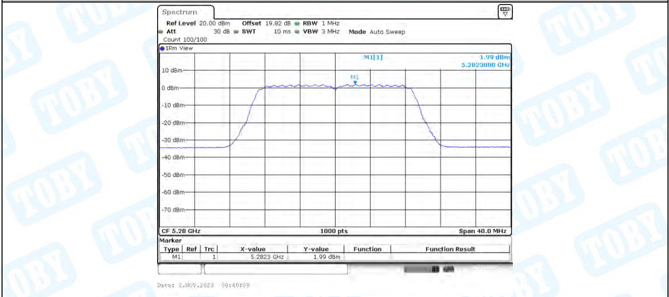
11N20-CDD_Ant2_5280
