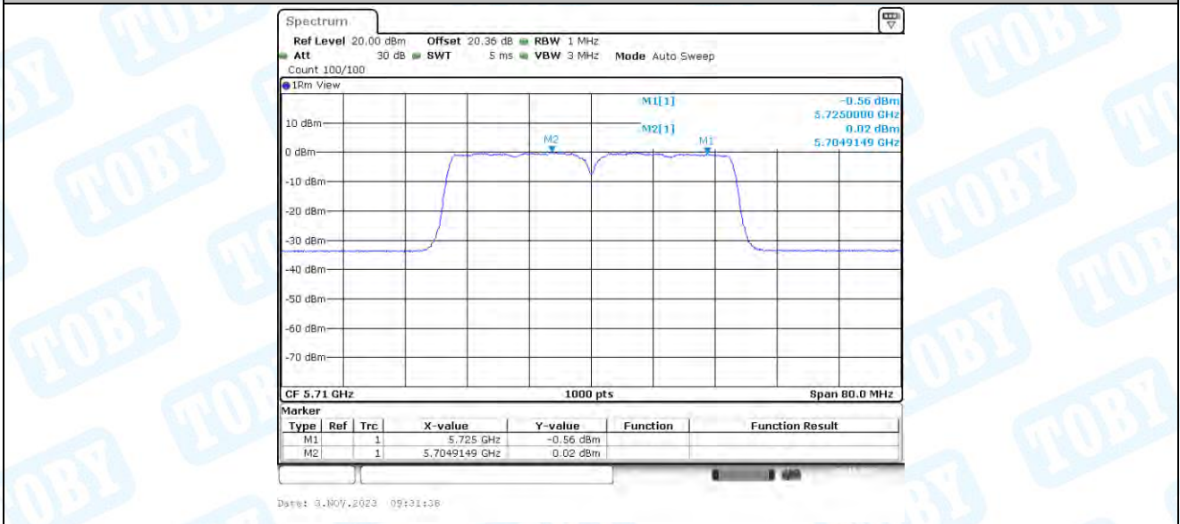
11N40-CDD_Ant3_5710_UNII-2C
