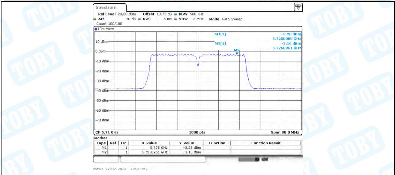
11AC40-CDD_Ant2_5710_UNII-3
