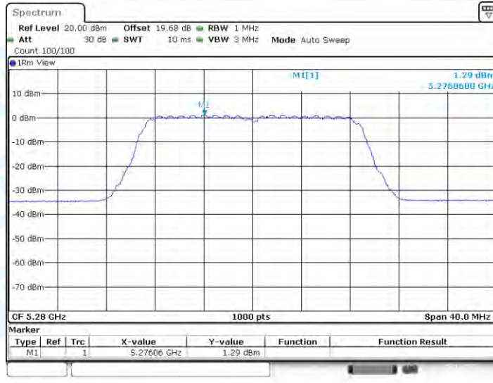
11N20-CDD_Ant3_5280
