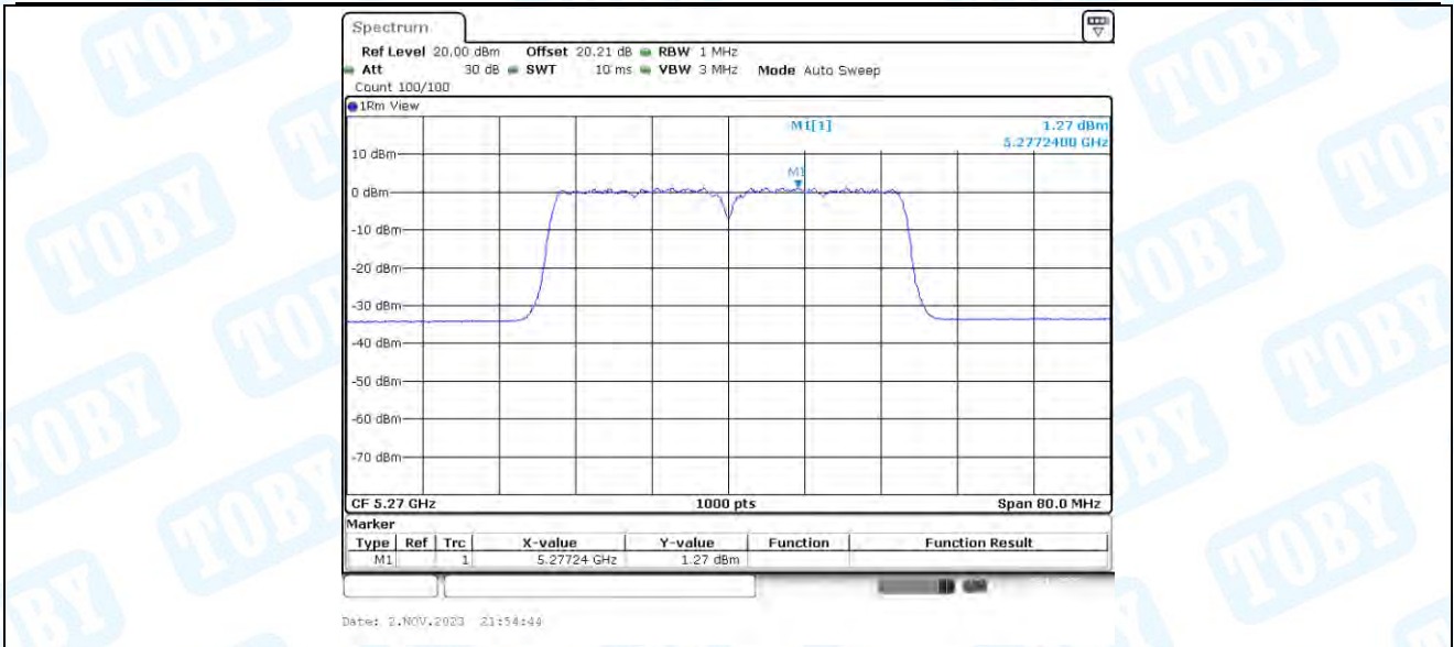
11N40-CDD_Ant3_5270
