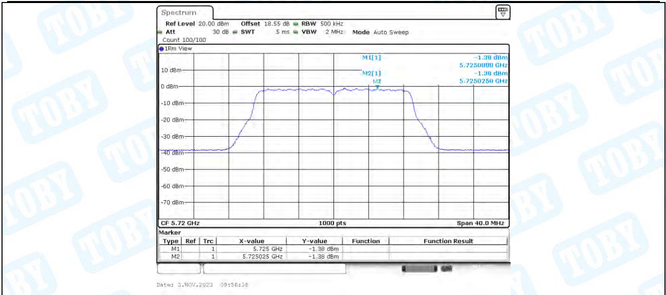
11AC20-CDD_Ant2_5720_UNII-3
