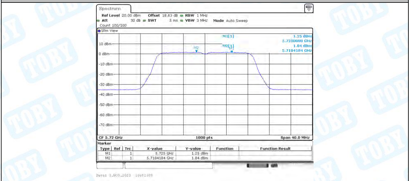
11AC20-CDD_Ant1_5720_UNII-3
