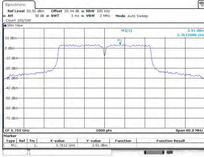
11N40-CDD_Ant2_5755
