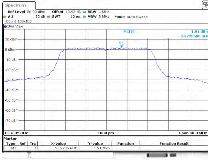
11N20-CDD_Ant2_5320
