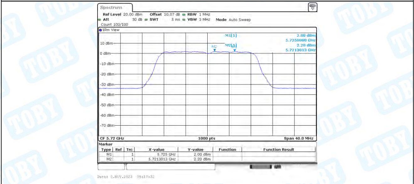
11N20-CDD_Ant3_5720_UNII-2C
