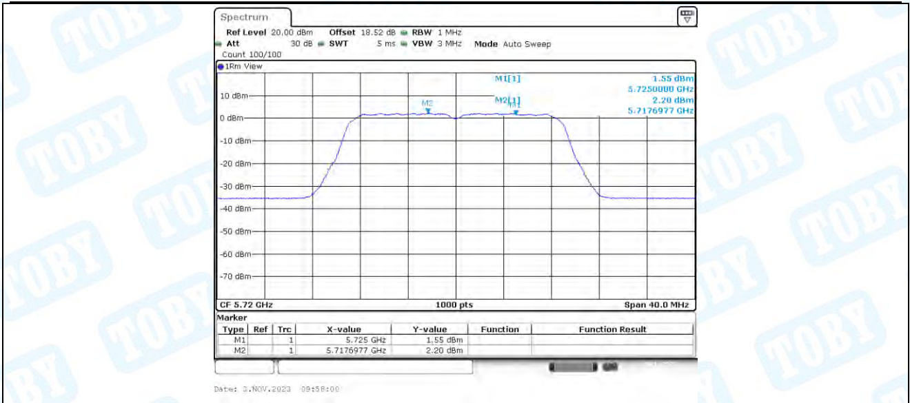
11AC20-CDD_Ant3_5720_UNII-2C
