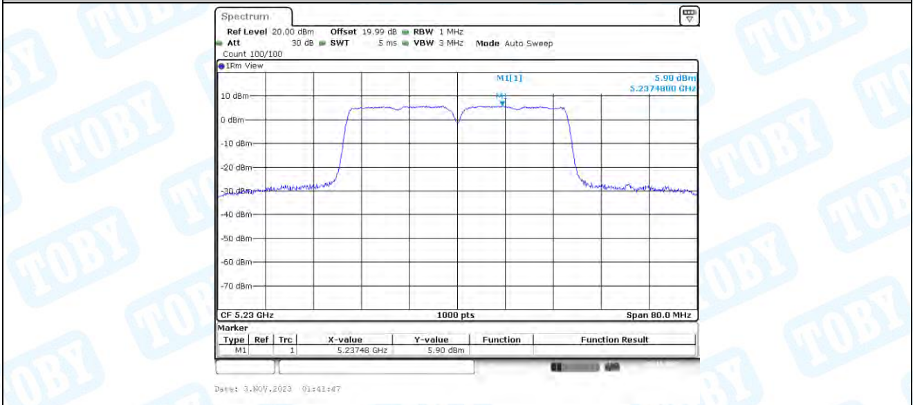
11N40-CDD_Ant3_5230
