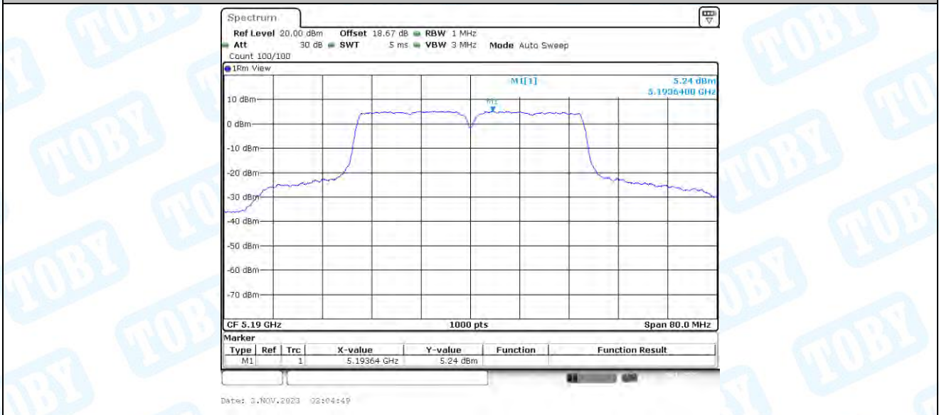
11AC40-CDD_Ant2_5190
