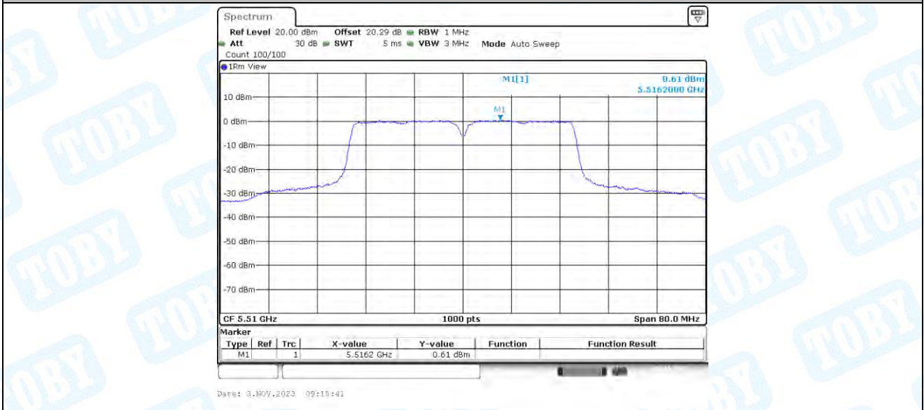
11N40-CDD_Ant3_5510
