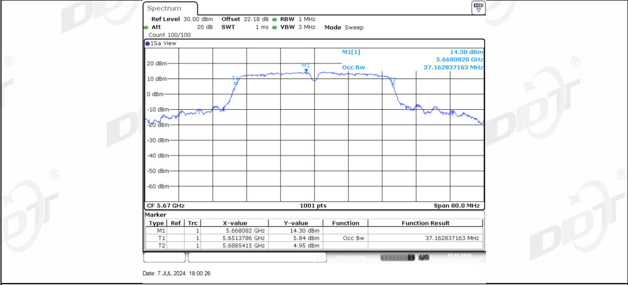
11AC40MIMO_Ant2_5670
