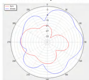
Theta=90 freq=2500MHz
