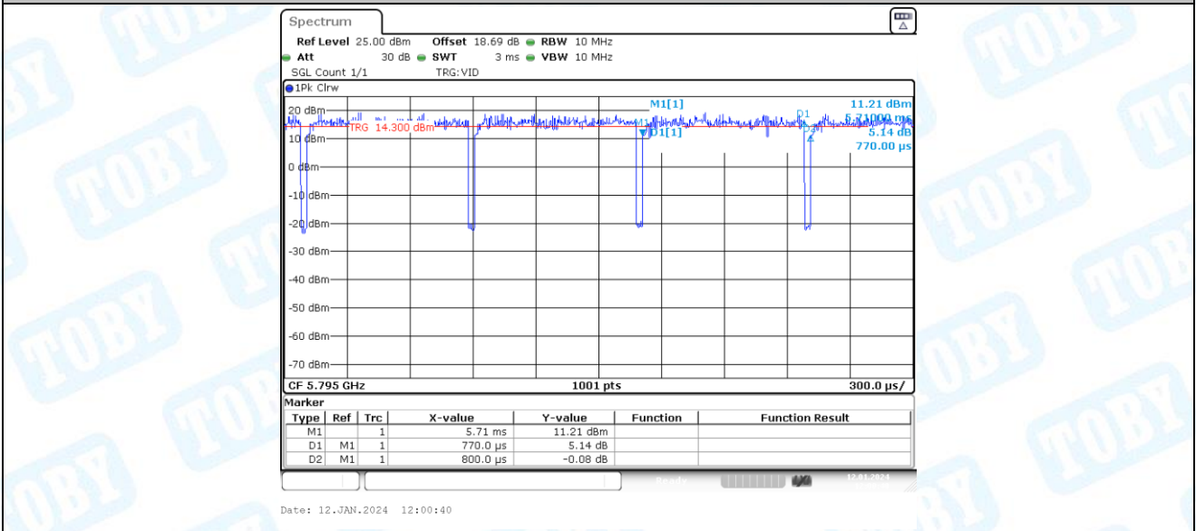
11AX40-CDD_Ant2_5795
