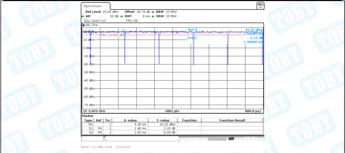
11AX20-CDD_Ant2_5825
