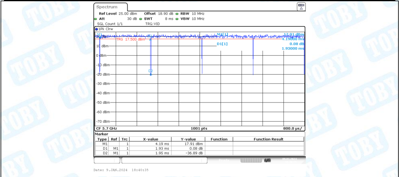
11AC20-CDD_Ant2_5700
