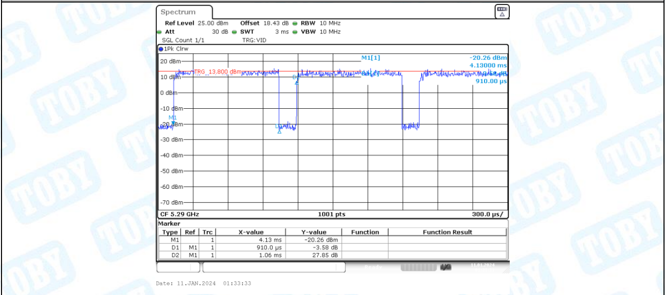
11AC80-CDD_Ant2_5290
