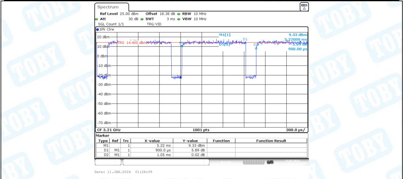
11AC80-CDD_Ant2_5210
