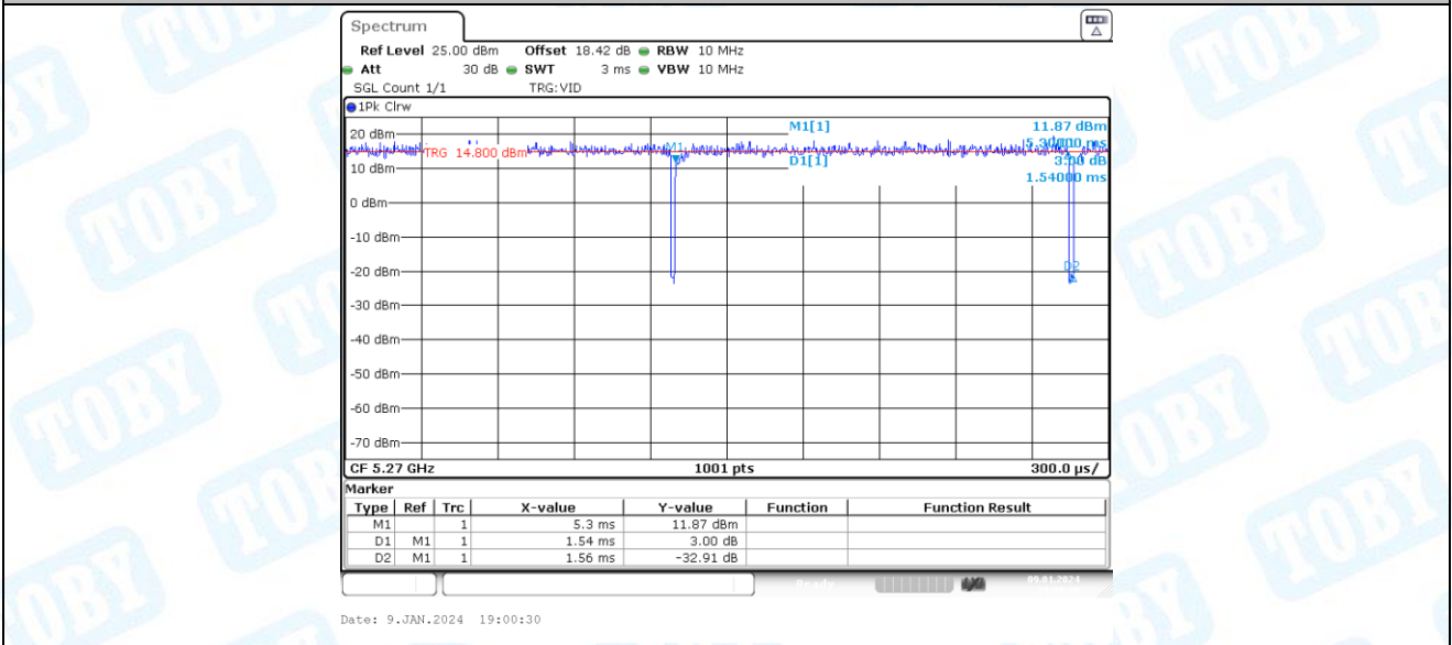
11AC40-CDD_Ant2_5270
