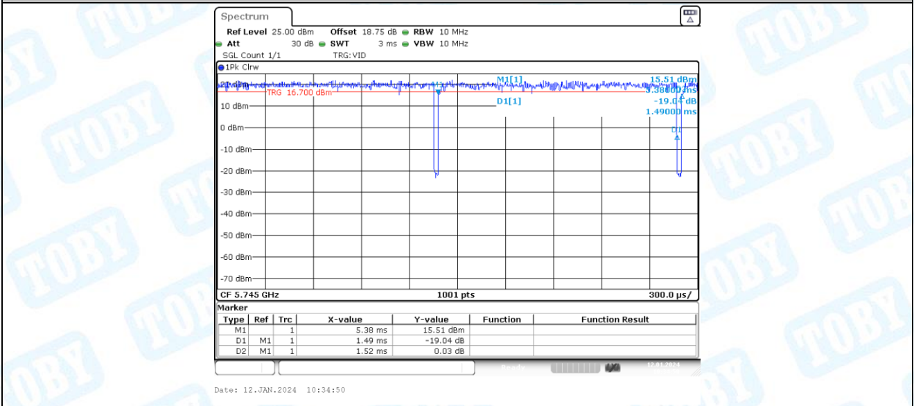
11AX20-CDD_Ant2_5745
