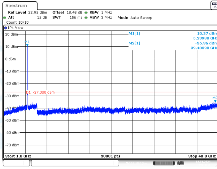
11AX20-CDD_Ant1_5240_1000~40000
