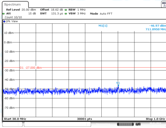
11AC40-CDD_Ant1_5550_30~1000
