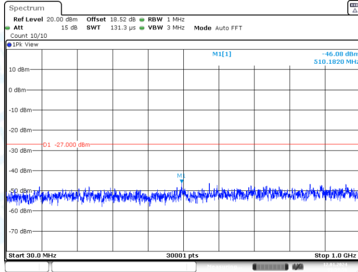
11AX20-CDD_Ant2_5280_30~1000
