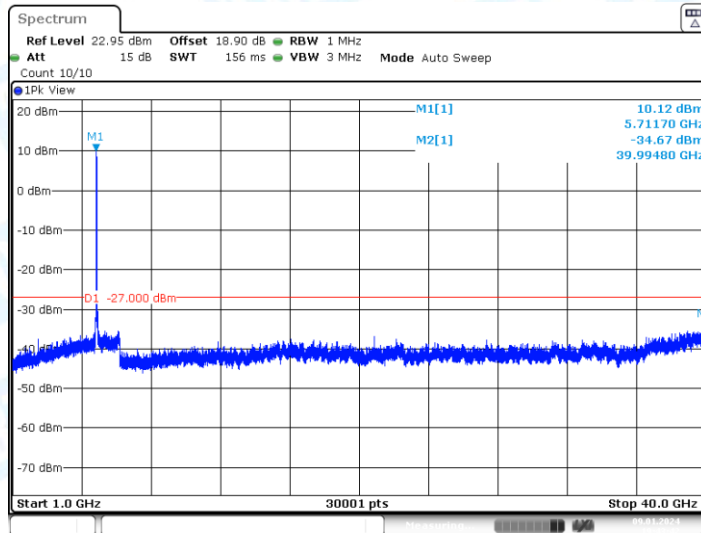
11AC40-CDD_Ant1_5710_1000~40000
