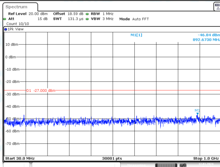
11AX20-CDD_Ant1_5580_30~1000
