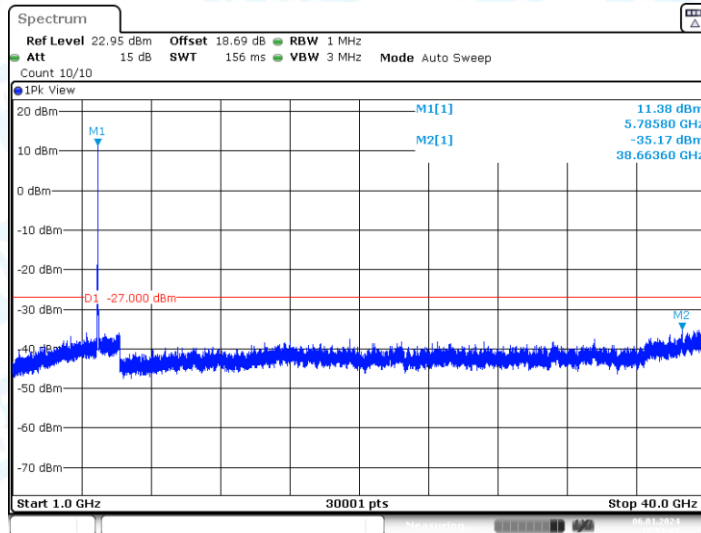
11AC20-CDD_Ant1_5785_1000~40000
