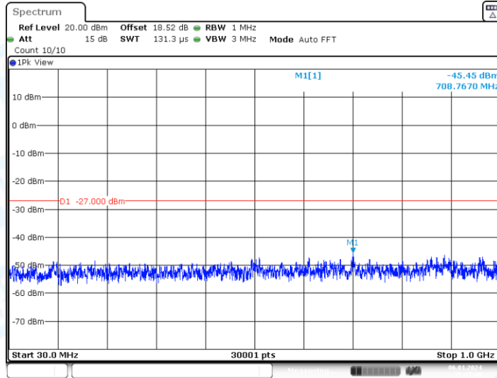
11N40-CDD_Ant2_5270_30~1000
