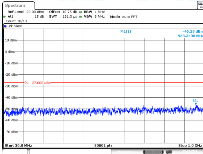
11N40-CDD_Ant2_5755_30~1000
