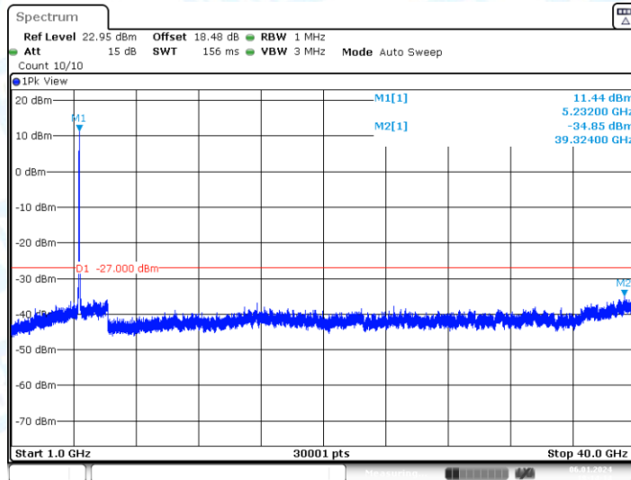
11AC40-CDD_Ant1_5230_1000~40000
