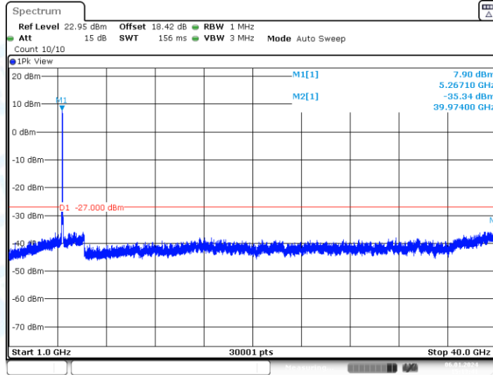
11N40-CDD_Ant1_5270_1000~40000
