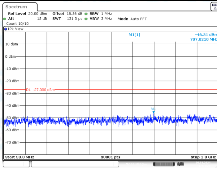
11AC20-CDD_Ant1_5500_30~1000
