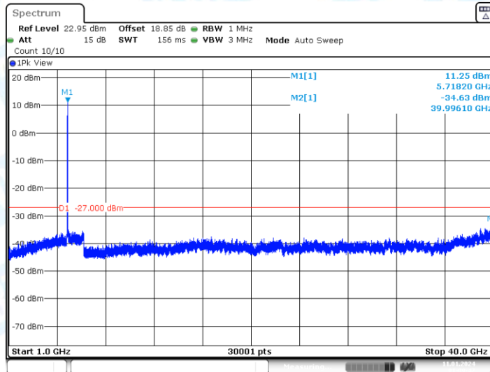
11AC20-CDD_Ant2_5720_1000~40000
