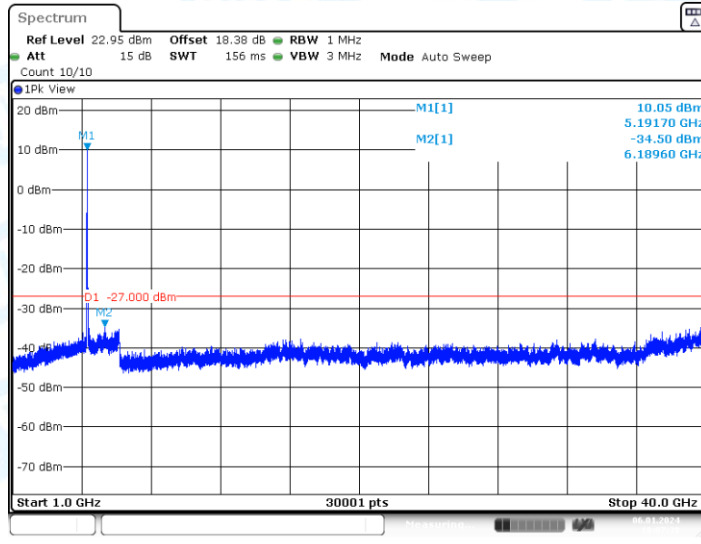
11AC40-CDD_Ant1_5190_1000~40000
