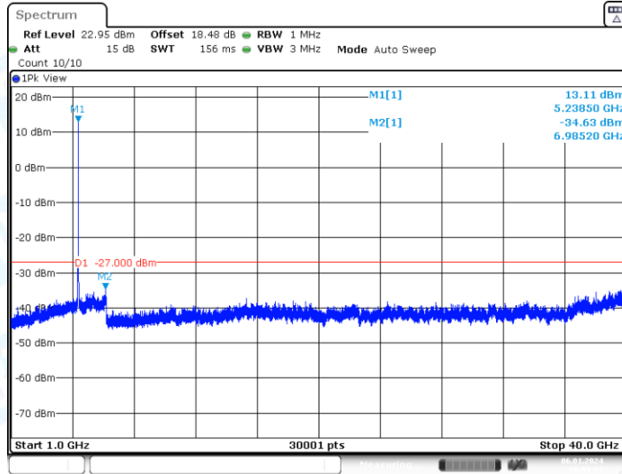
11AC20-CDD_Ant1_5240_1000~40000
