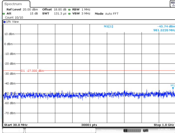
11AC20-CDD_Ant2_5720_30~1000
