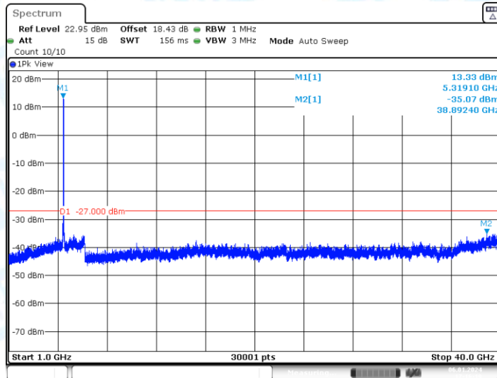
11AC20-CDD_Ant1_5320_1000~40000
