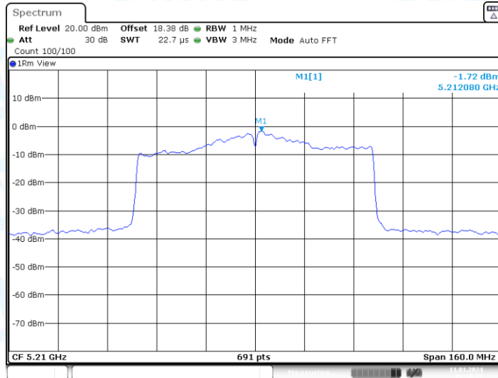
11AC80-CDD_Ant2_5210
