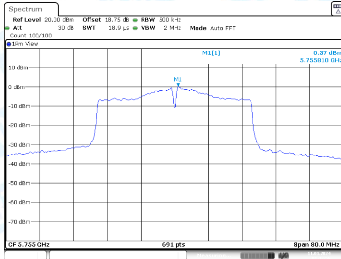
11AC40-CDD_Ant1_5755
