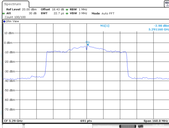
11AC80-CDD_Ant1_5290
