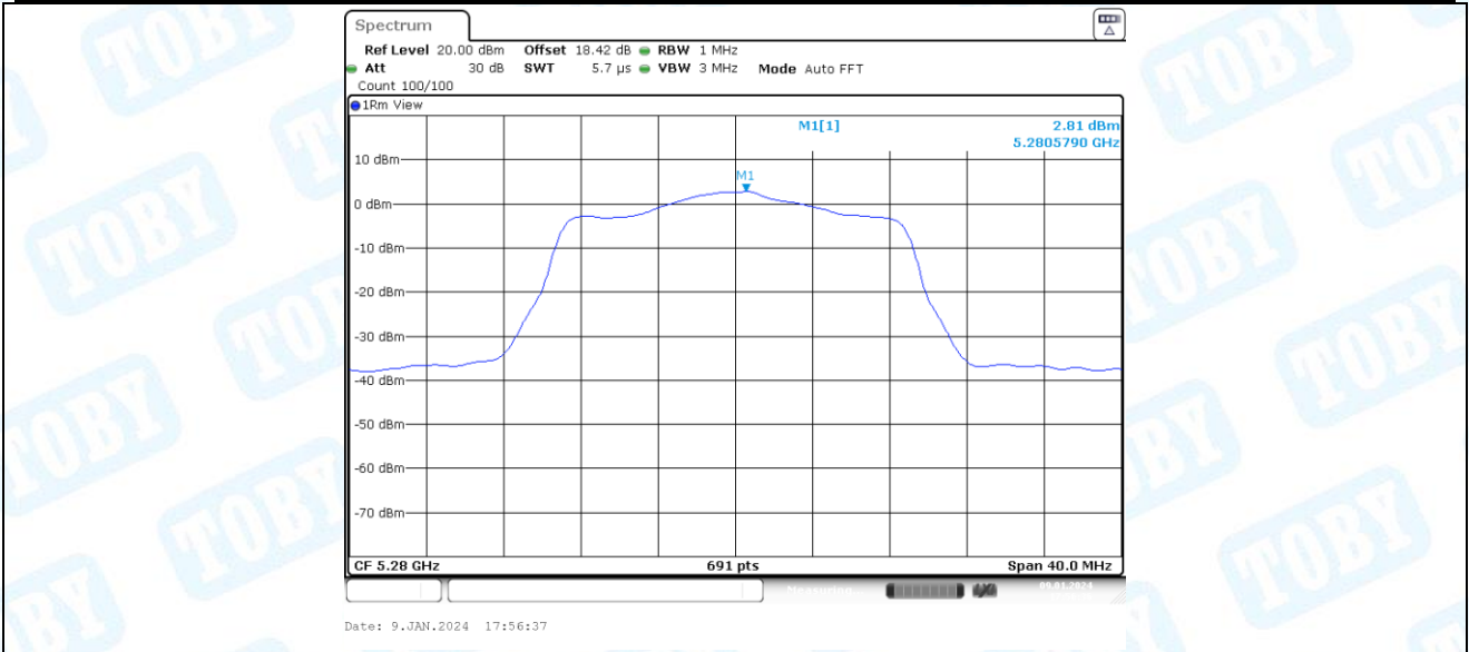
11AC20-CDD_Ant2_5280
