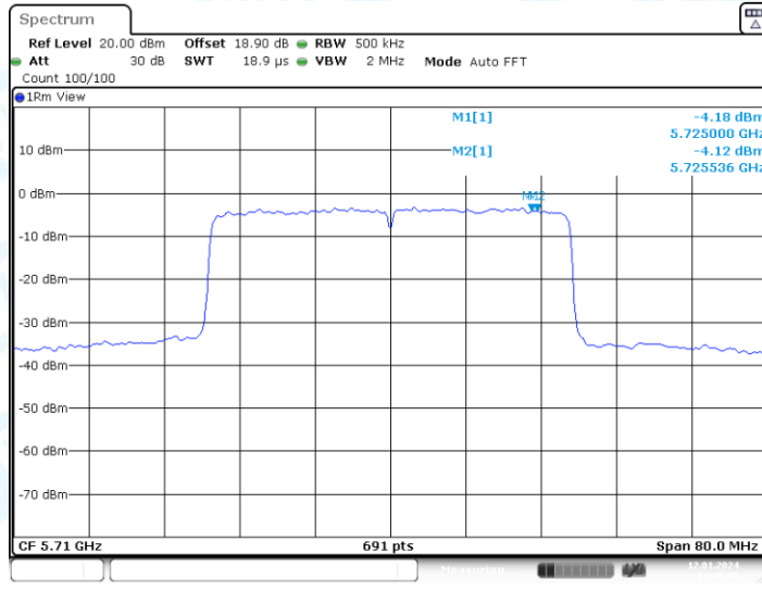
11AX40-CDD_Ant1_5710_UNII-3
