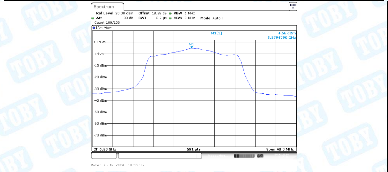
11AC20-CDD_Ant2_5580
