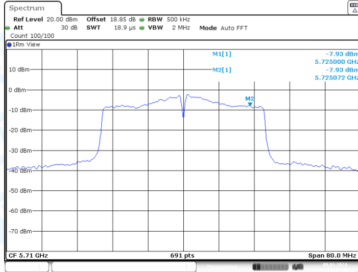
11AC40-CDD_Ant2_5710_UNII-3
