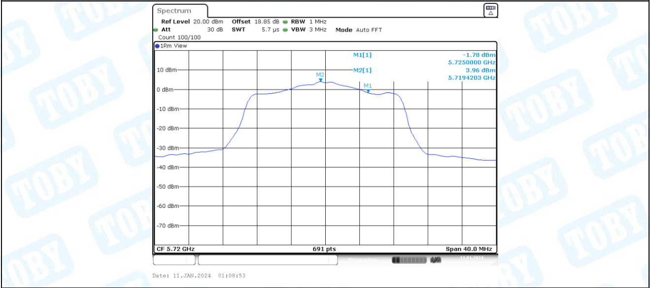
11AC20-CDD_Ant1_5720_UNII-3
