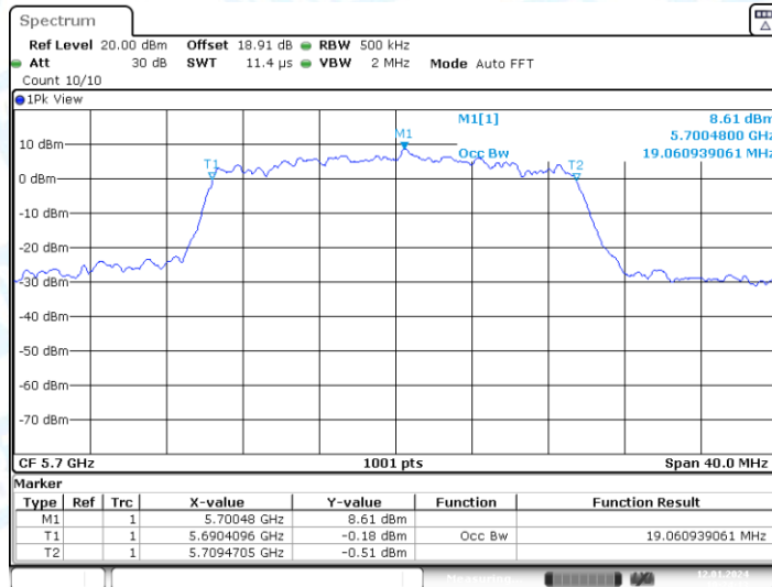
11AX20-CDD_Ant2_5700
