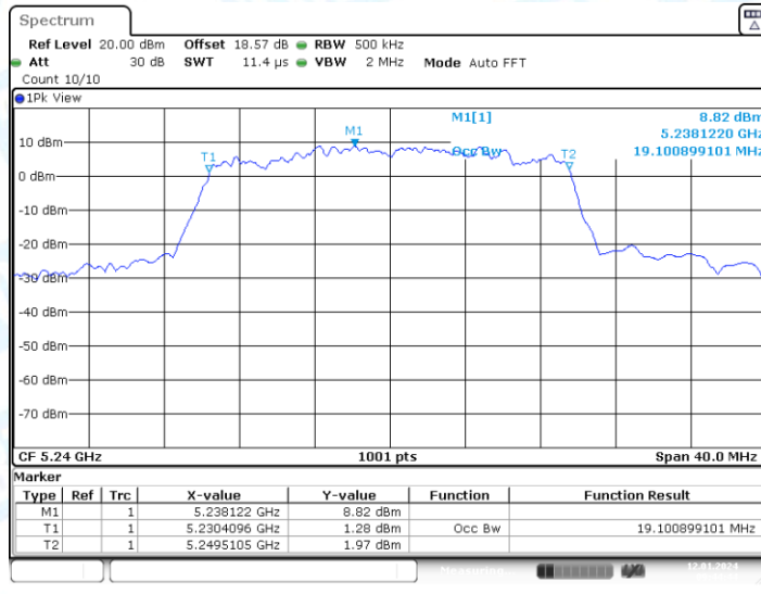
11AX20-CDD_Ant2_5240
