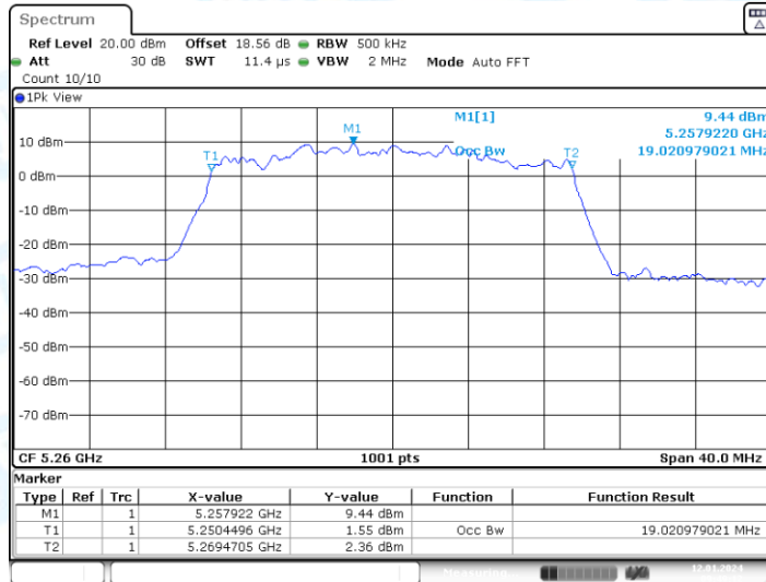
11AX20-CDD_Ant2_5260
