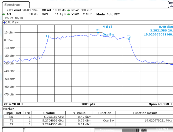
11AX20-CDD_Ant1_5280
