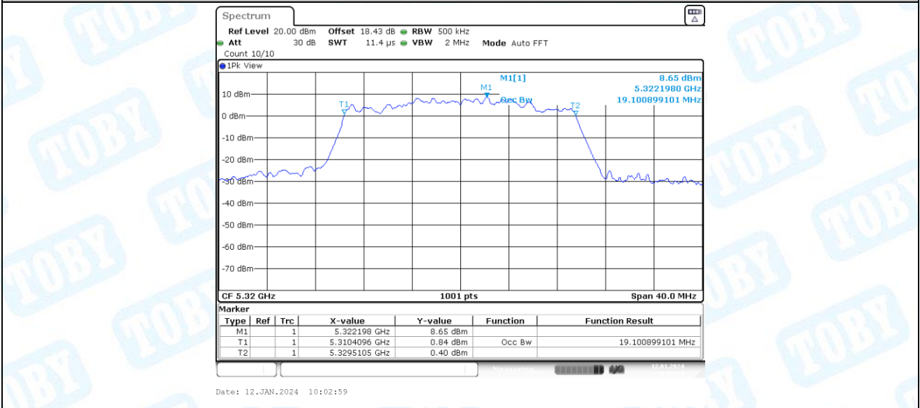
11AX20-CDD_Ant2_5320
