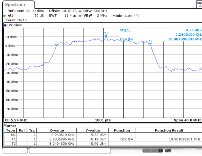
11AX20-CDD_Ant1_5240
