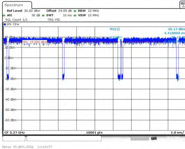
11AX40-BF_Ant2_5270
