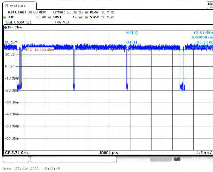
11N40-BF_Ant2_5710
