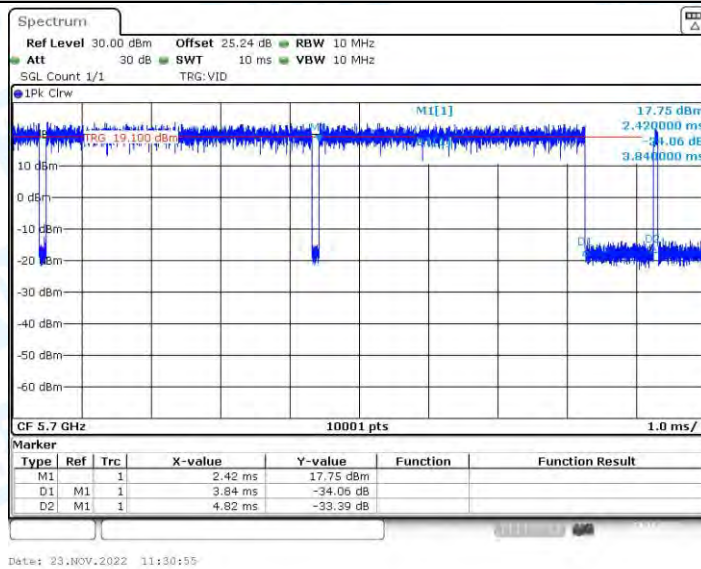
11N20-BF_Ant1_5720
