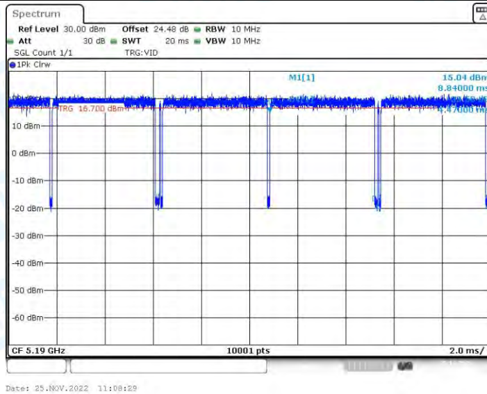
11AX40-BF_Ant2_5190
