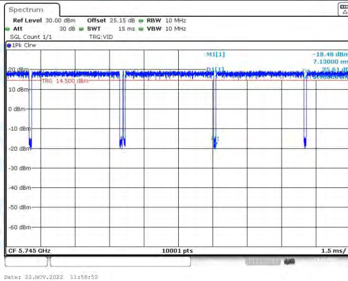
11N20-BF_Ant2_5745
