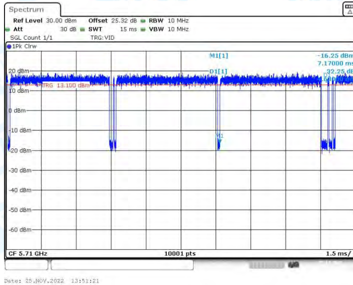
11AX40-BF_Ant2_5710
