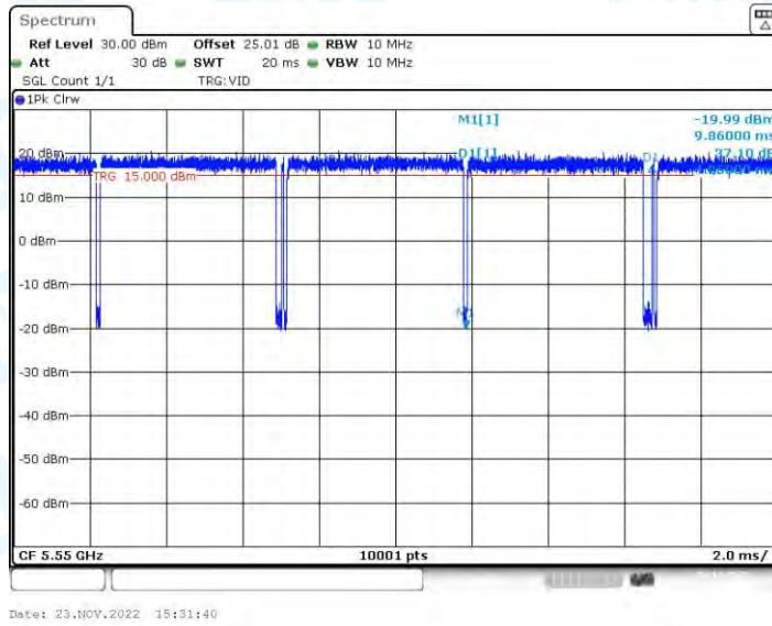
11N40-BF_Ant2_5550
