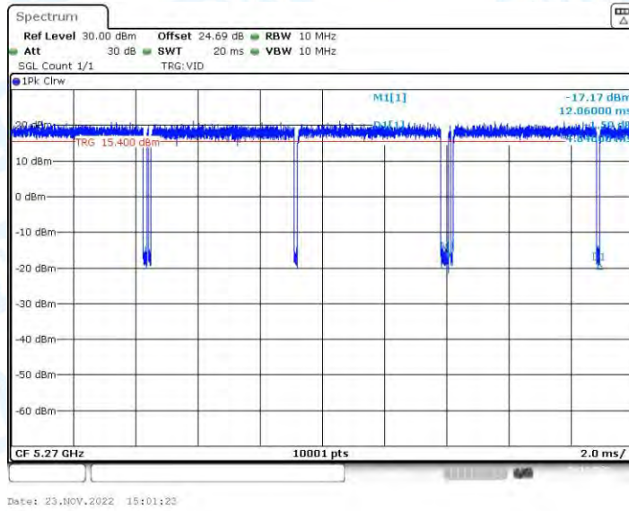
11N40-BF_Ant2_5270
