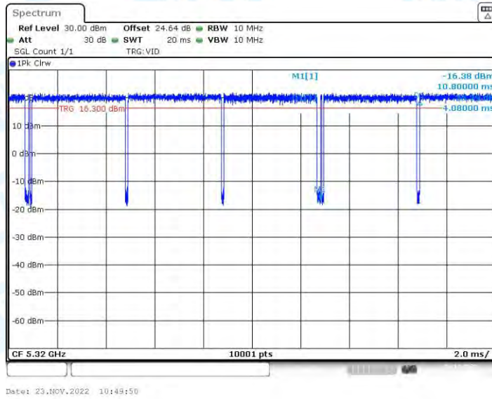
11N20-BF_Ant2_5320
