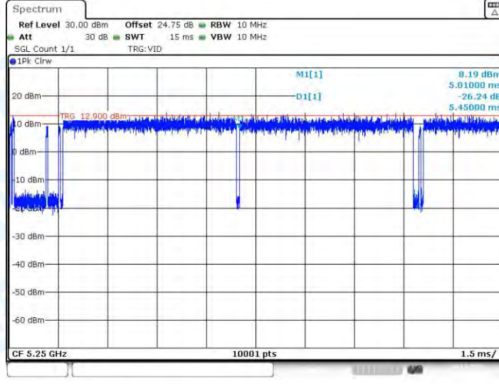
11AC160-BF_Ant1_5250
