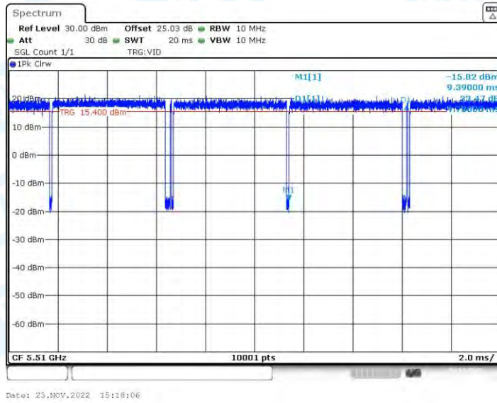
11N40-BF_Ant2_5510
