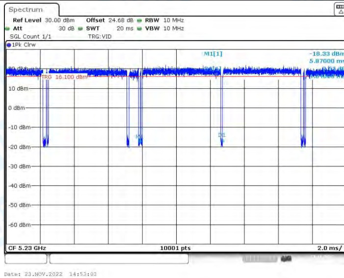
11AC40-BF_Ant2_5230
