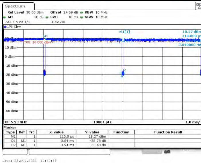
11N20-BF_Ant2_5280
