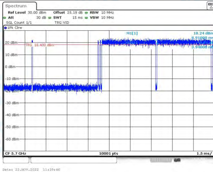
11AC20-BF_Ant2_5700
