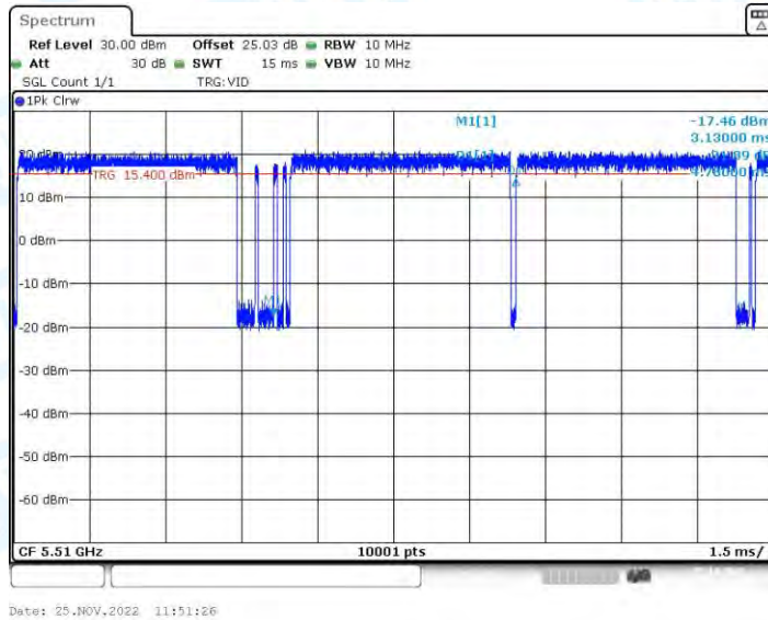
11AX40-BF_Ant2_5510
