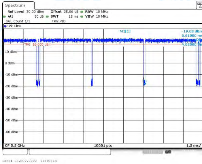
11N20-BF_Ant2_5500
