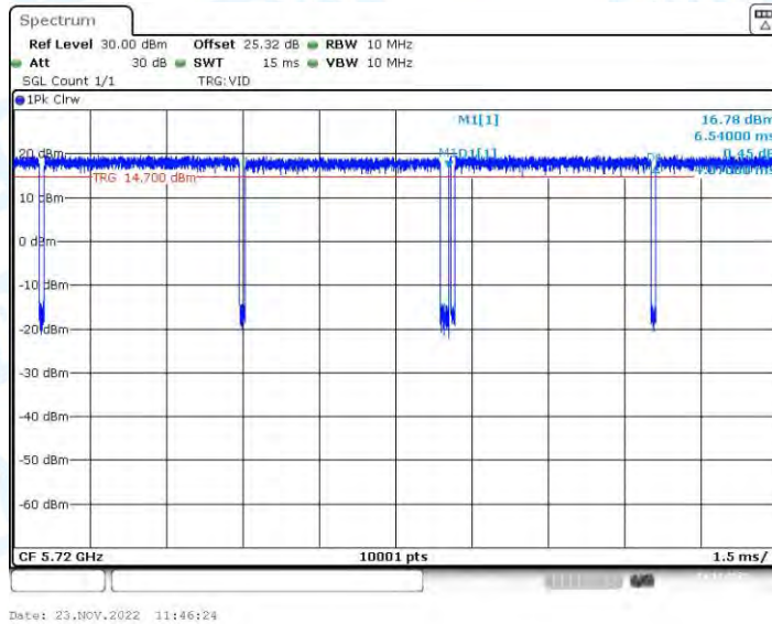
11N20-BF_Ant2_5720
