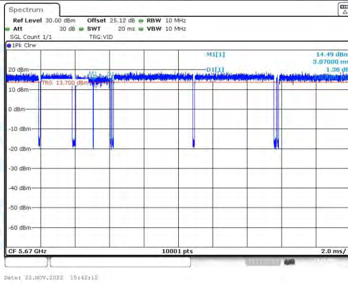
11N40-BF_Ant2_5670
