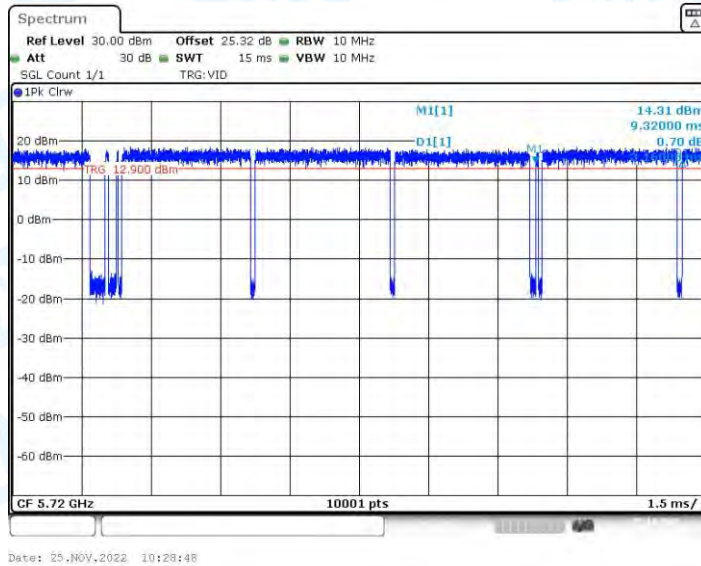
11AX20-BF_Ant2_5720
