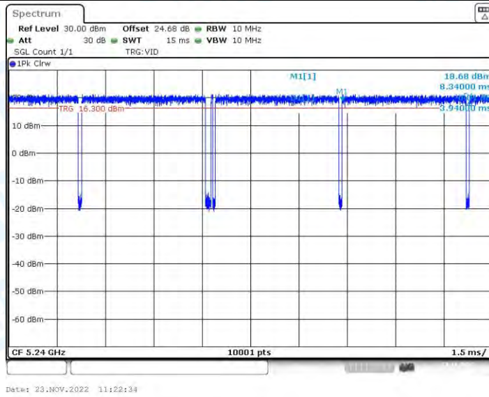
11AC20-BF_Ant2_5240
