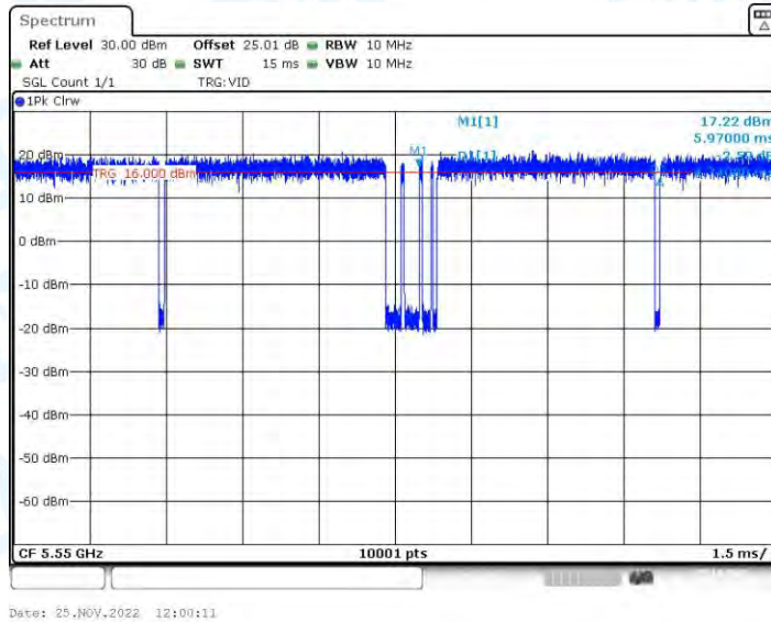
11AX40-BF_Ant2_5550
