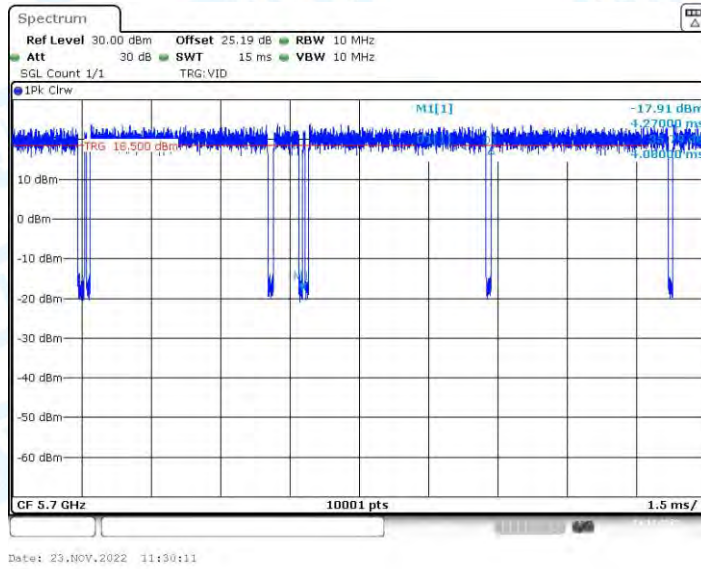
11N20-BF_Ant2_5700
