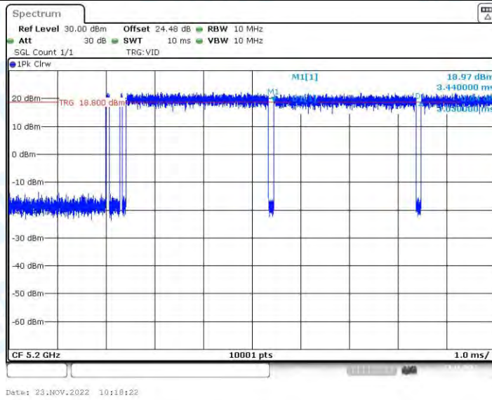
11AX20-BF_Ant2_5200
