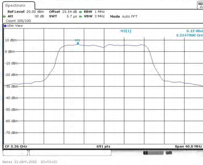
11AC20-CDD_Ant2_5260
