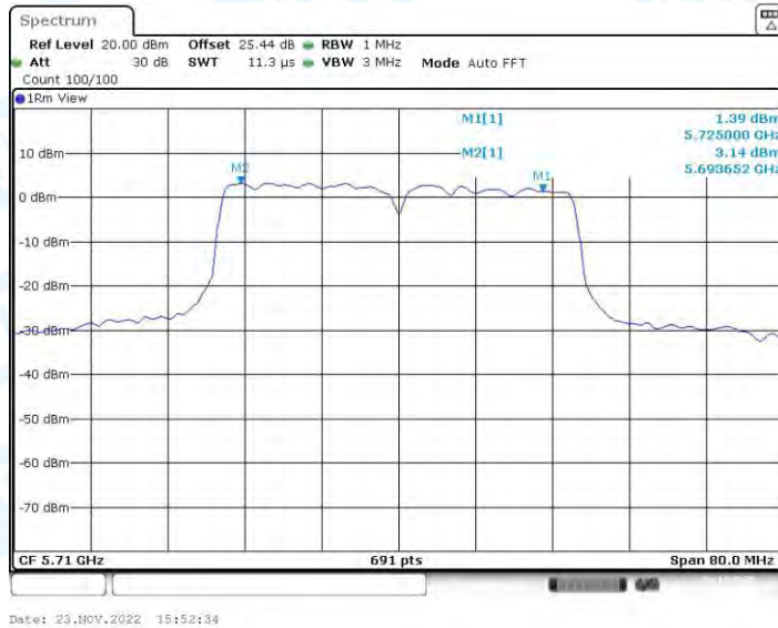
11N40-BF_Ant1_5710_UNII-3
