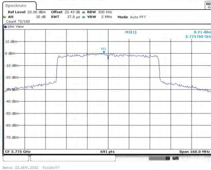
11AX80-CDD_Ant2_5775
