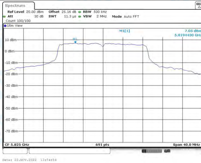
11N20-BF_Ant2_5825
