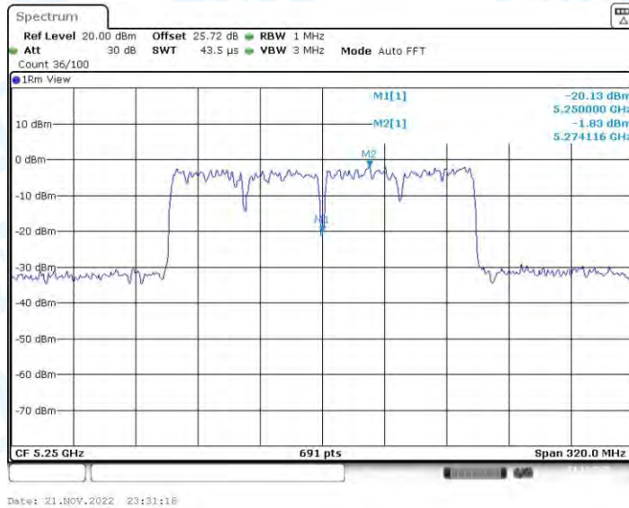
11AC160-CDD_Ant2_5250_UNII-2A
