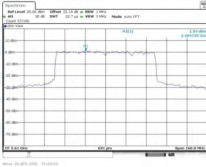
11AX80-CDD_Ant2_5610
