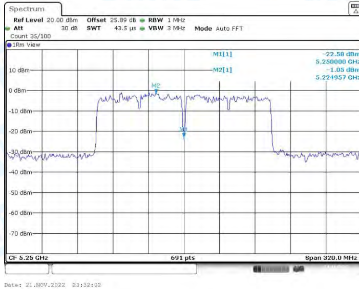
11AC160-CDD_Ant1_5250_UNII-2A
