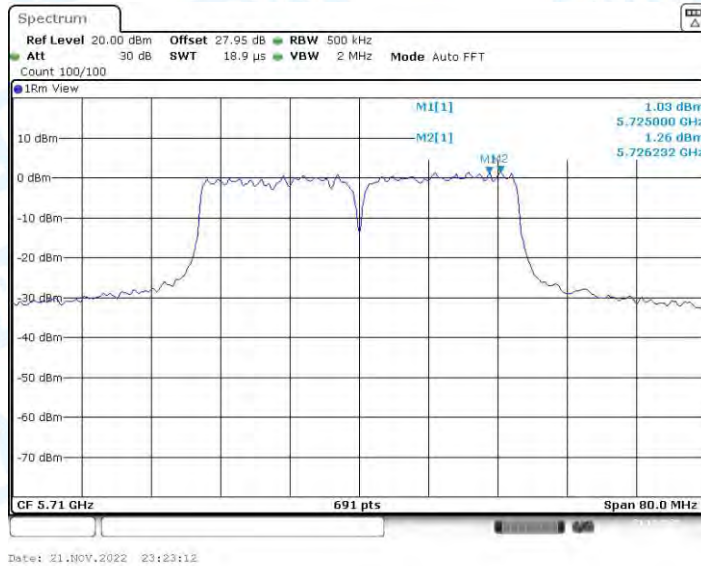
11N40-CDD_Ant2_5710_UNII-3
