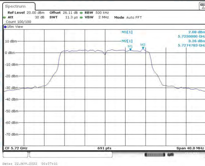
11AC20-CDD_Ant2_5720_UNII-3
