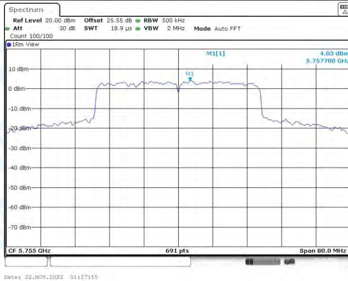
11AX40-CDD_Ant2_5755
