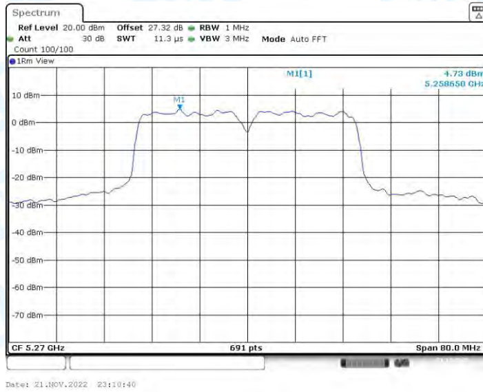
11N40-CDD_Ant2_5270
