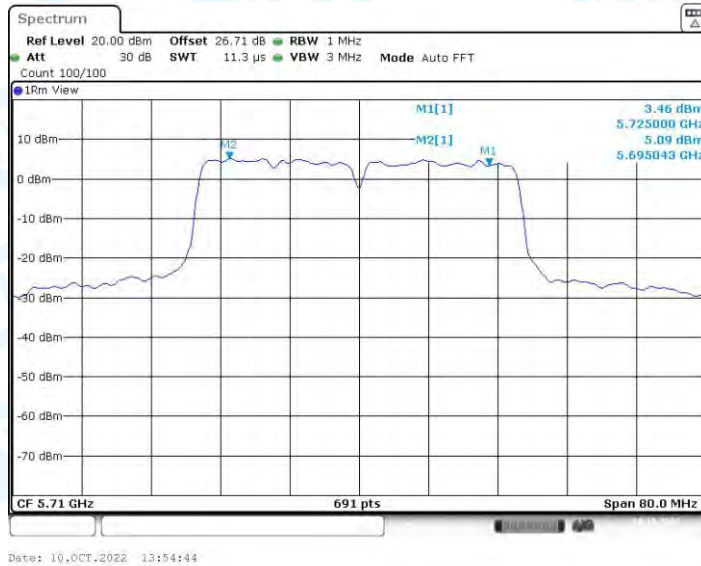
11AC40-SDM_Ant1_5710_UNII-3
