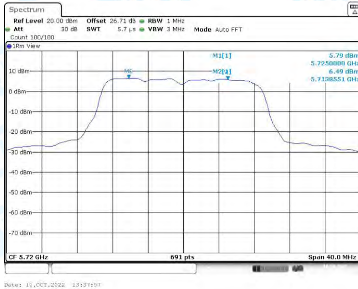
11AC20-SDM_Ant1_5720_UNII-3
