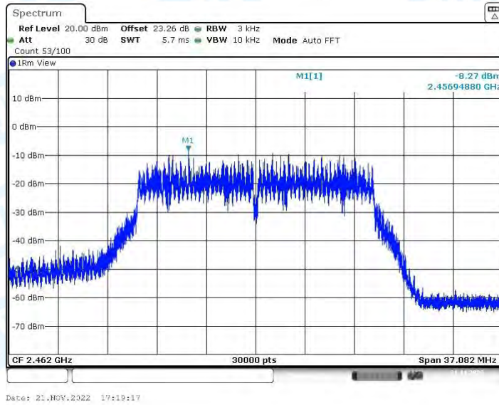
VHT20-CDD_Ant2_2462
