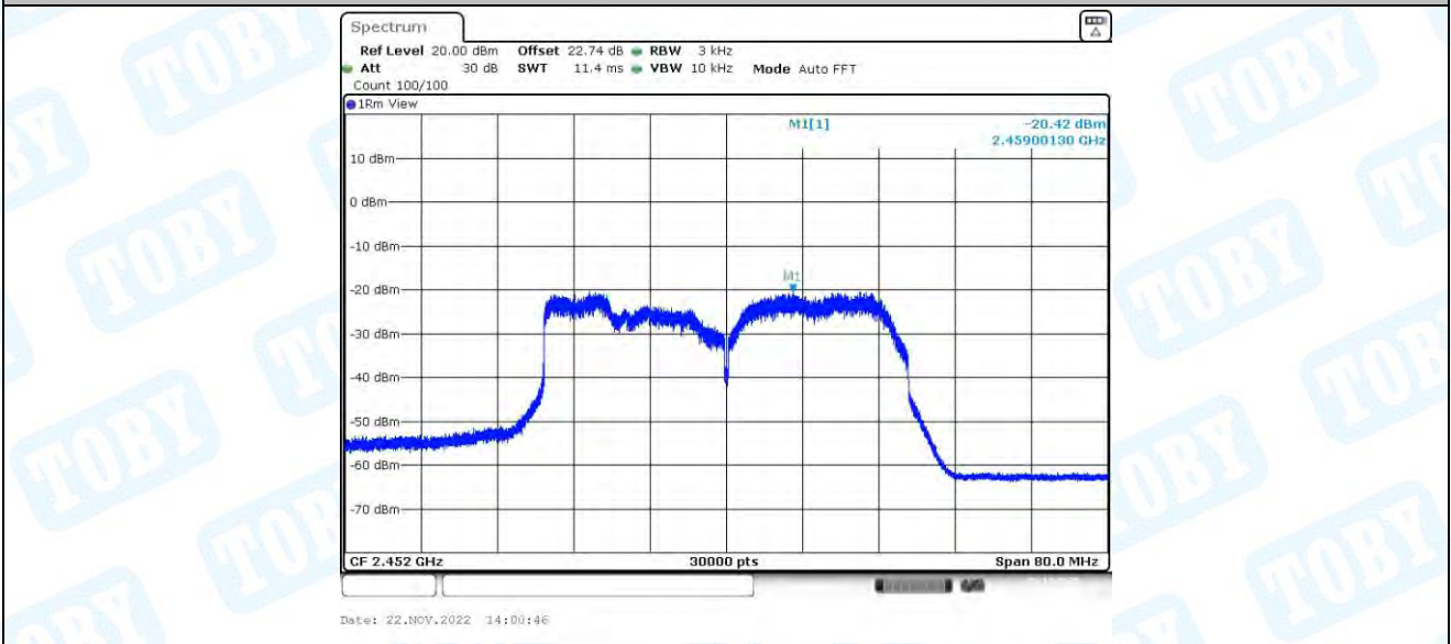
11AX40-BF_Ant2_2452
