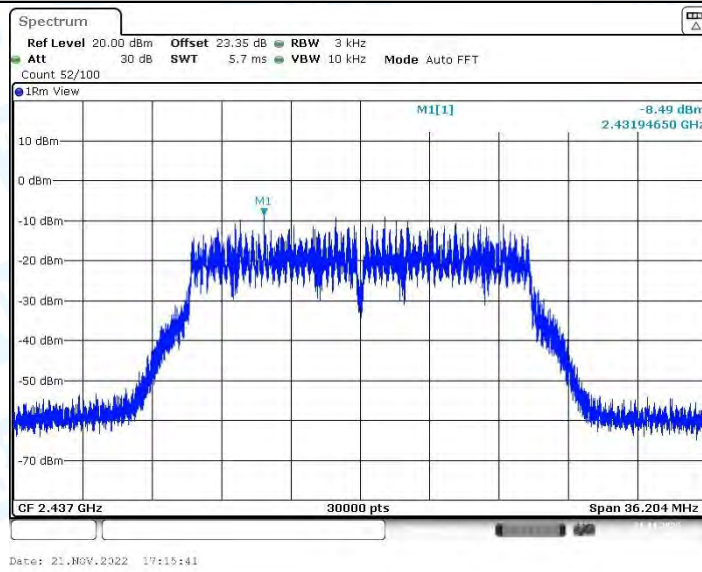
VHT20-CDD_Ant2_2437
