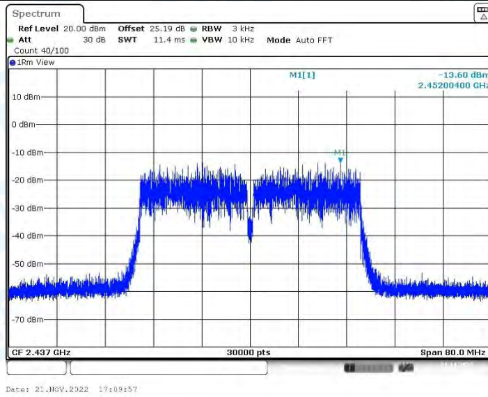
11N40-CDD_Ant2_2437
