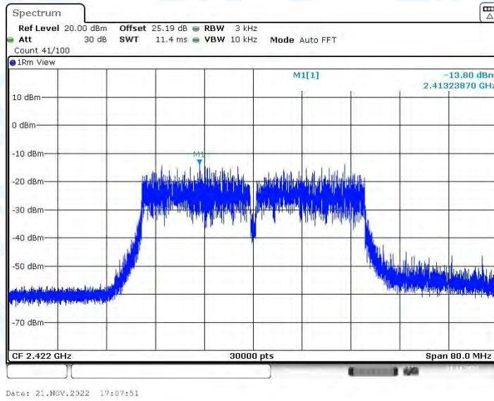
11N40-CDD_Ant2_2422
