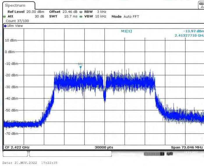
VHT40-CDD_Ant2_2422
