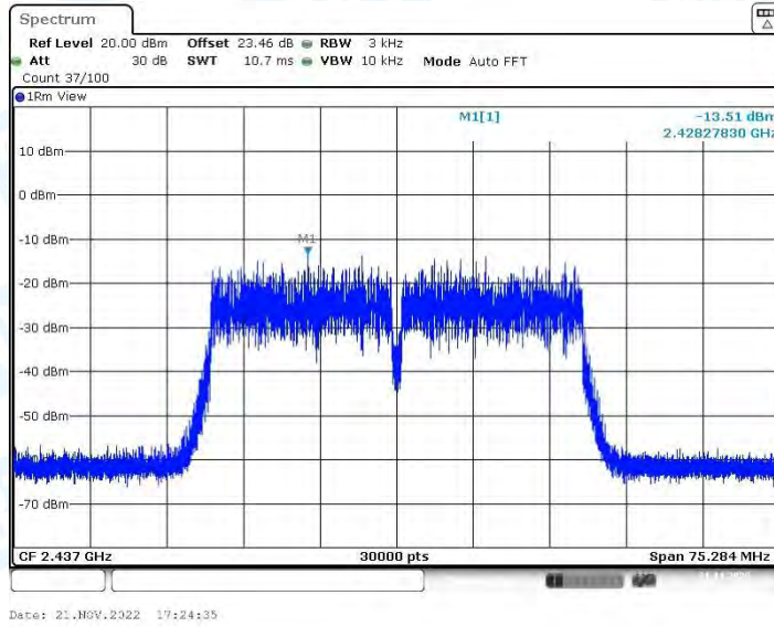
VHT40-CDD_Ant2_2437
