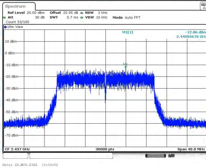
11AX20-CDD_Ant2_2437
