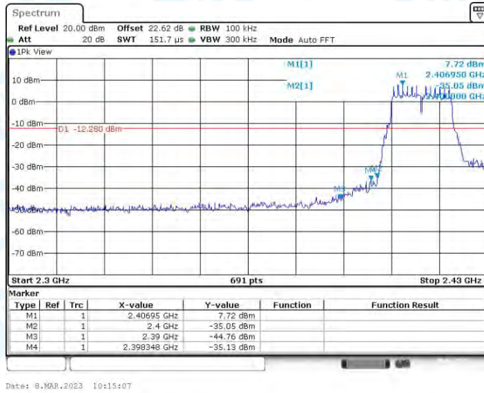
11G-SISO_Ant2_Low_2412
