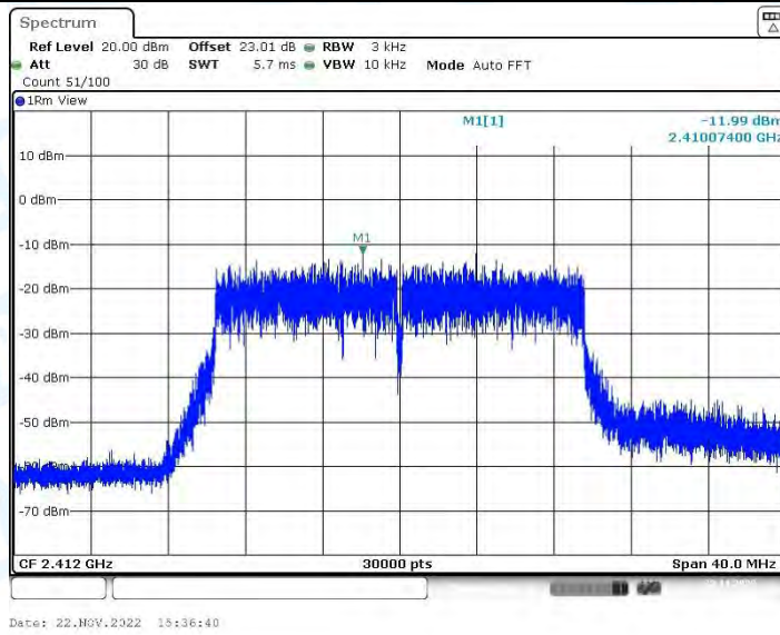
11AX20-CDD_Ant2_2412
