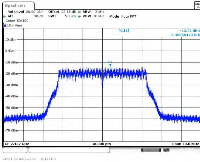
VHT20-BF_Ant2_2437
