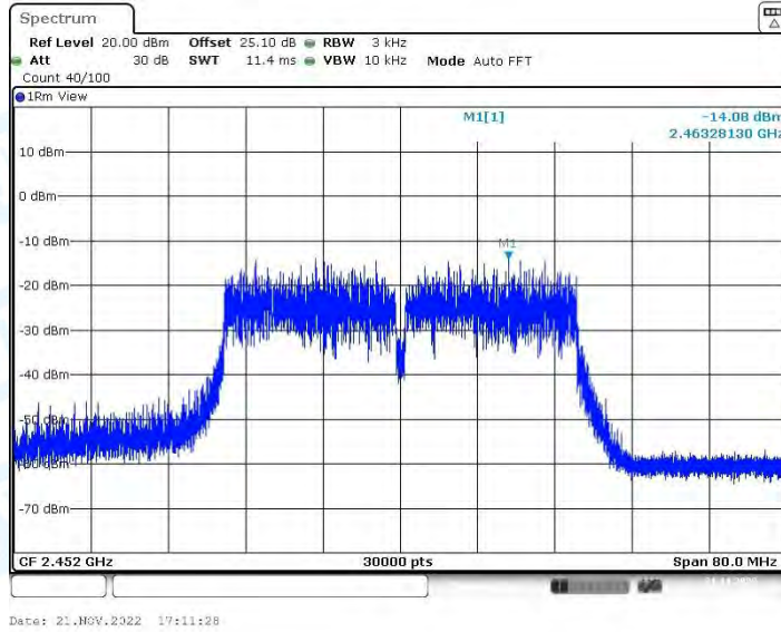
11N40-CDD_Ant2_2452
