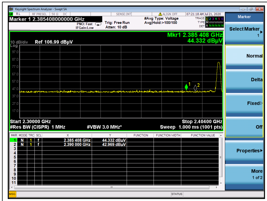
(AVERAGE,Channel = 0,GFSK)
