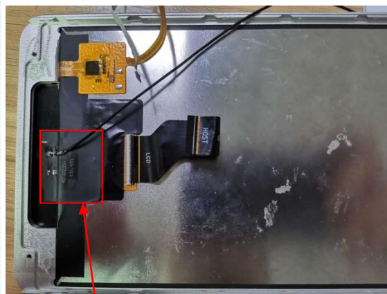
Antenna
