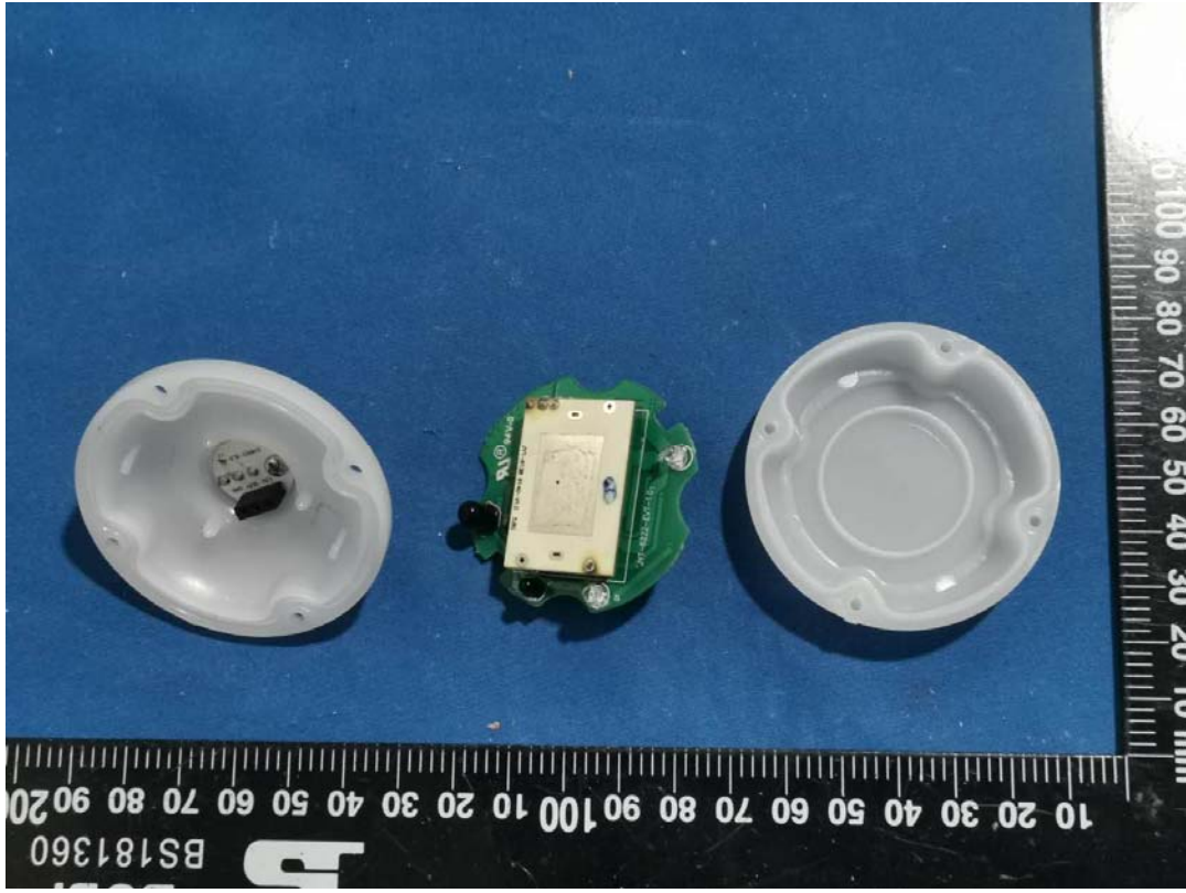
RF module
