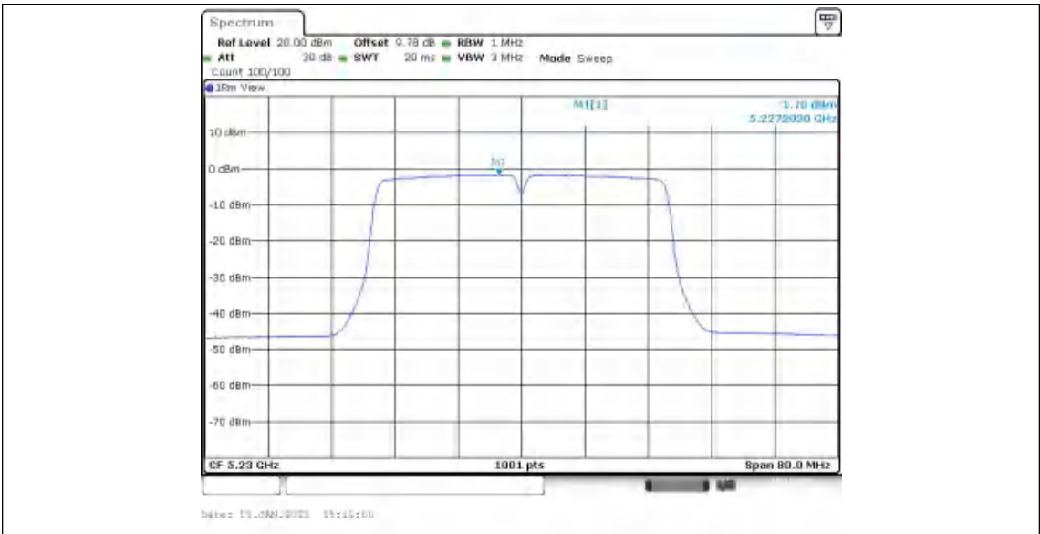
11N40MIMO_Ant2_5230
