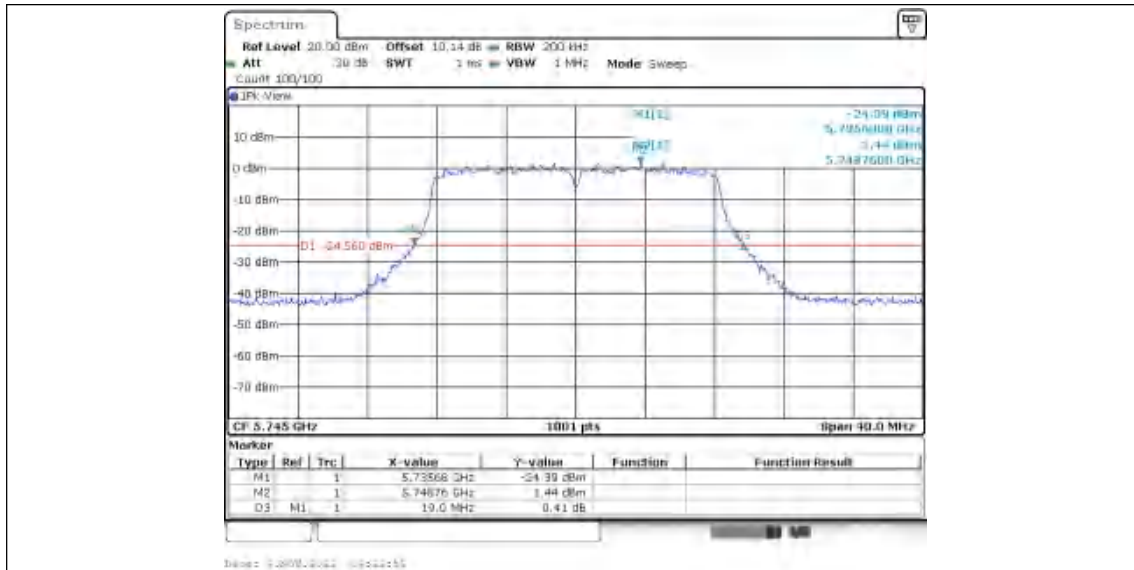
11A-CDD_Ant2_5745
