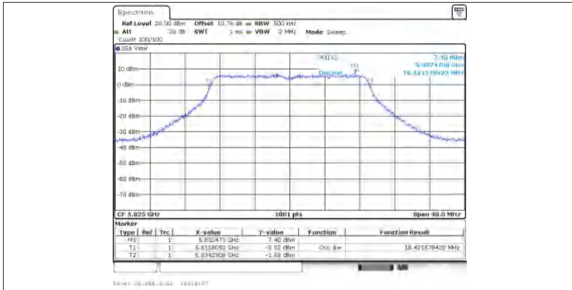
11N20MIMO_Ant2_5825
