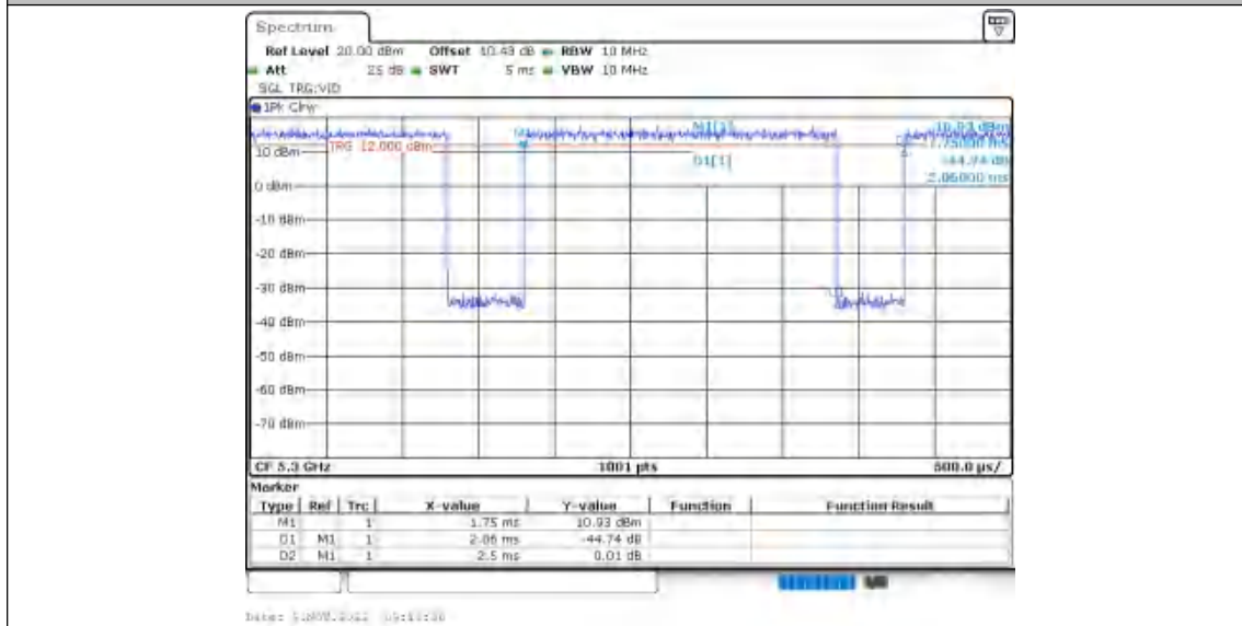
11A-CDD_Ant1_5320
