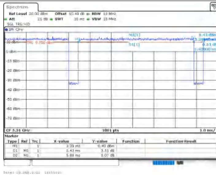
11N40MIMO_Ant2_5310
