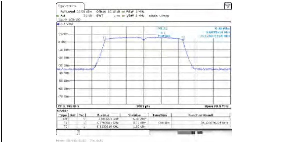
11N40MIMO_Ant2_5795
