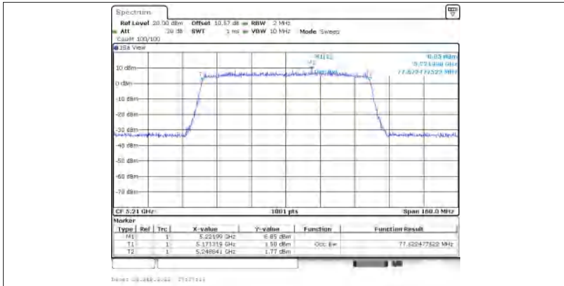
11AX80MIMO_Ant2_5210
