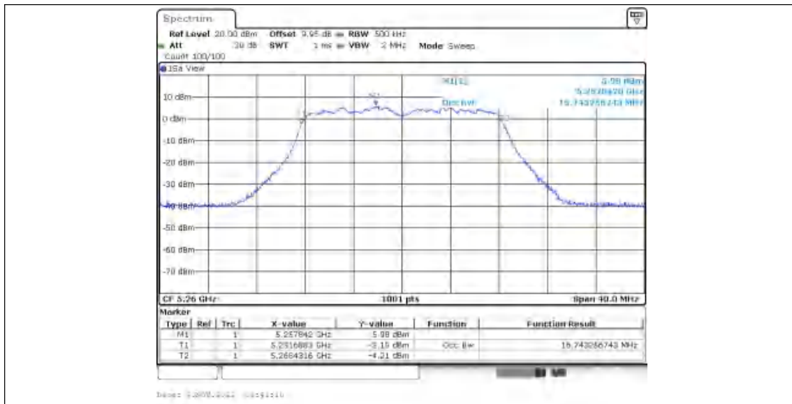
11A-CDD_Ant2_5260
