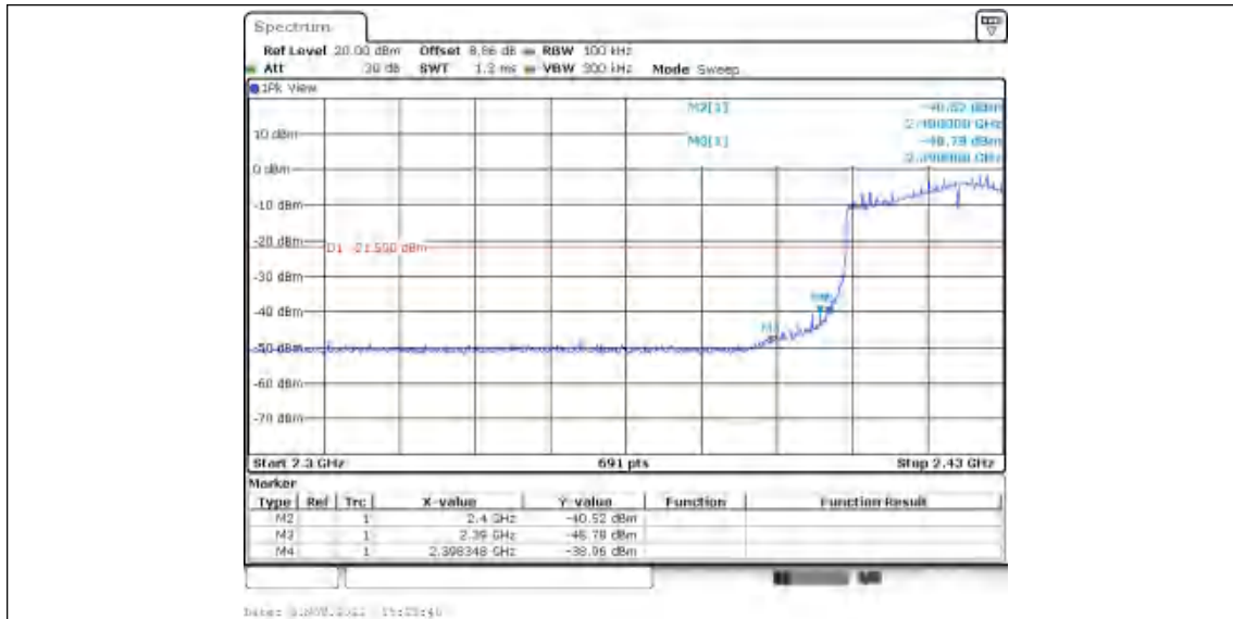
11AX40MIMO_Ant2_Low_2422
