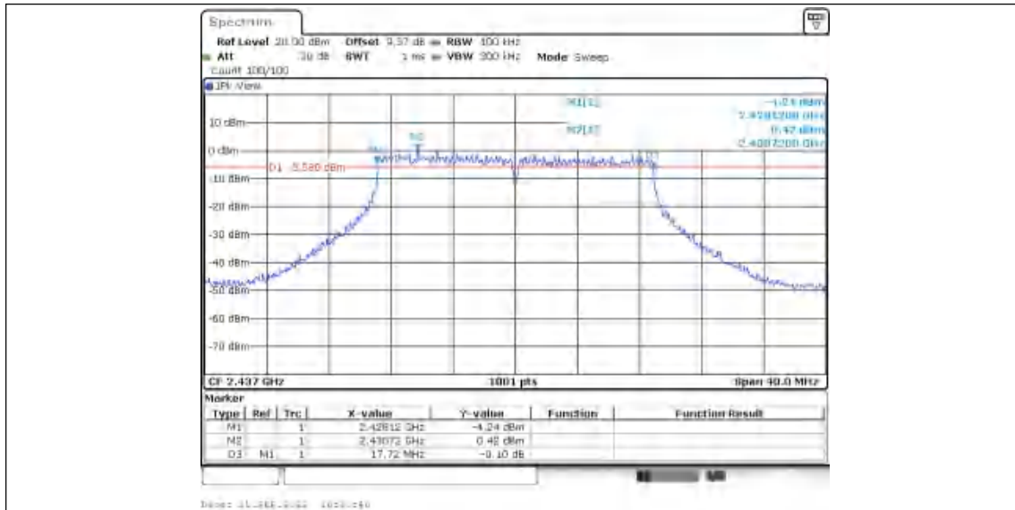
11N20MIMO_Ant2_2437
