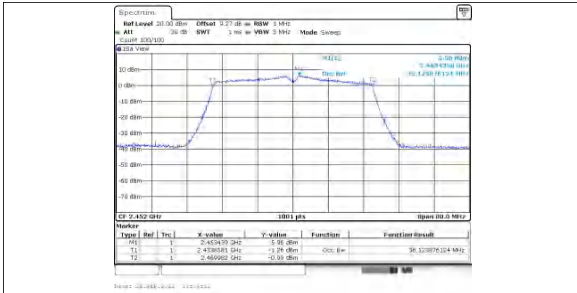
11N40MIMO_Ant2_2452
