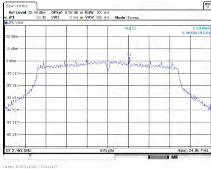
11G-CDD_Ant2_2462
