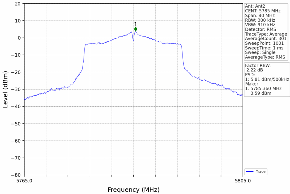
802.11n(HT20)_MCH_5785MHz_MIMO_NTNV
