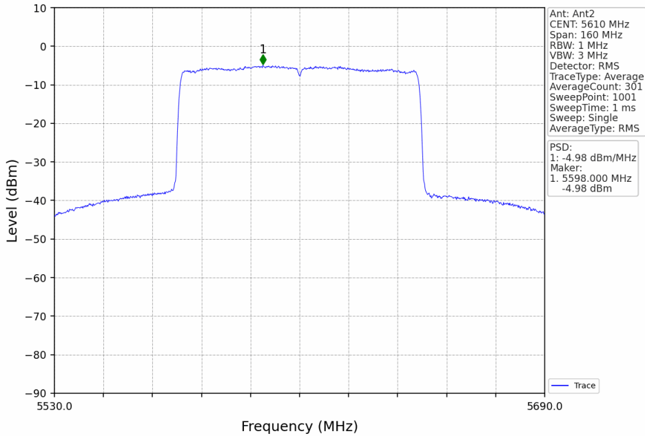
802.11ax(HEW80)_HCH_5610MHz_RU996_Left_MIMO_NTNV
