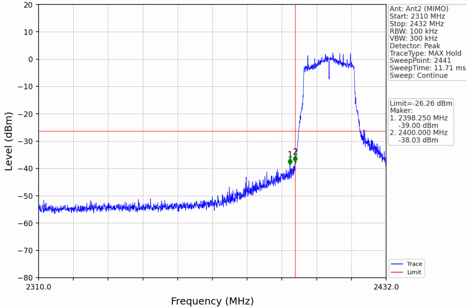
802.11n(HT20)_LCH_2412MHz_Ant2 (MIMO)_NTNV
