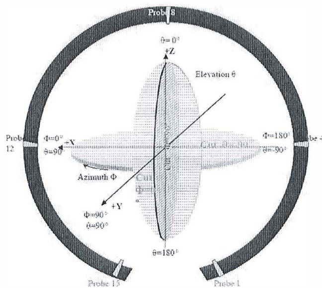
图 1 3D 微波暗室测试坐标系 (back view)
