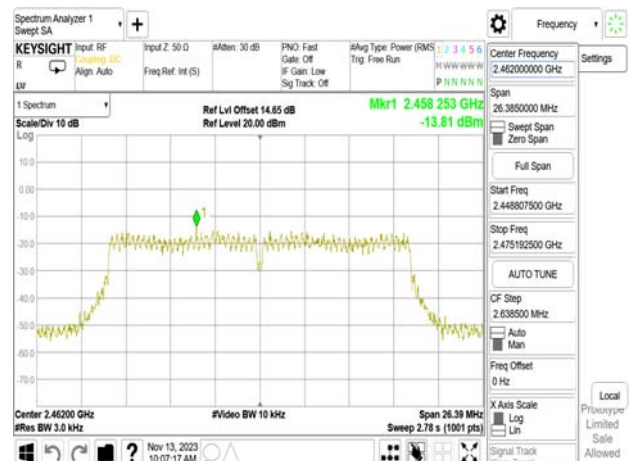
802.11n_20MHz_WLAN2_2462MHz
