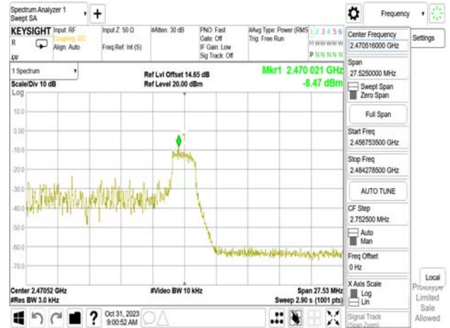
802.11ax_20MHz_WLAN2_2462MHz_RU52_40
