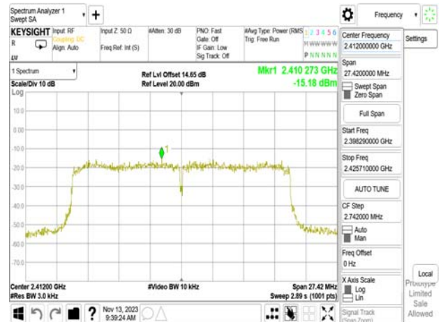
802.11ax_20MHz_WLAN2_2412MHz_RU26_0
