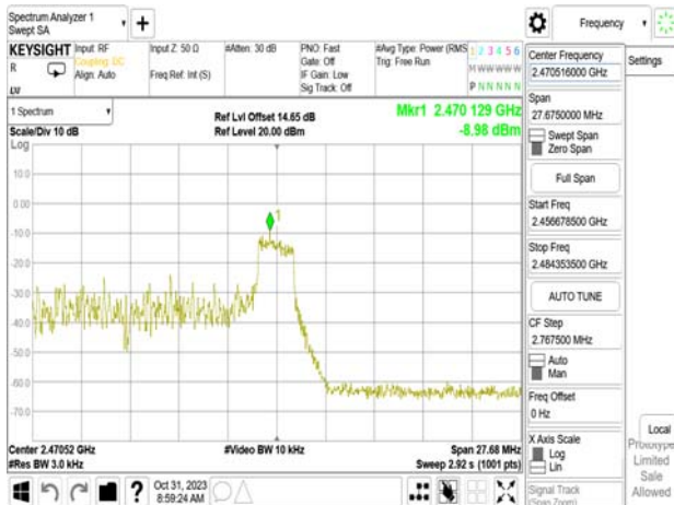
802.11ax_20MHz_WLAN1_2462MHz_RU52_40
