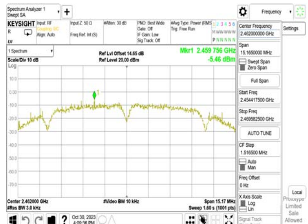
802.11b_20MHz_WLAN2_2462MHz
