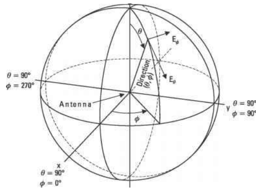
Antenna Coordinates
