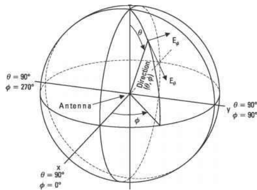
Antenna Coordinates
