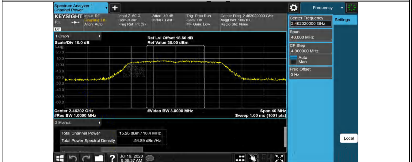
11N20MIMO Ant2 2462
