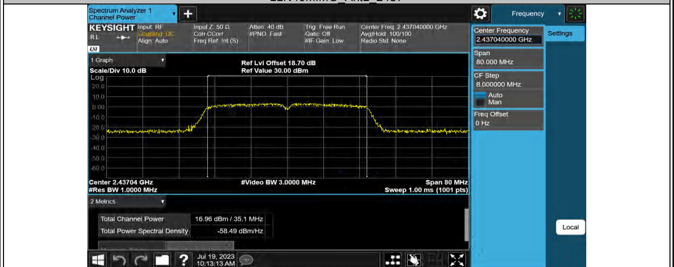
11N40MIMO Ant2 2437
