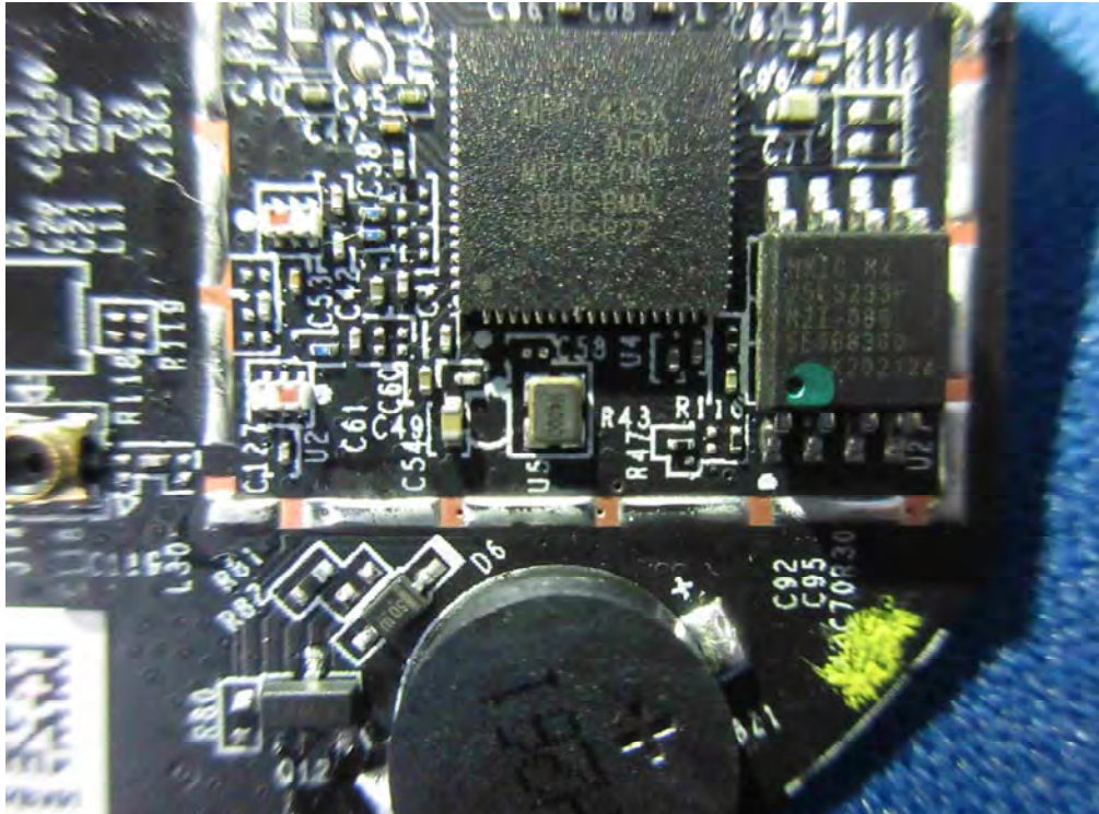
(12) EUT Photo
