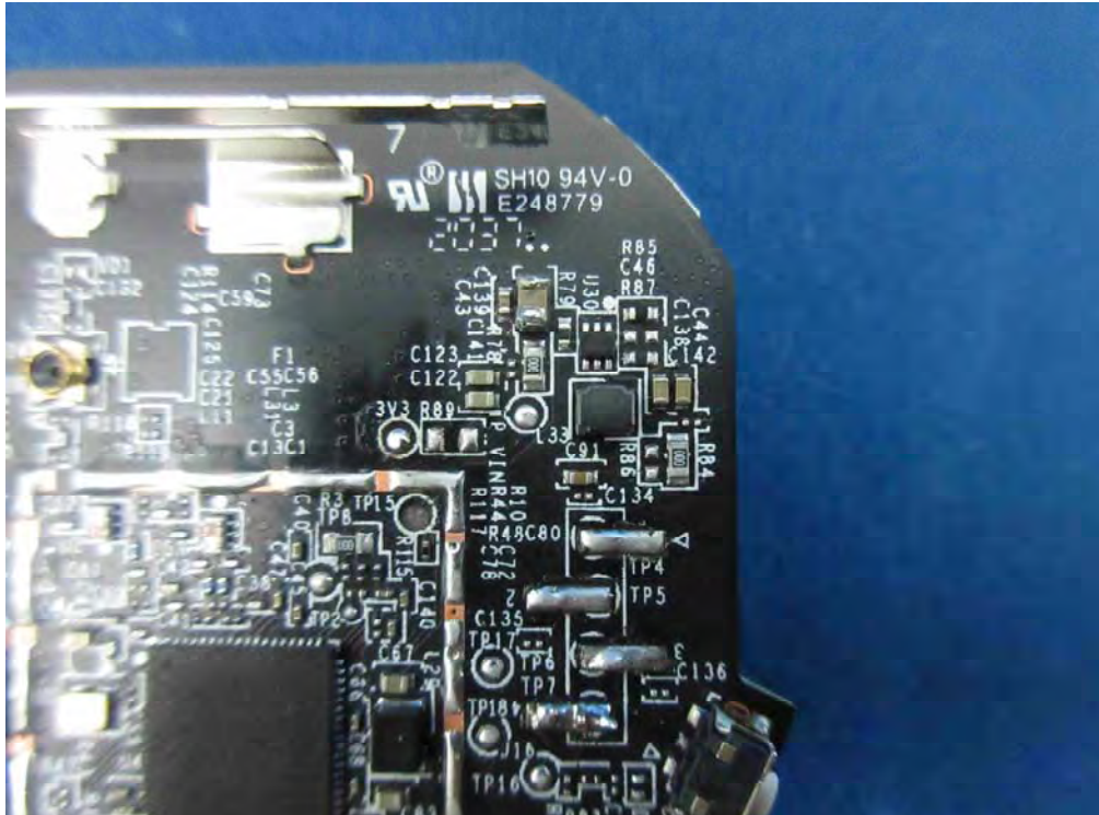
(10) EUT Photo
