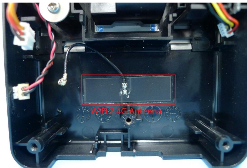
(4) EUT Photo
