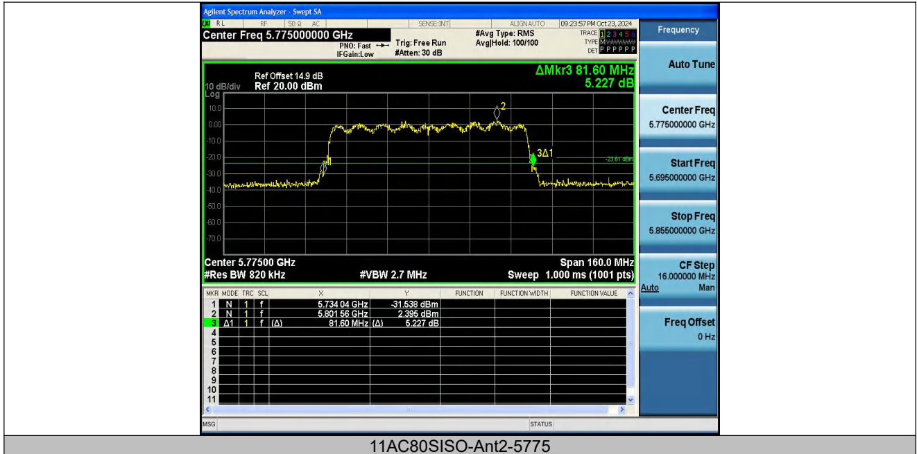
11AC80SISO-Ant2-5775
