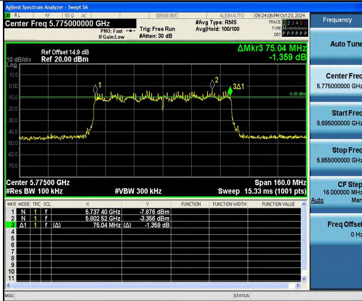
11AC80SISO-Ant2-5775-PASS
