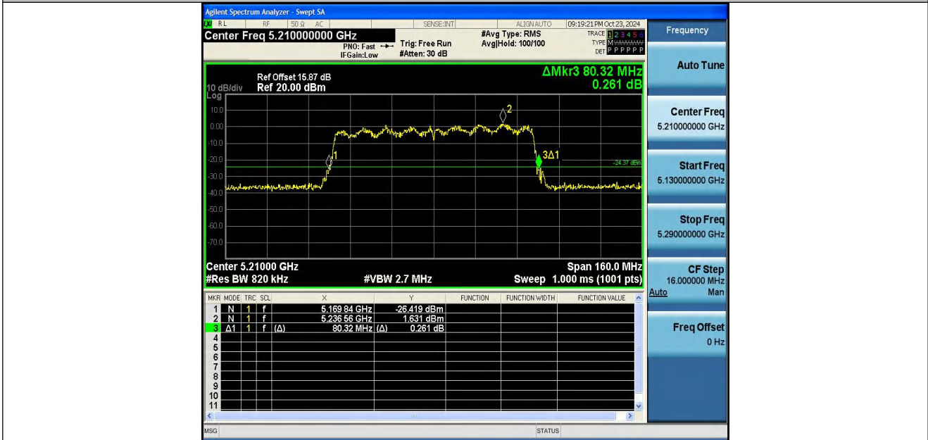
11AC80SISO-Ant2-5210
