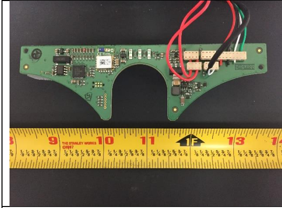
EUT Internal PCBA Top
