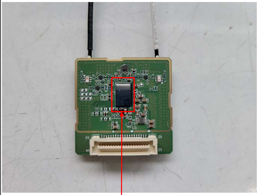
BT/WIFI Module
