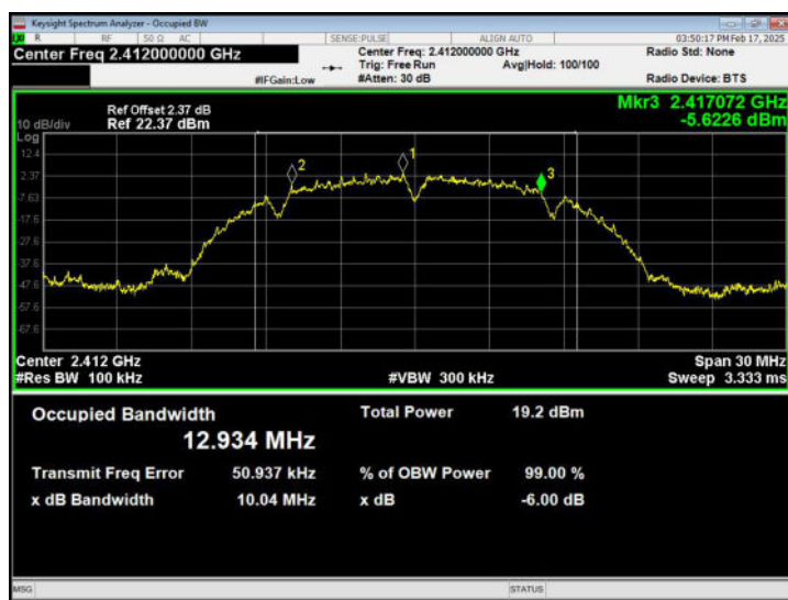
802.11b - CH01
