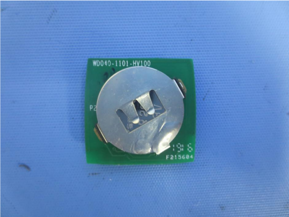
(3) EUT Photo
